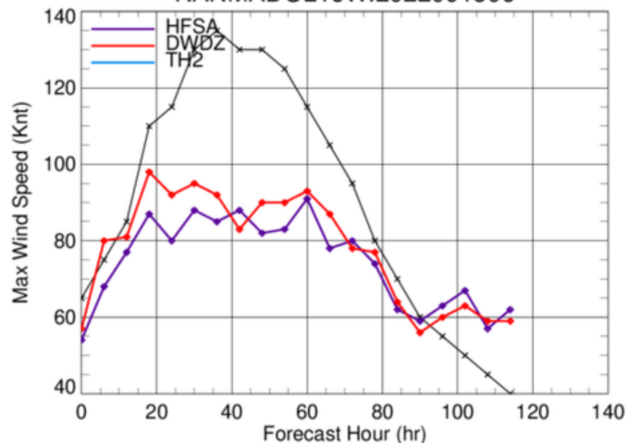
NANMADOL16W.2022091506
