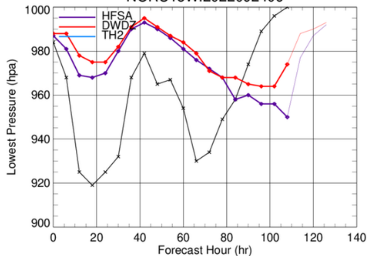
NORU18W.2022092406
