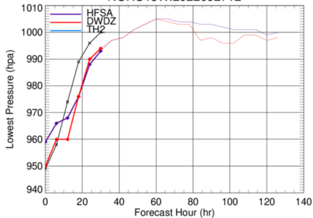
NORU18W.2022092712
