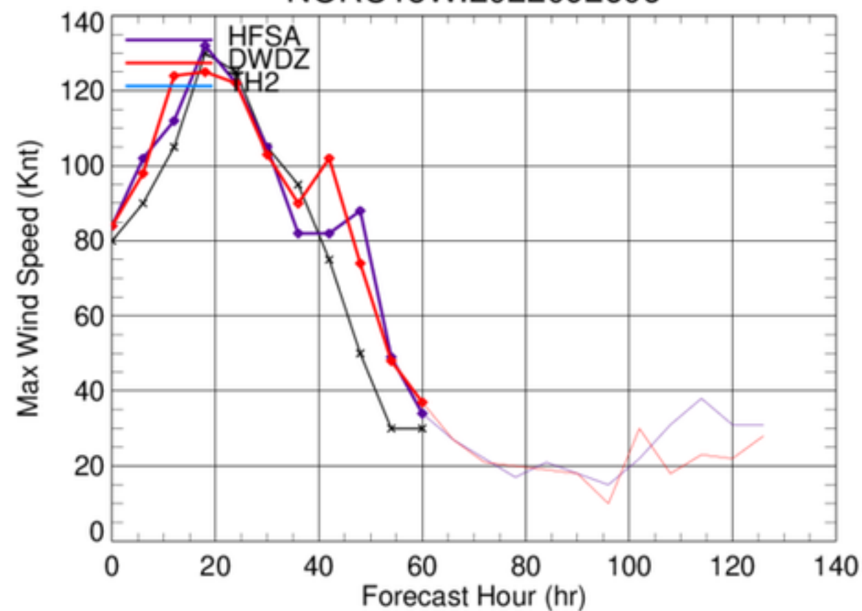
NORU18W.2022092606
