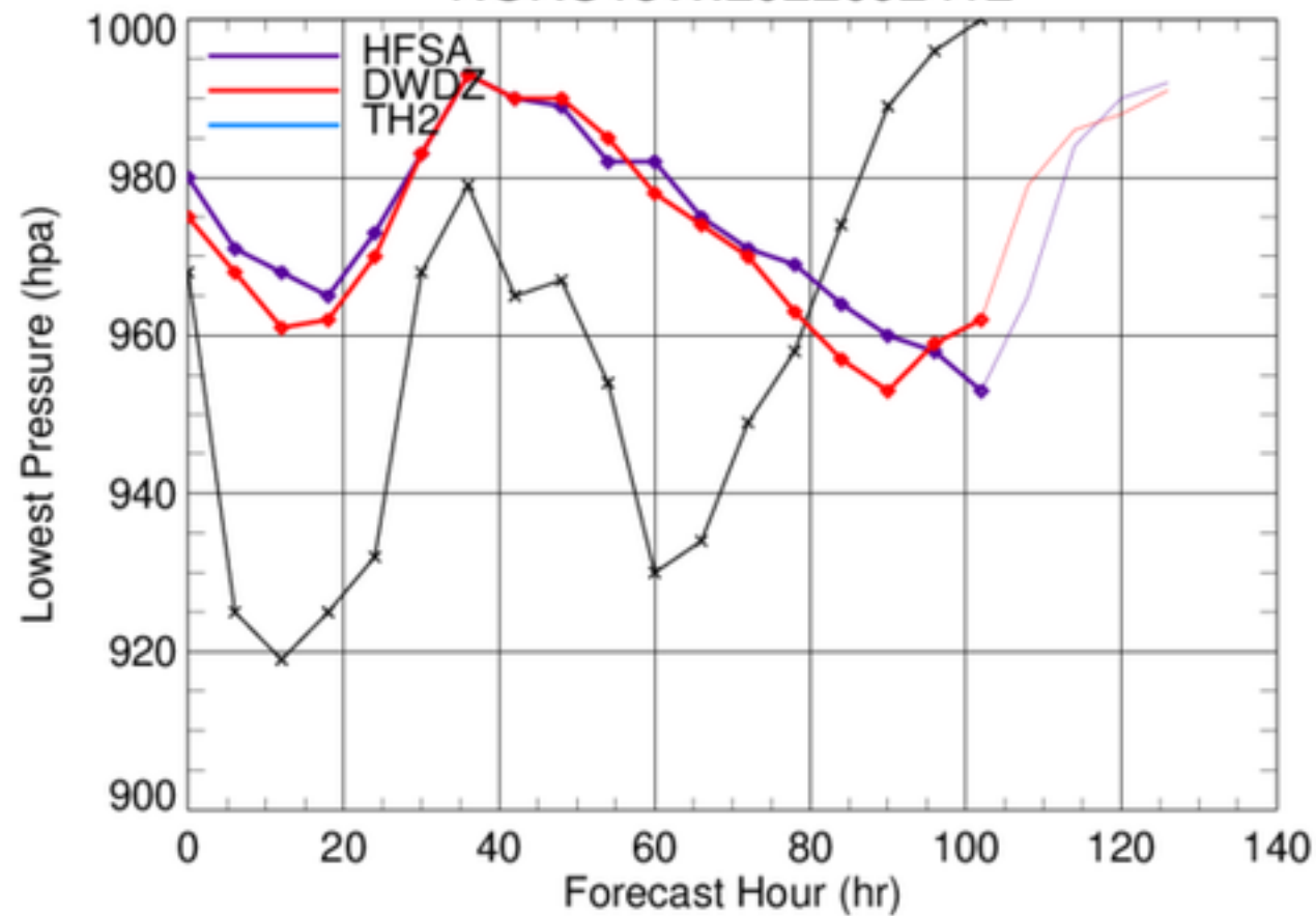
NORU18W.2022092412
