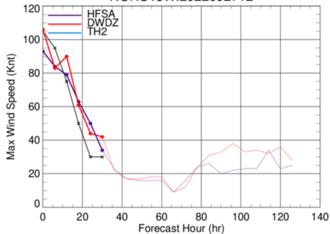
NORU18W.2022092712
