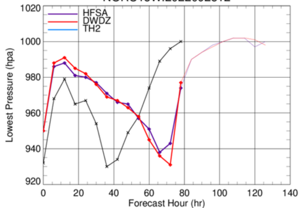
NORU18W.2022092512
