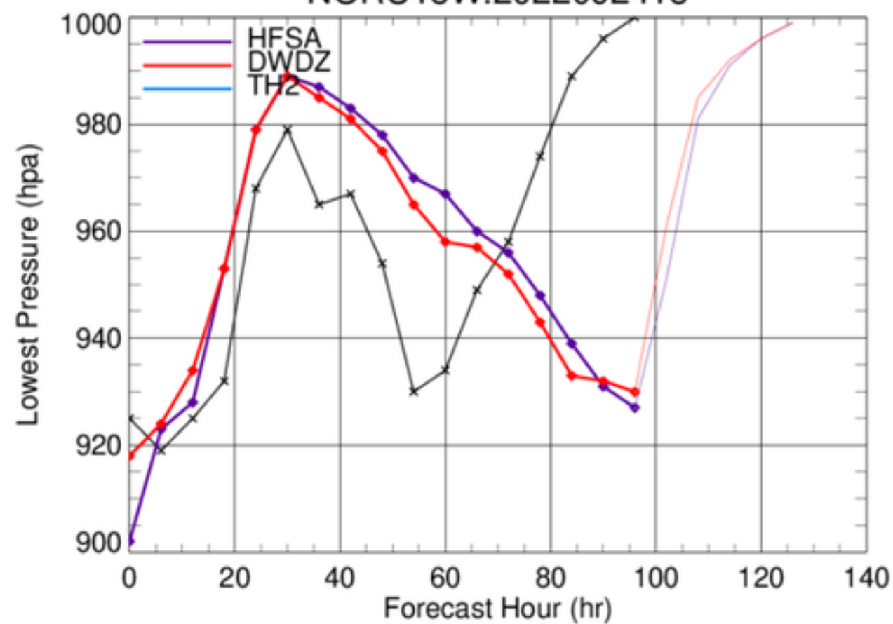
NORU18W.2022092418
