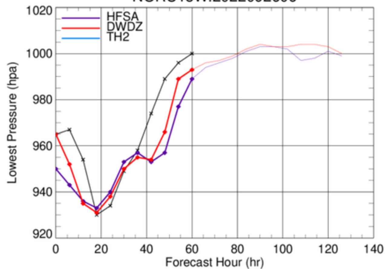
NORU18W.2022092606
