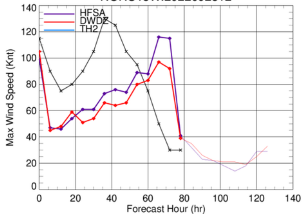
NORU18W.2022092512
