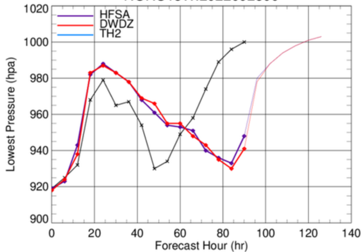
NORU18W.2022092500
