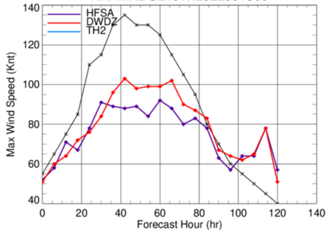
NANMADOL16W.2022091500
