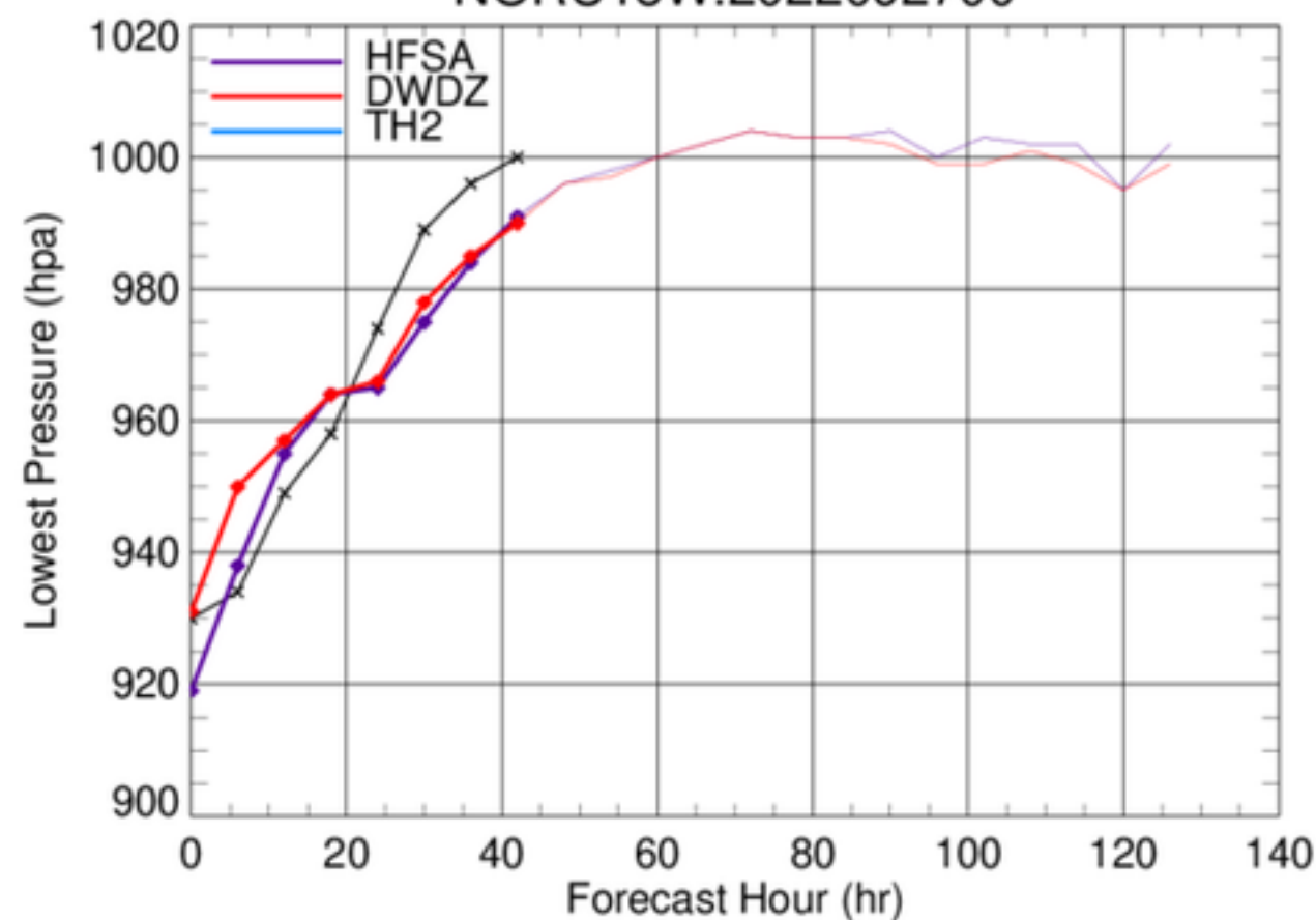
NORU18W.2022092700
