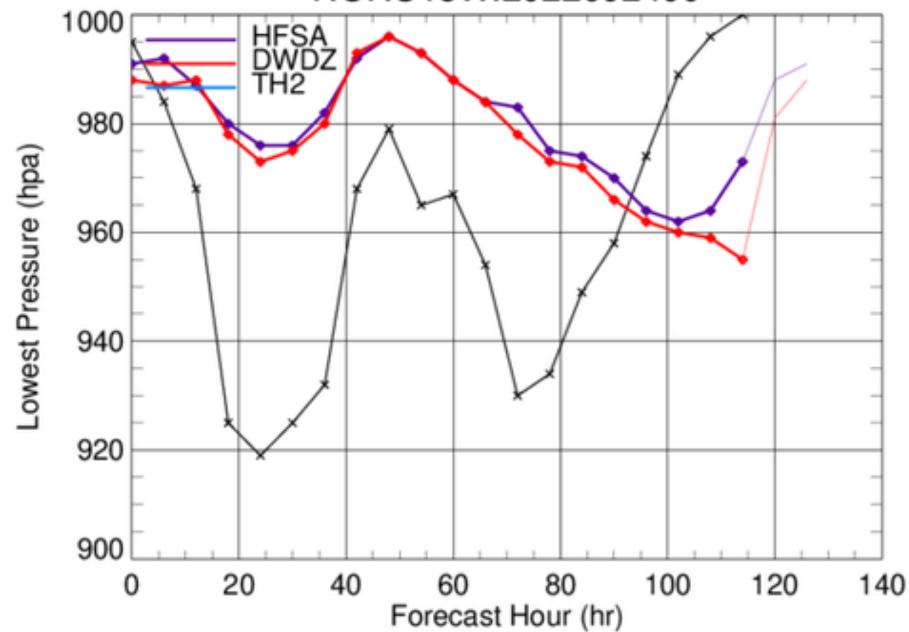
NORU18W.2022092400
