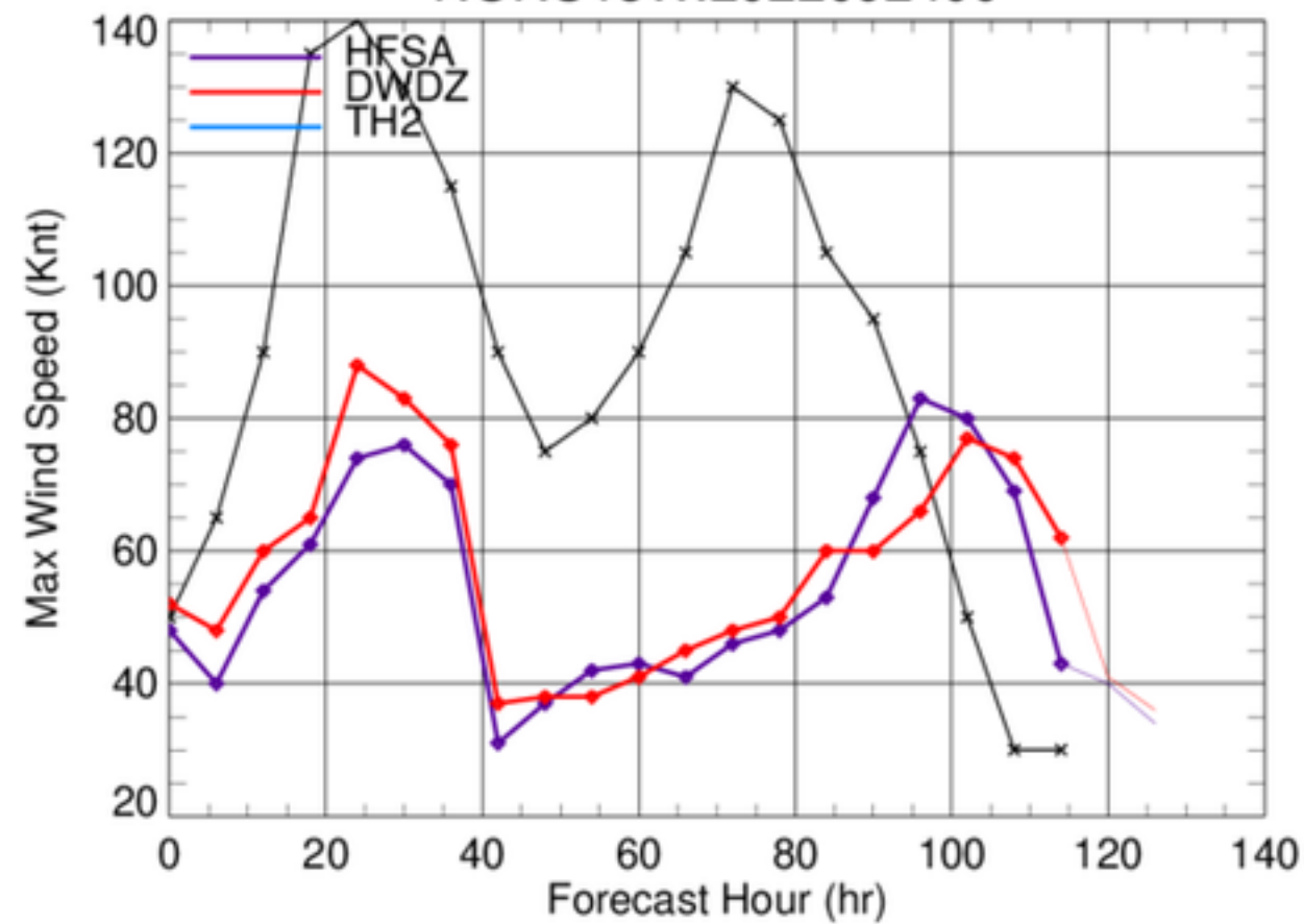
NORU18W.2022092400
