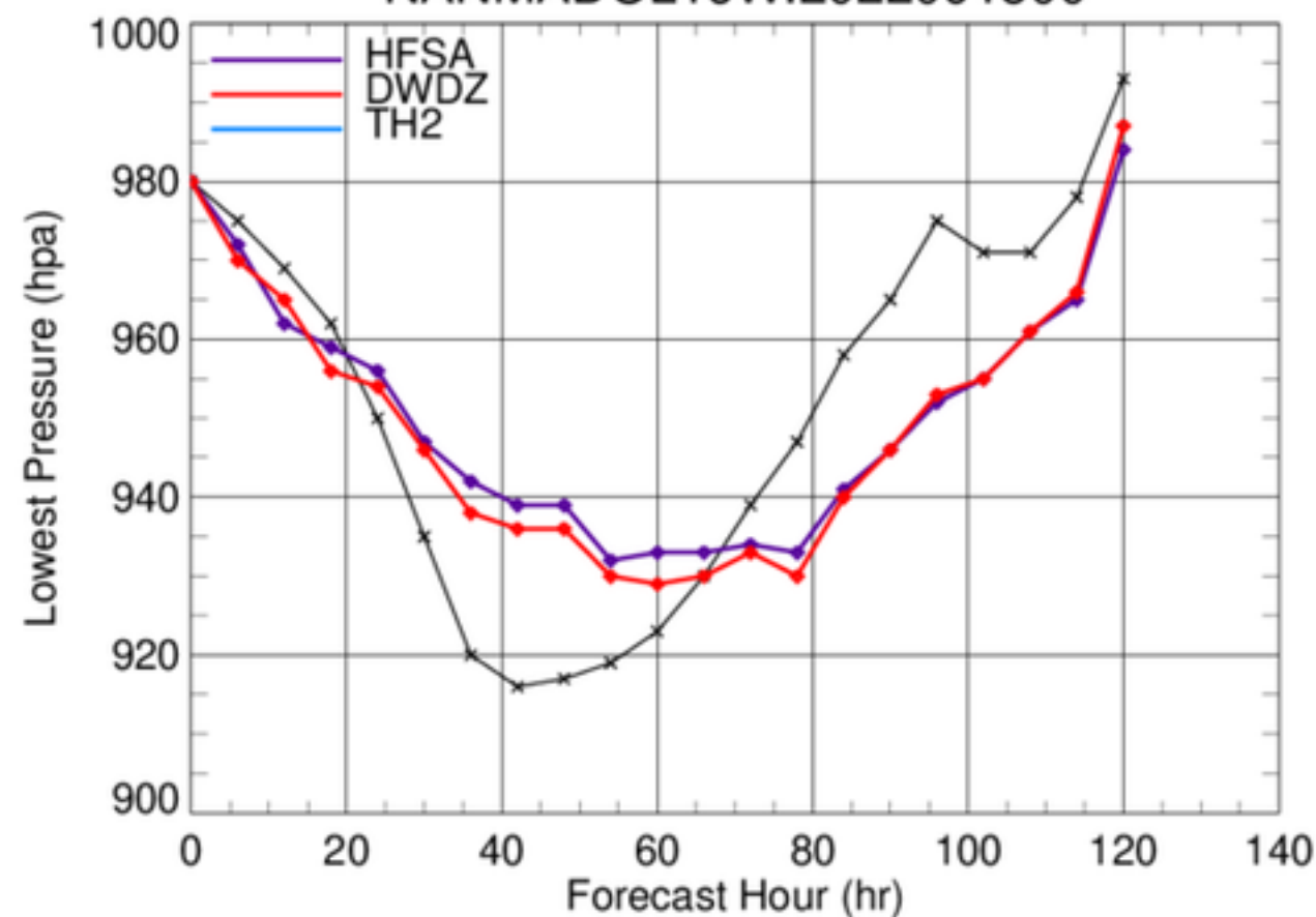
NANMADOL16W.2022091500
