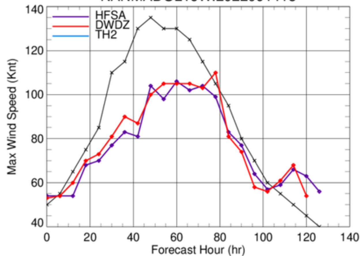
NANMADOL16W.2022091418
