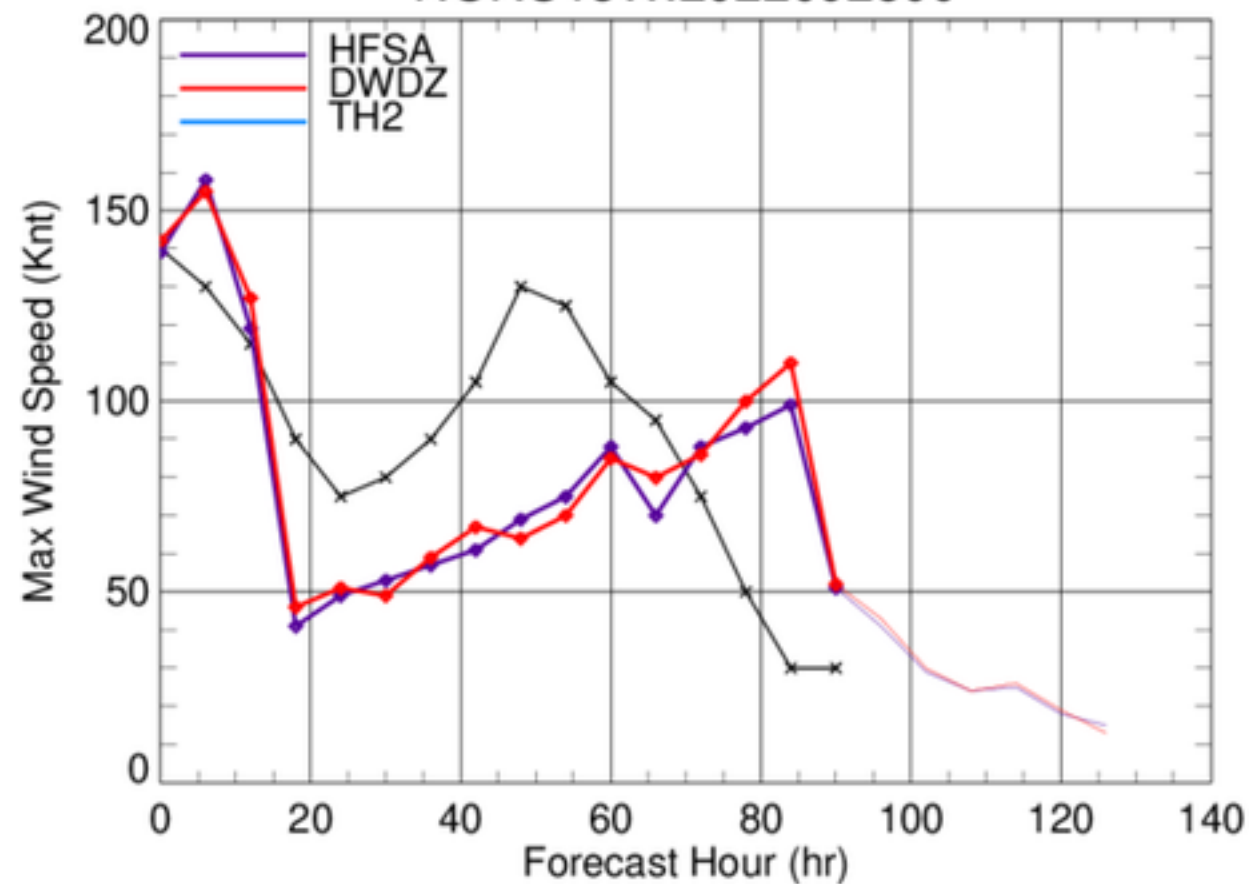
NORU18W.2022092500
