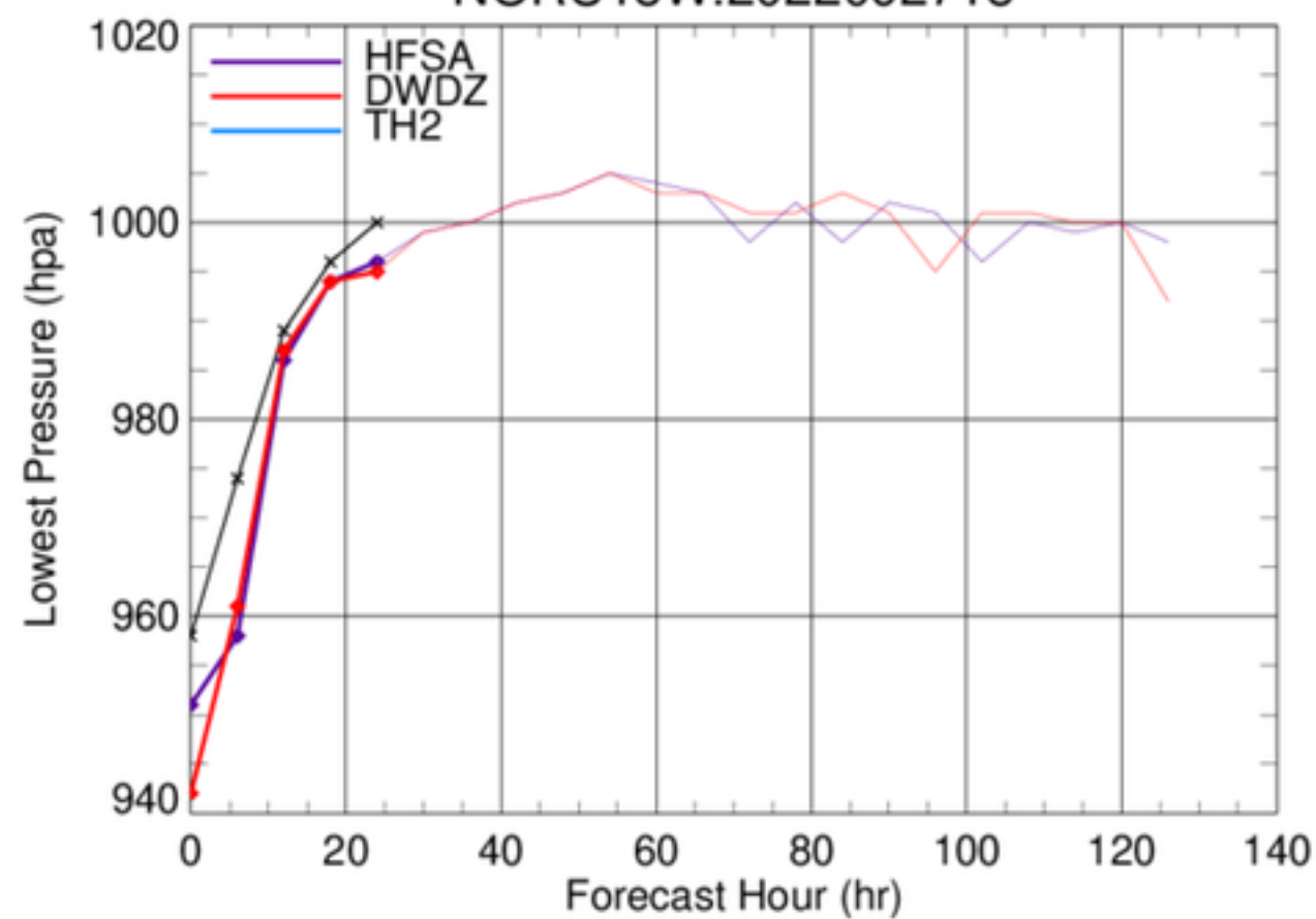
NORU18W.2022092718
