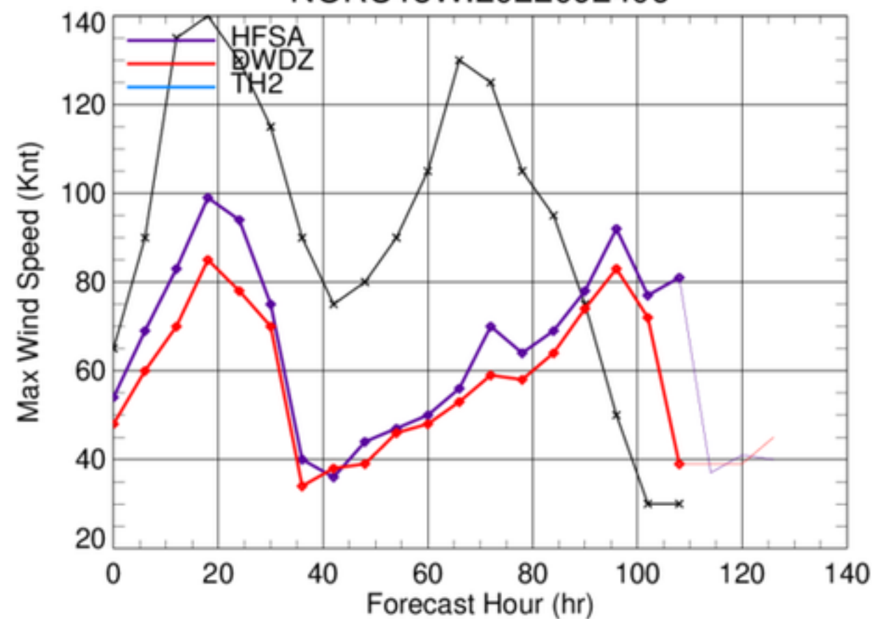
NORU18W.2022092406
