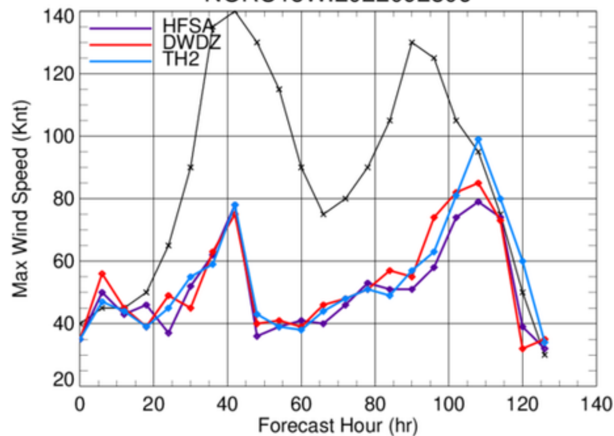
NORU18W.2022092306
