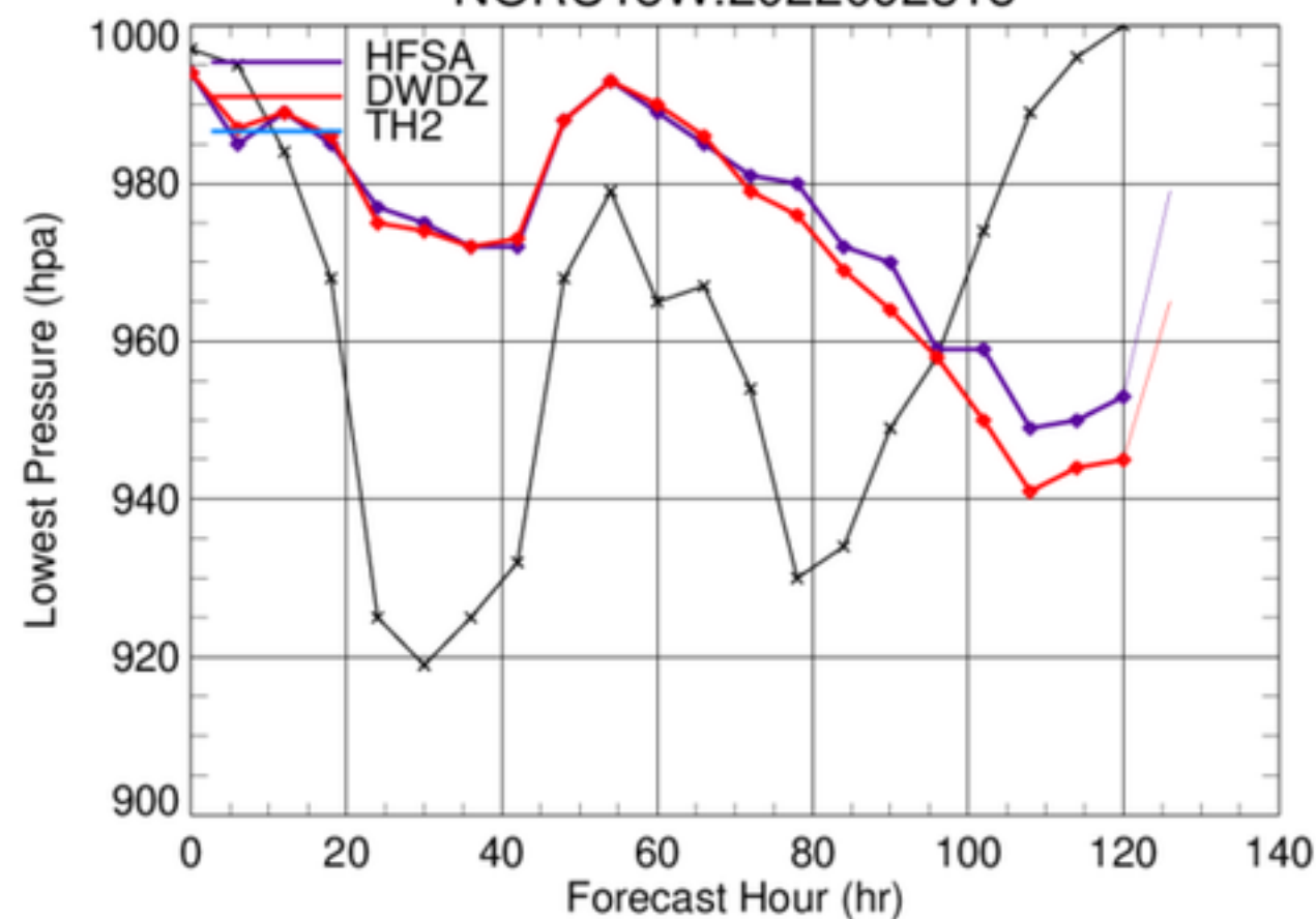
NORU18W.2022092318
