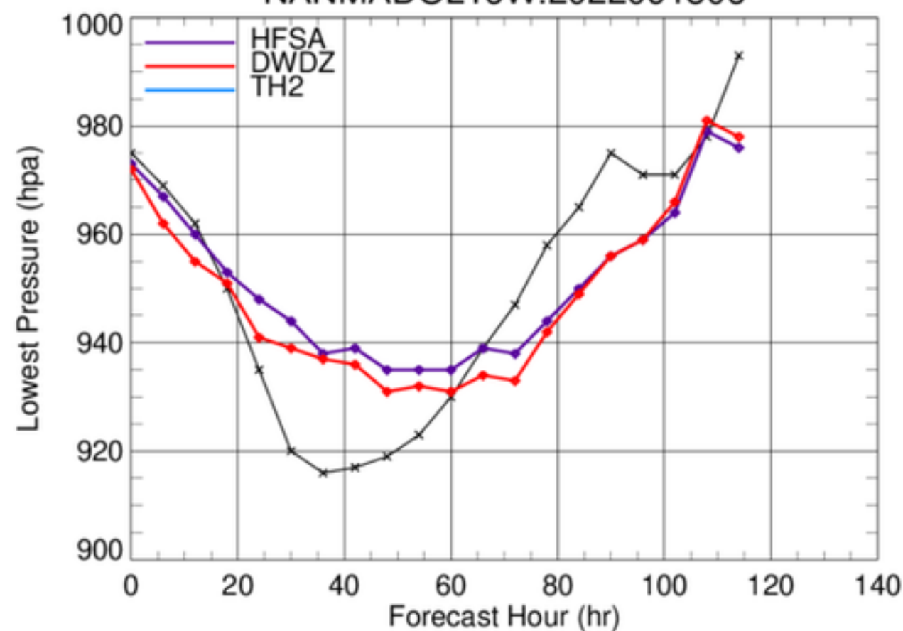
NANMADOL16W.2022091506
