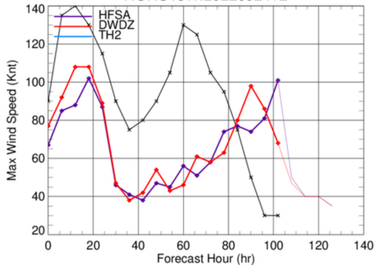
NORU18W.2022092412
