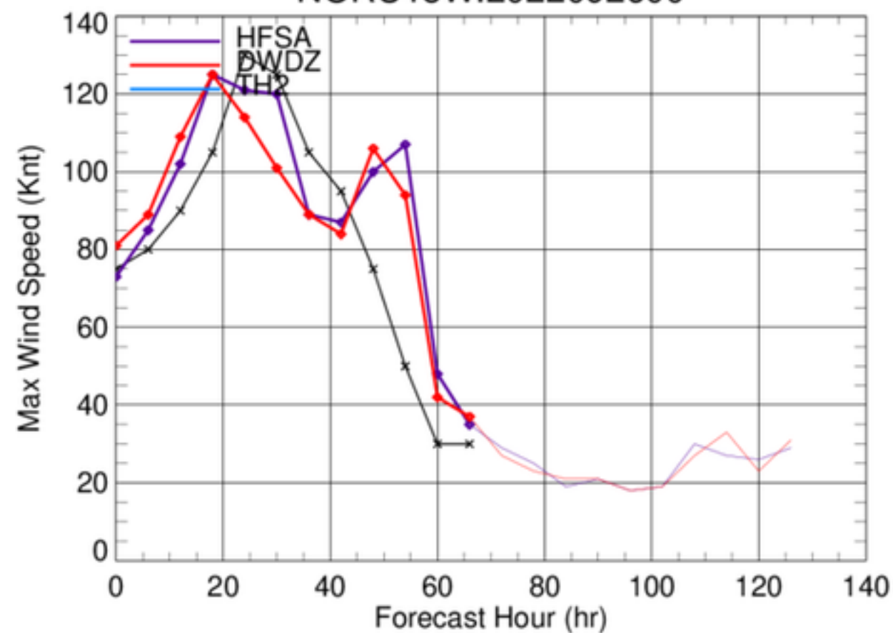
NORU18W.2022092600
