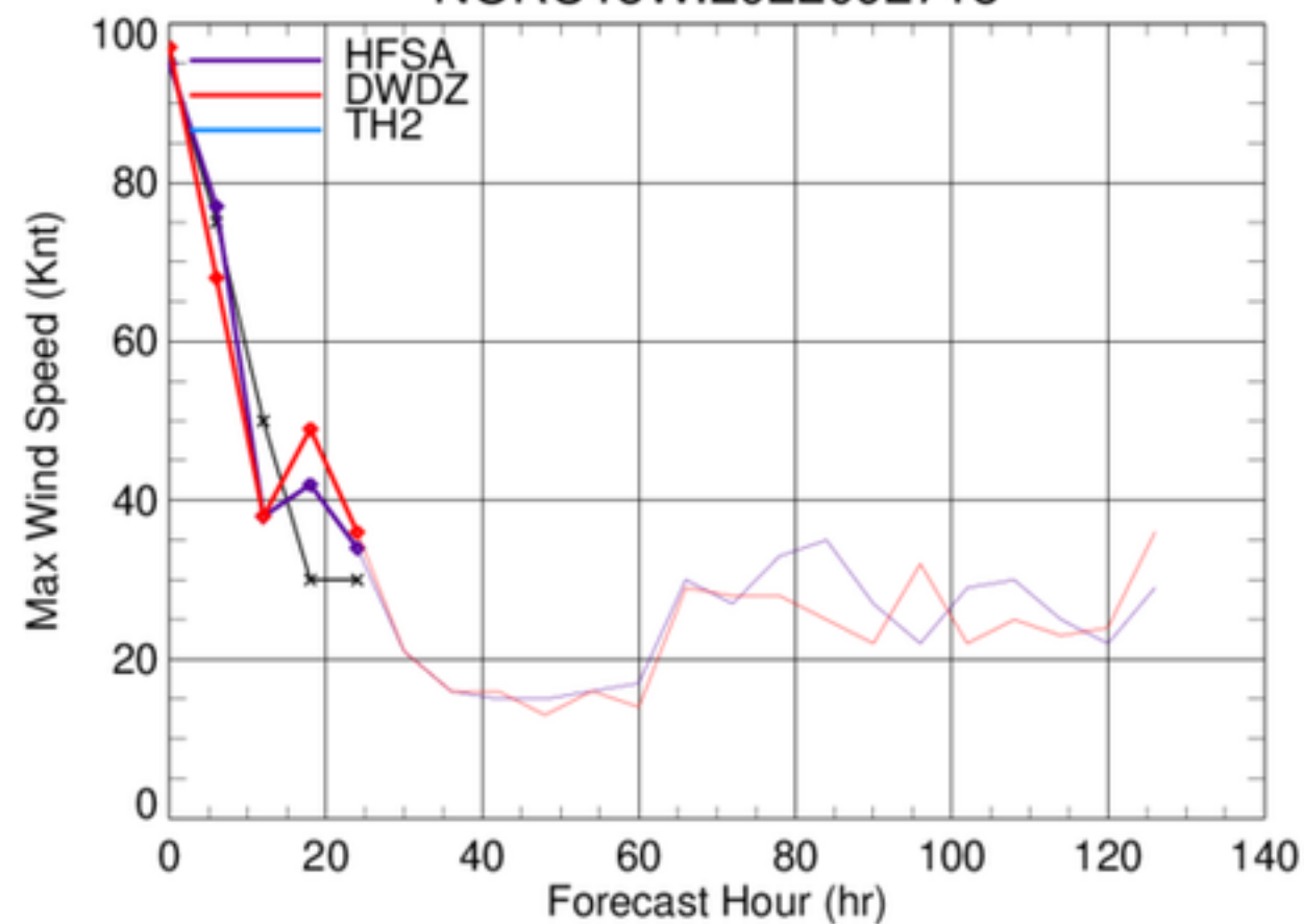
NORU18W.2022092718
