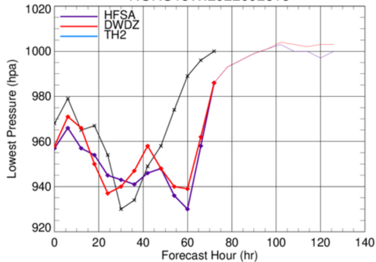
NORU18W.2022092518
