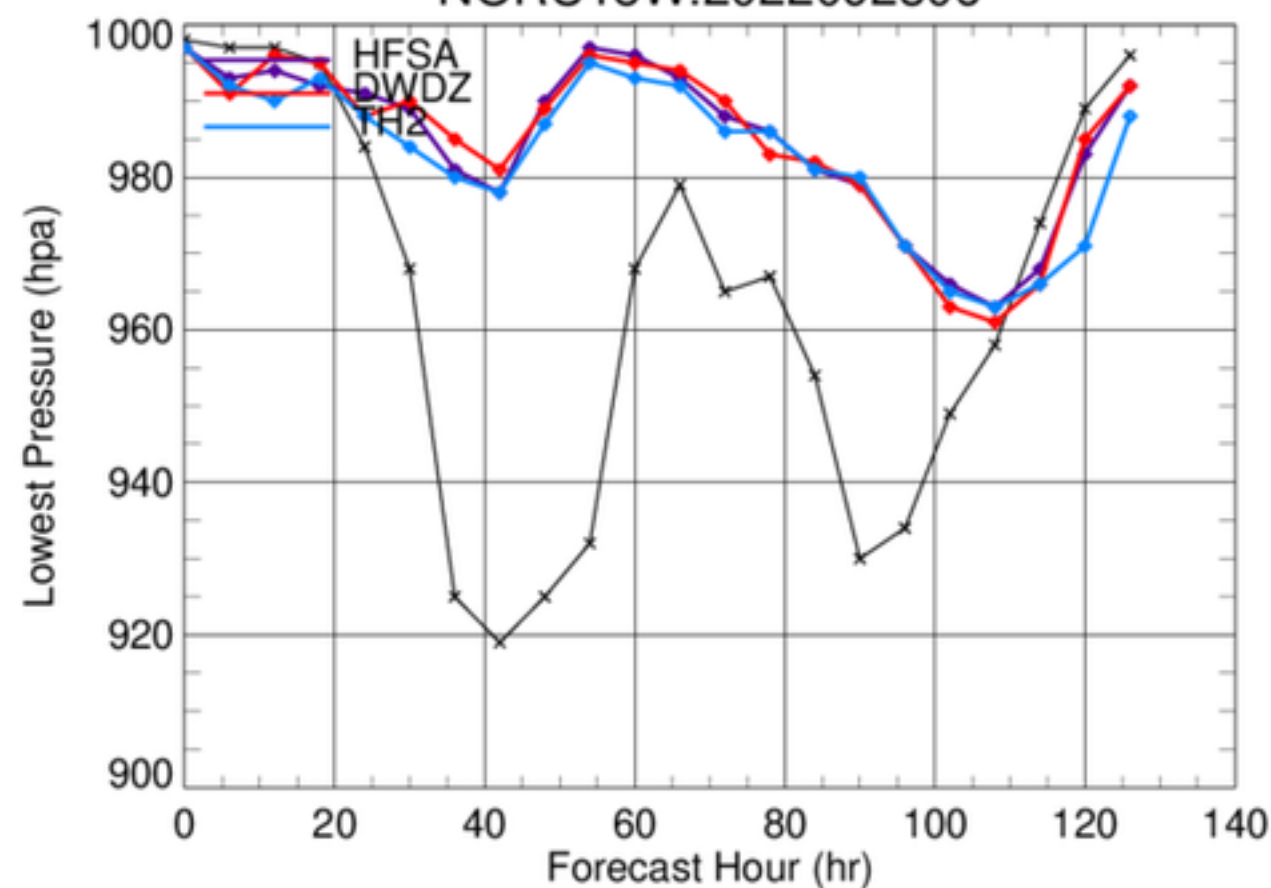
NORU18W.2022092306
