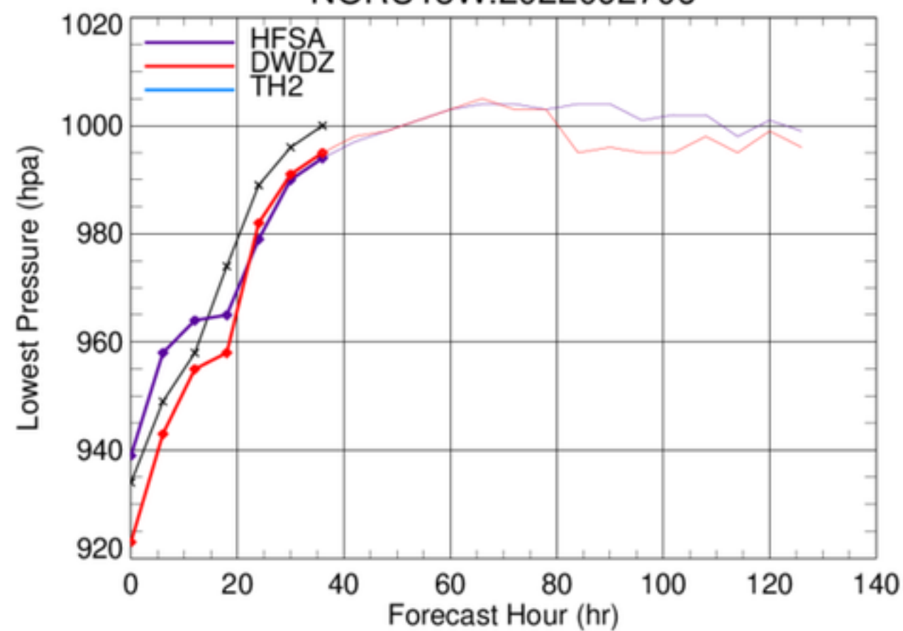
NORU18W.2022092706
