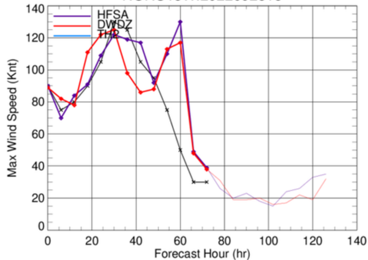
NORU18W.2022092518
