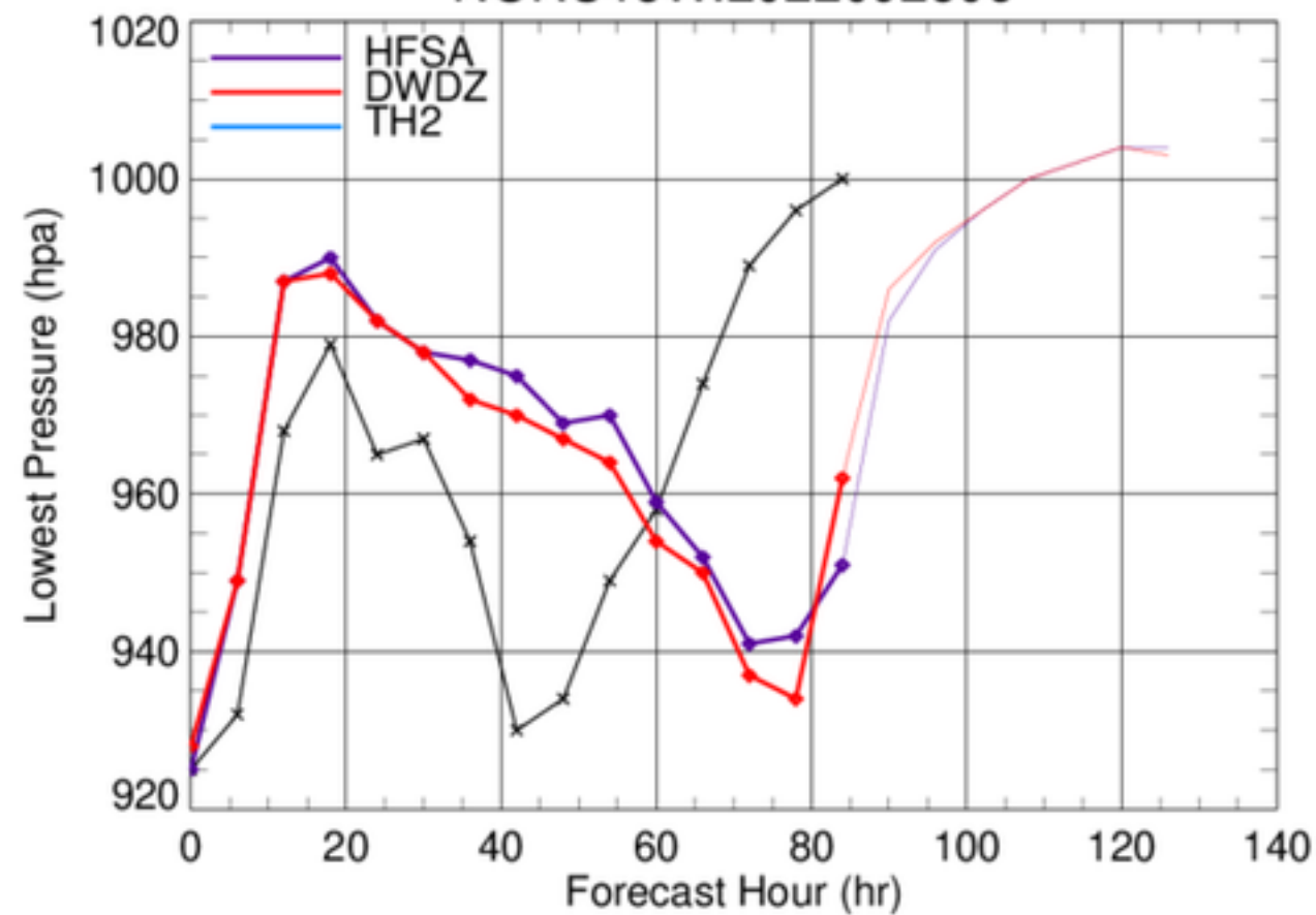
NORU18W.2022092506
