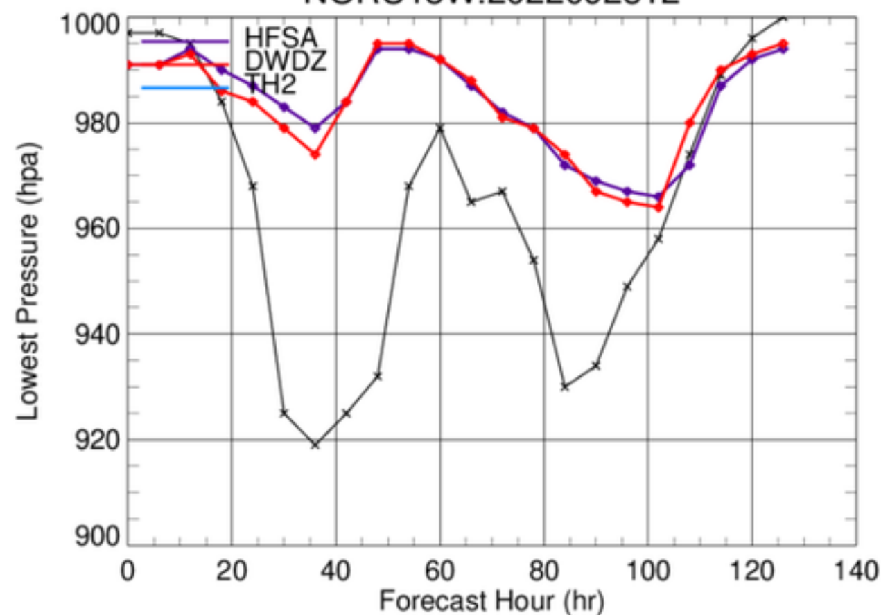
NORU18W.2022092312
