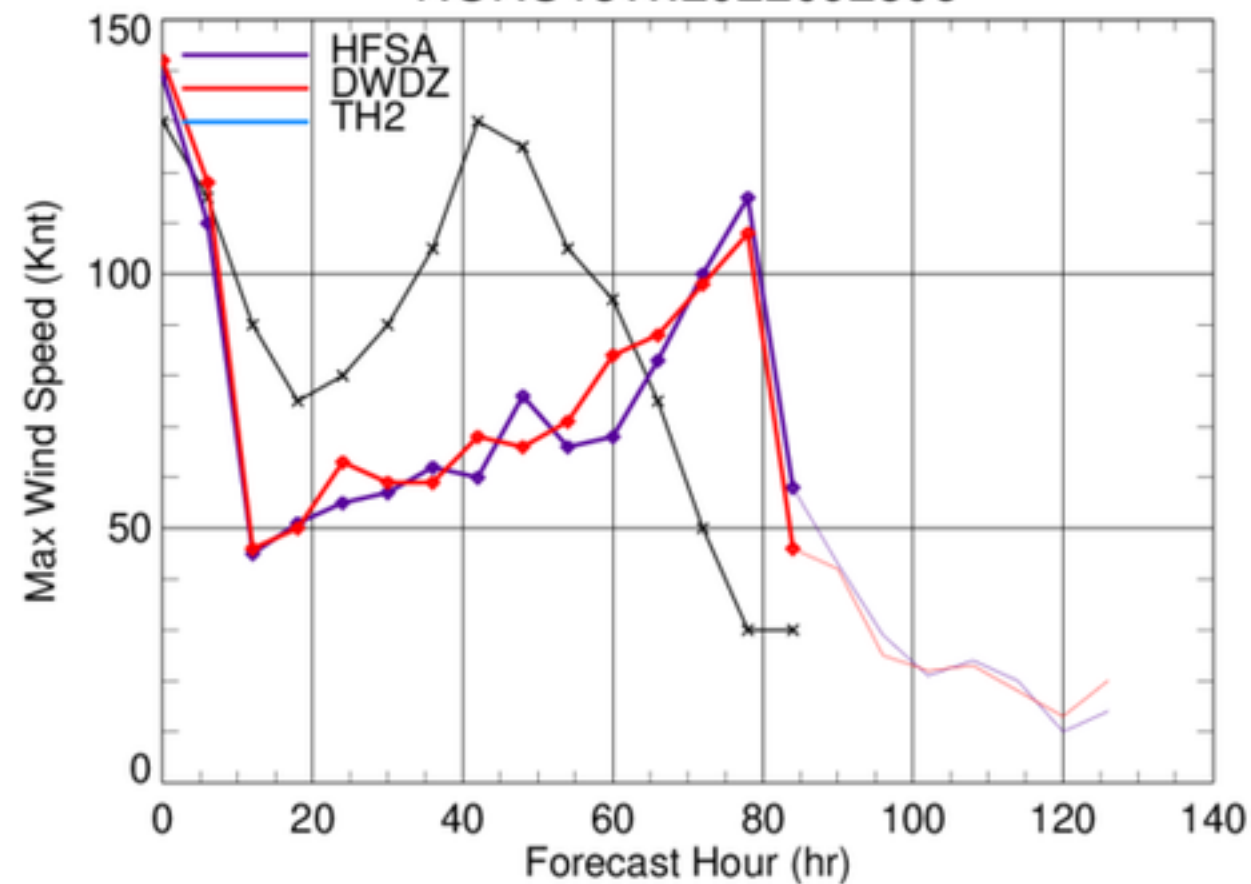
NORU18W.2022092506
