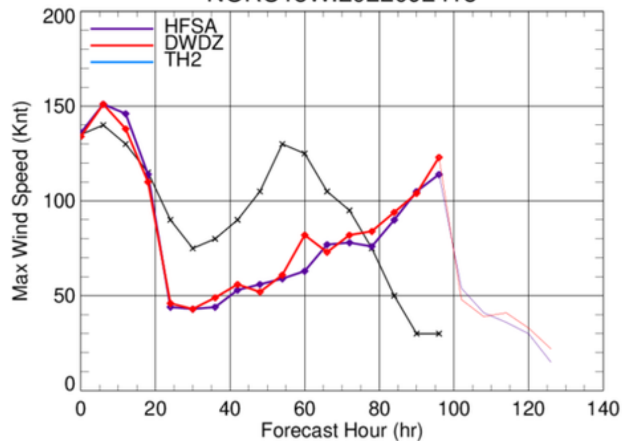
NORU18W.2022092418
