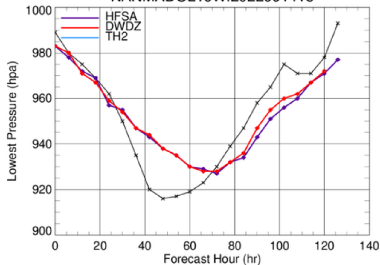
NANMADOL16W.2022091418
