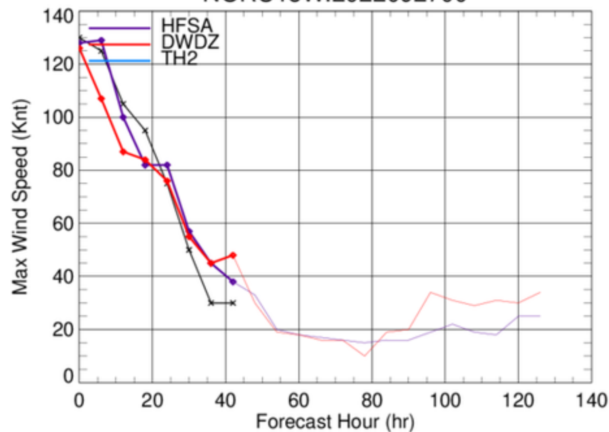
NORU18W.2022092700
