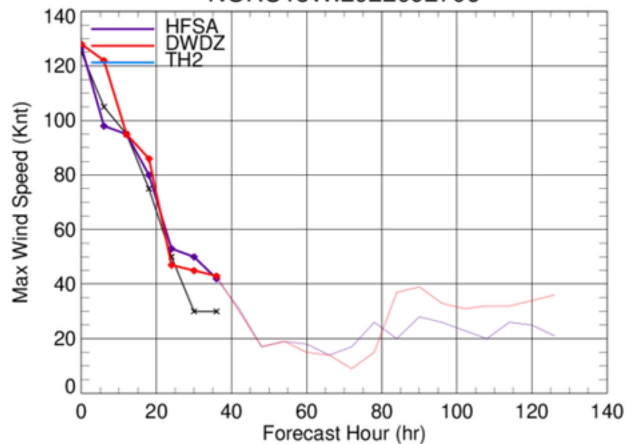
NORU18W.2022092706
