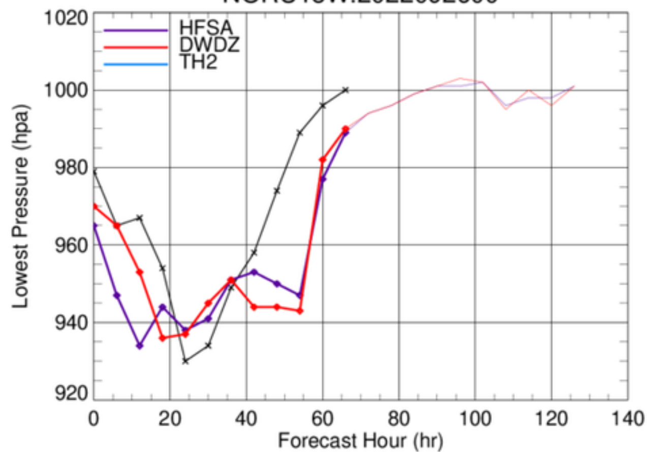
NORU18W.2022092600
