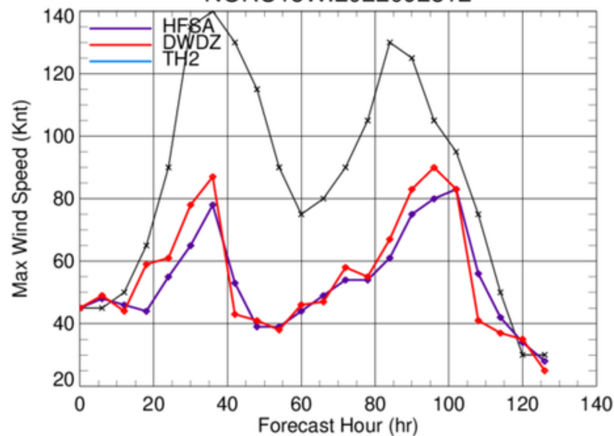
NORU18W.2022092312
