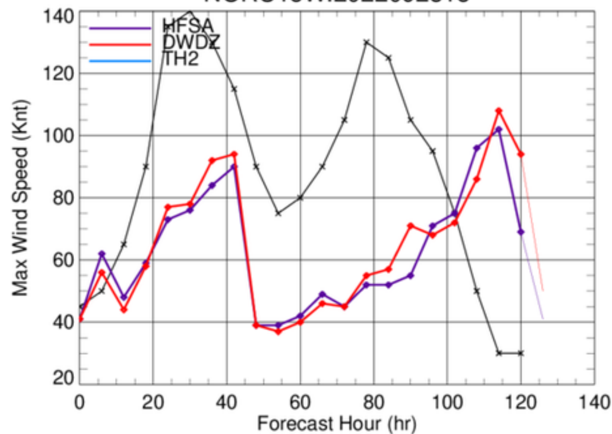
NORU18W.2022092318
