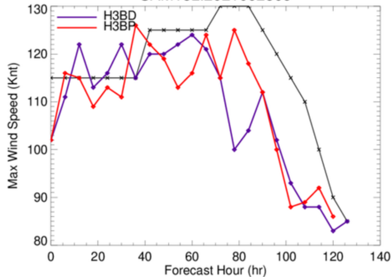
SAM18L.2021092806
