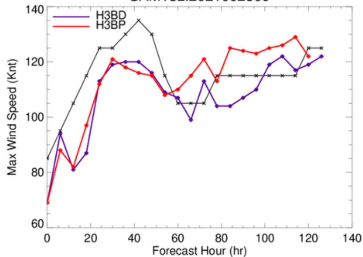
SAM18L.2021092500
