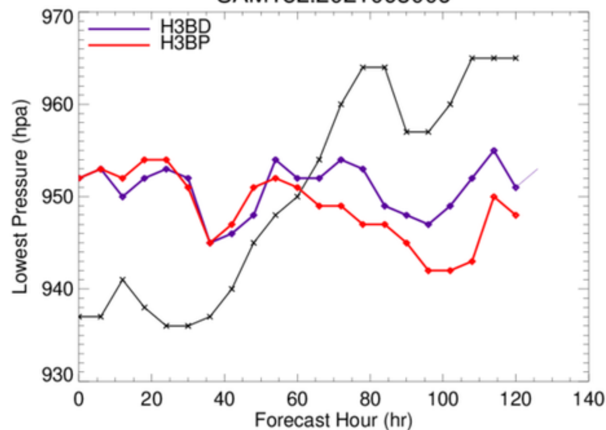
SAM18L.2021093006
