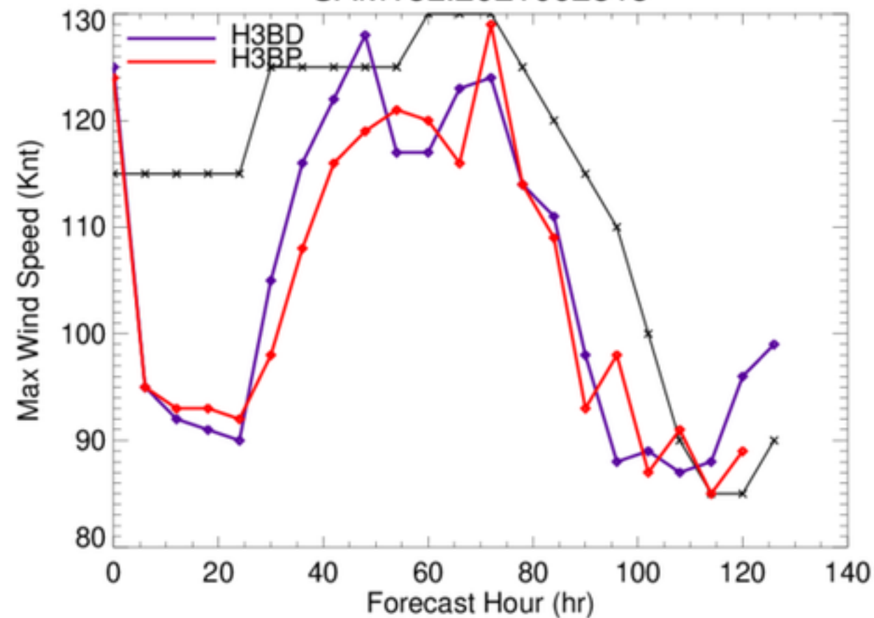
SAM18L.2021092818
