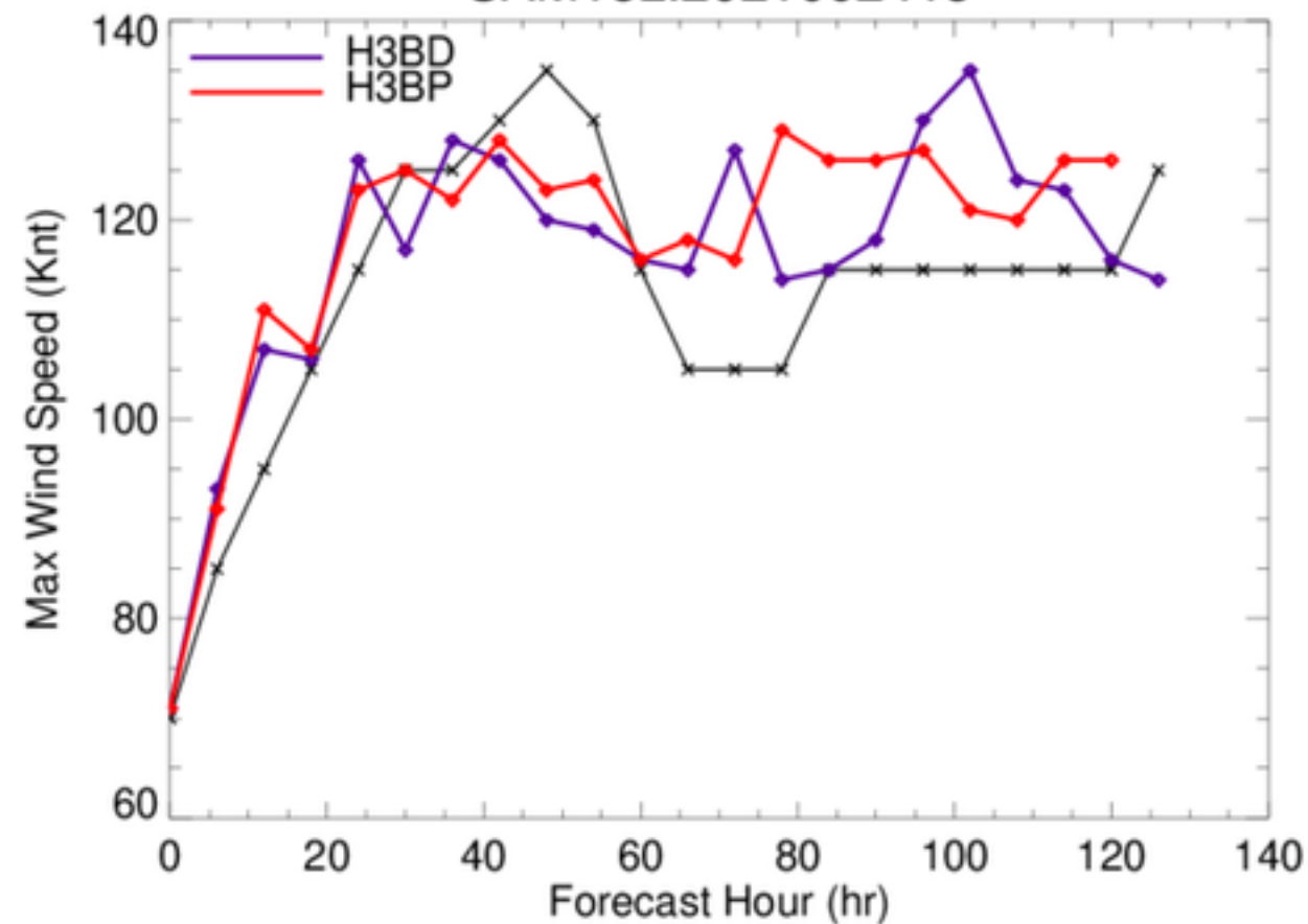
SAM18L.2021092418
