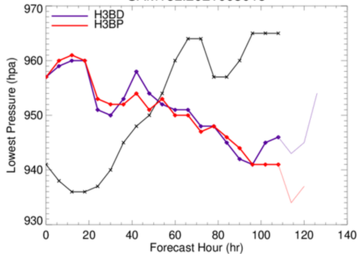
SAM18L.2021093018
