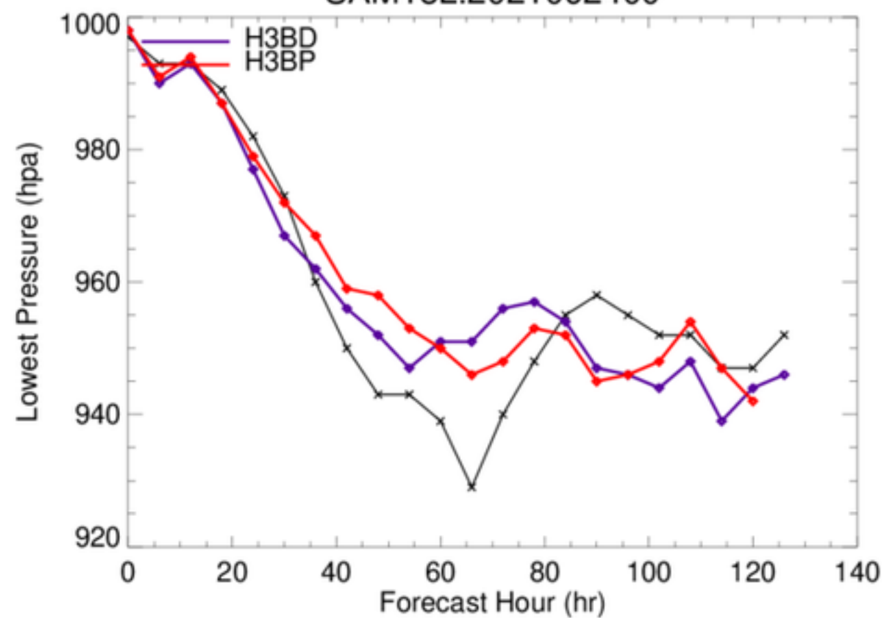
SAM18L.2021092400
