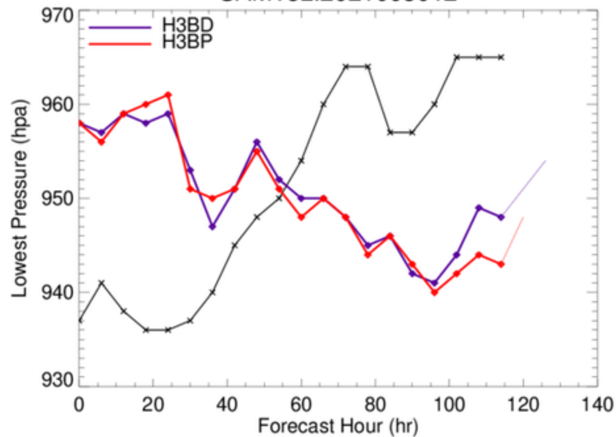
SAM18L.2021093012
