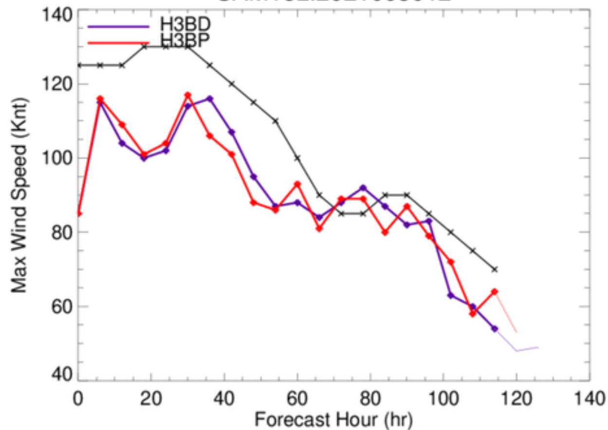
SAM18L.2021093012
