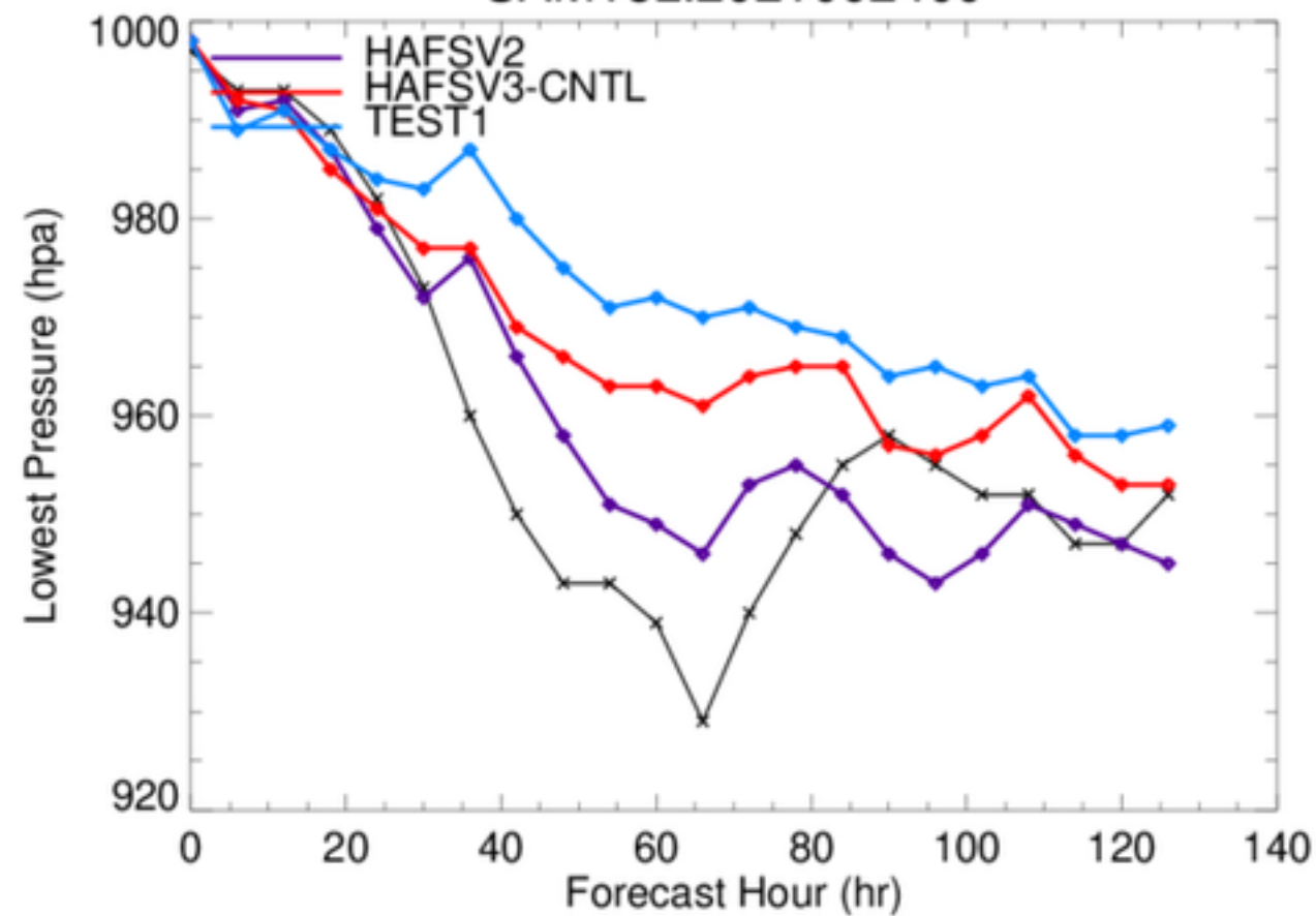
SAM18L.2021092400
