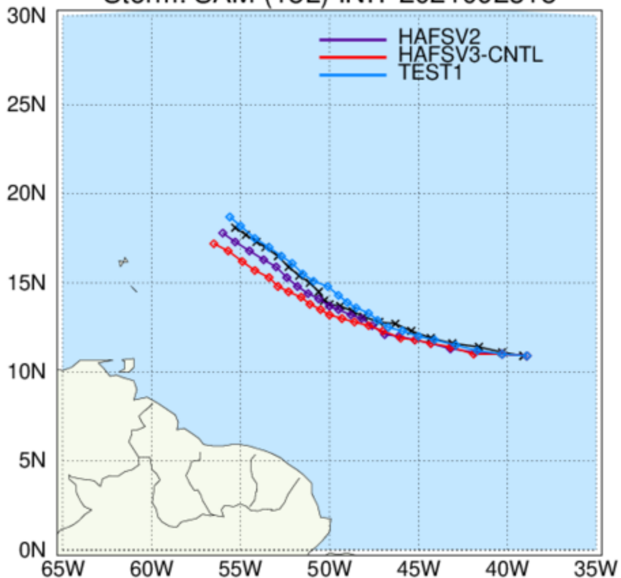
HWRF: TC Tracks Storm: SAM (18L) INIT 2021092318
