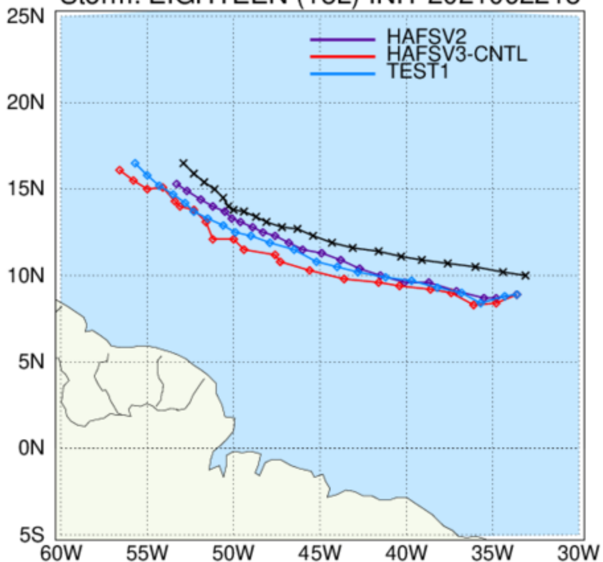
HWRF: TC Tracks Storm: EIGHTEEN (18L) INIT 2021092218
