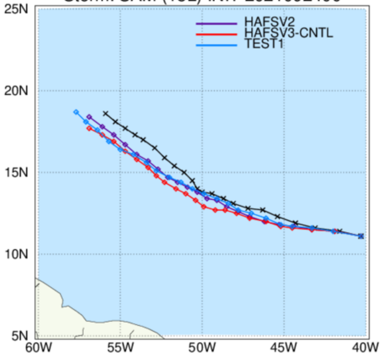
HWRF: TC Tracks Storm: SAM (18L) INIT 2021092400
