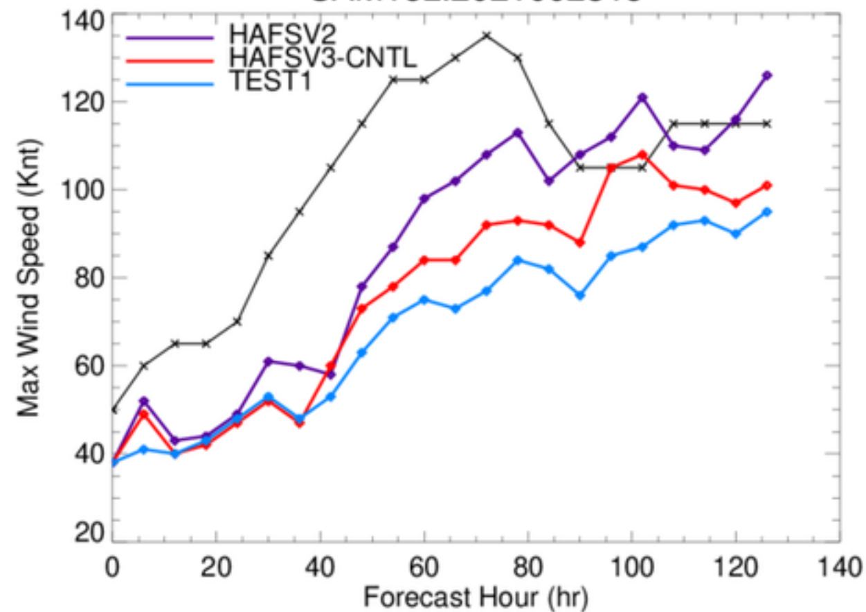
SAM18L.2021092318
