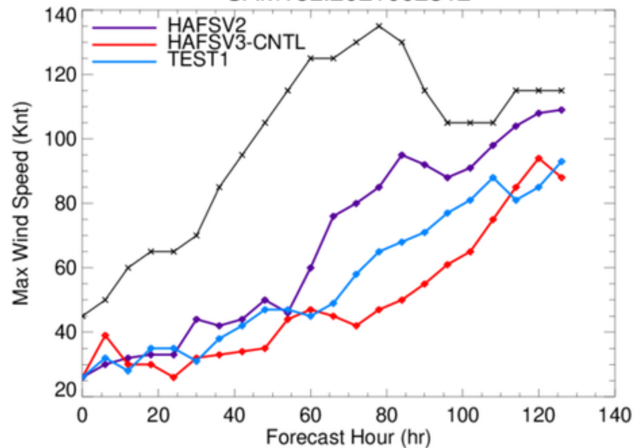
SAM18L.2021092312
