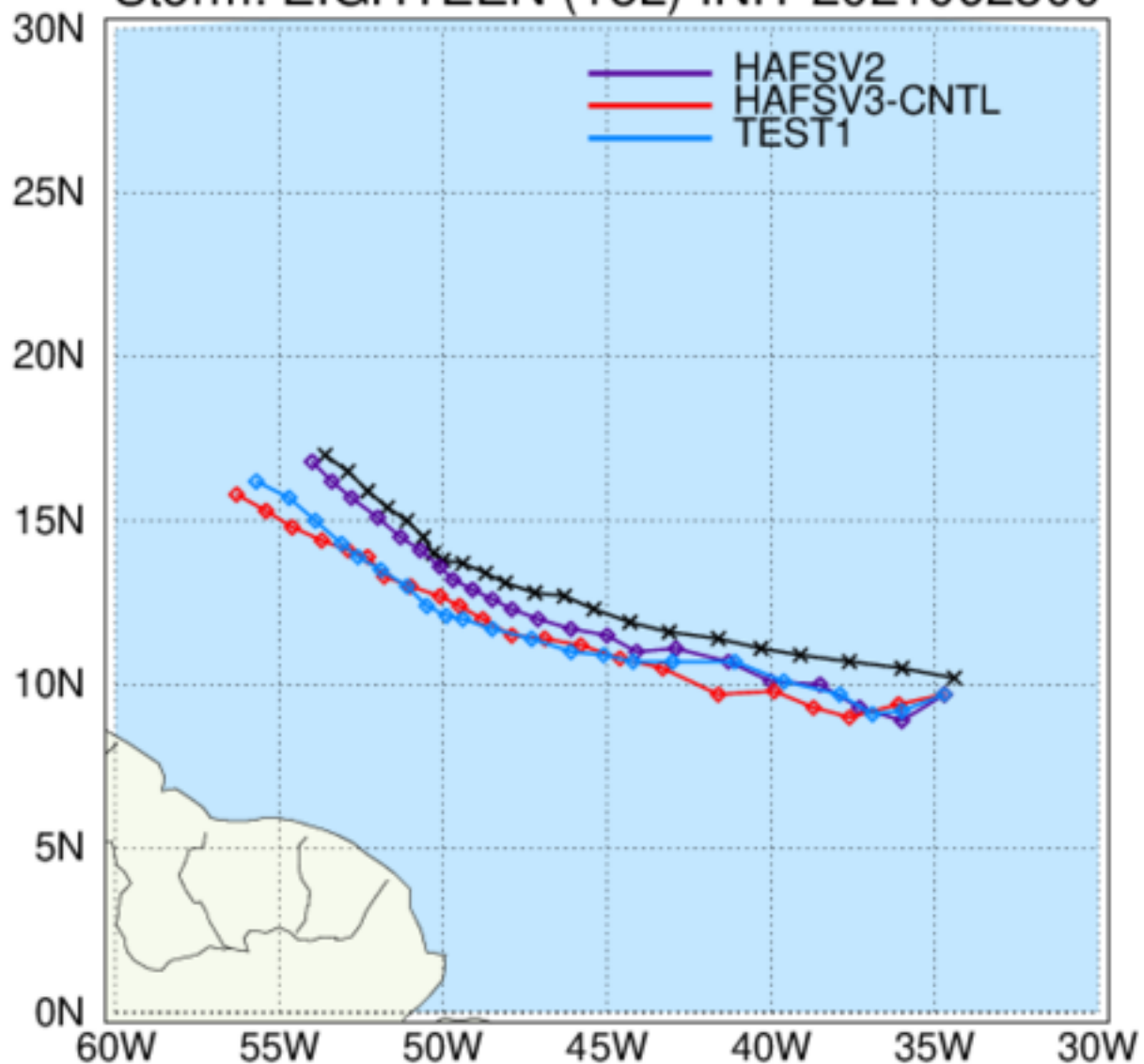
HWRF: TC Tracks Storm: EIGHTEEN (18L) INIT 2021092300
