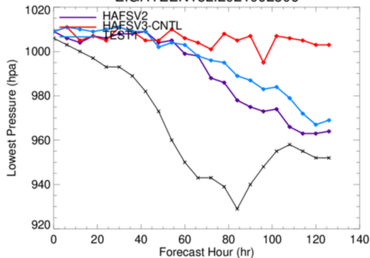
EIGHTEEN18L.2021092306
