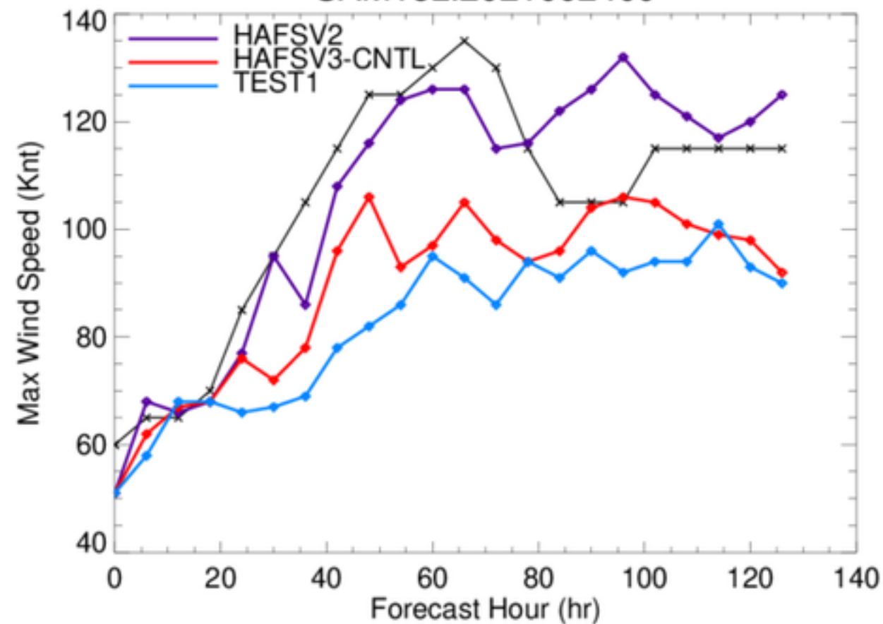
SAM18L.2021092400
