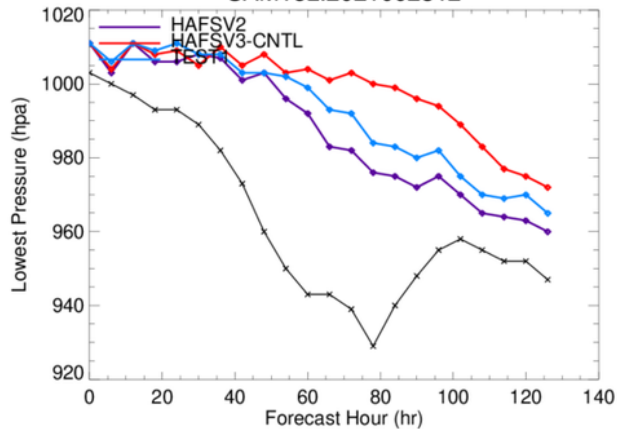
SAM18L.2021092312
