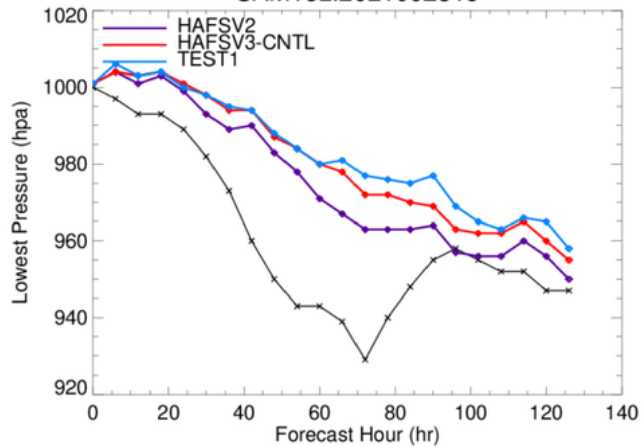
SAM18L.2021092318
