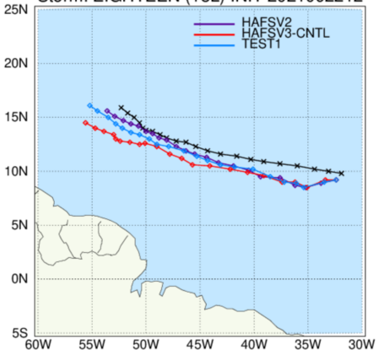
HWRF: TC Tracks Storm: EIGHTEEN (18L) INIT 2021092212
