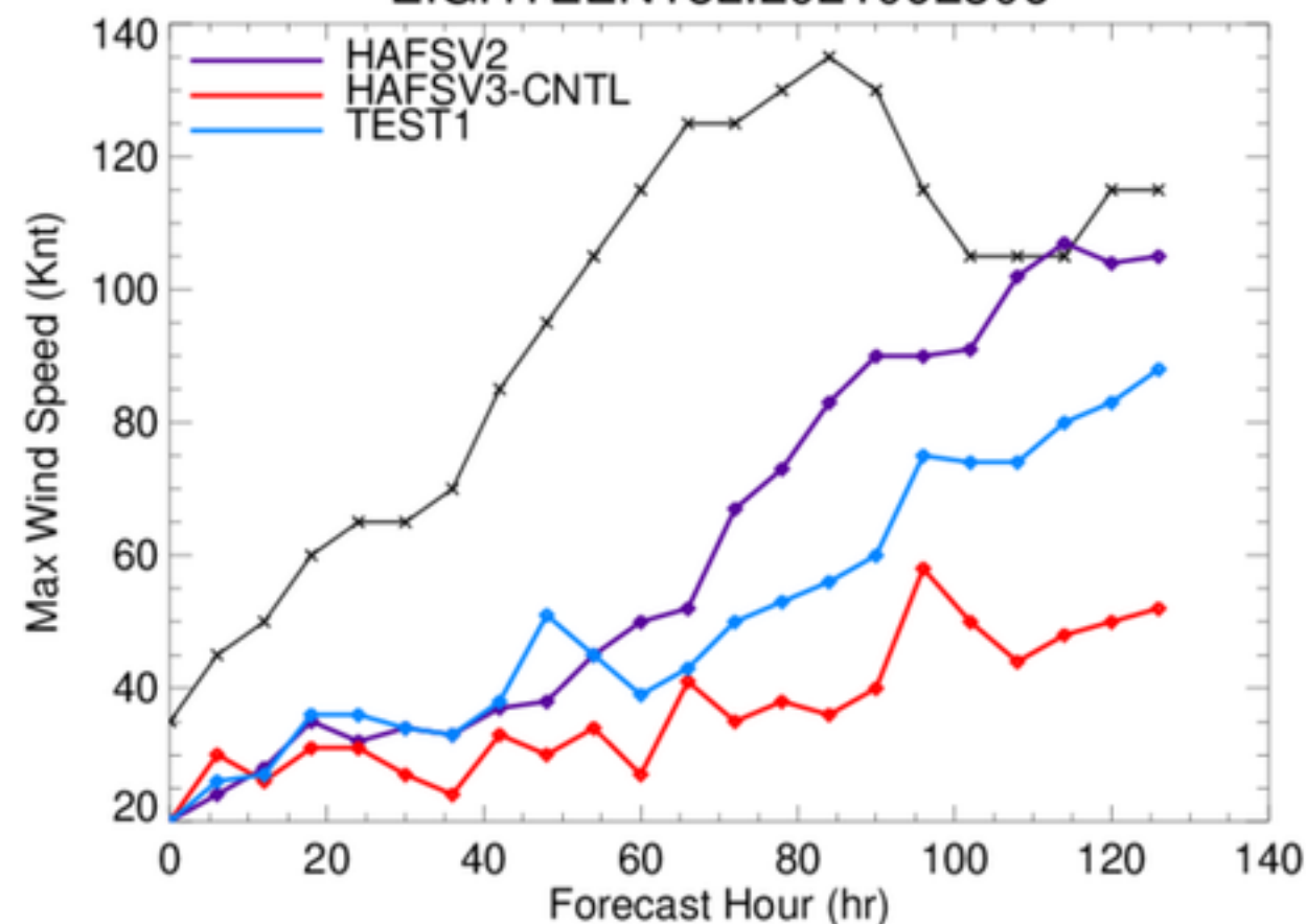
EIGHTEEN18L.2021092306
