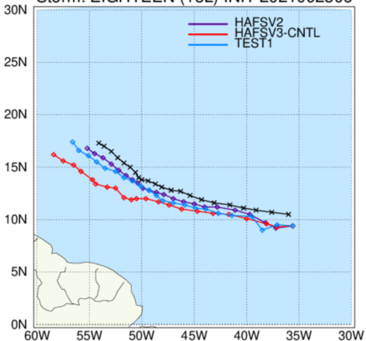
HWRF: TC Tracks Storm: EIGHTEEN (18L) INIT 2021092306
