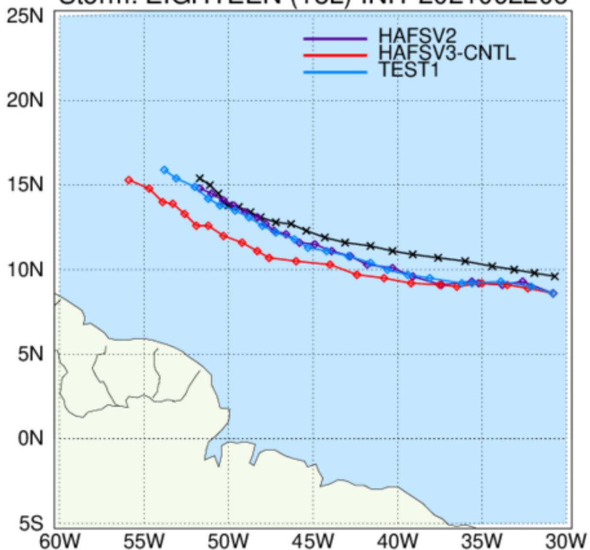
HWRF: TC Tracks Storm: EIGHTEEN (18L) INIT 2021092206
