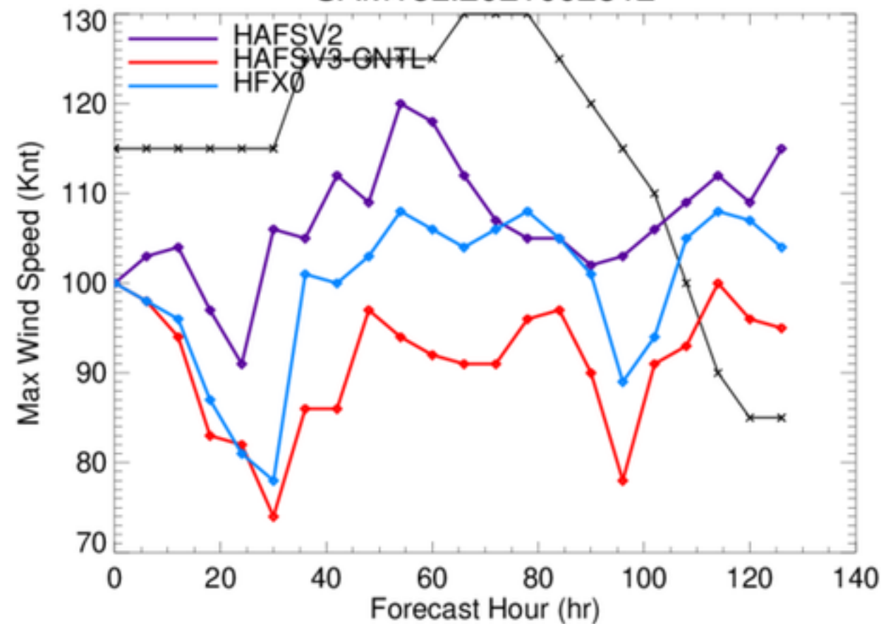
SAM18L.2021092812
