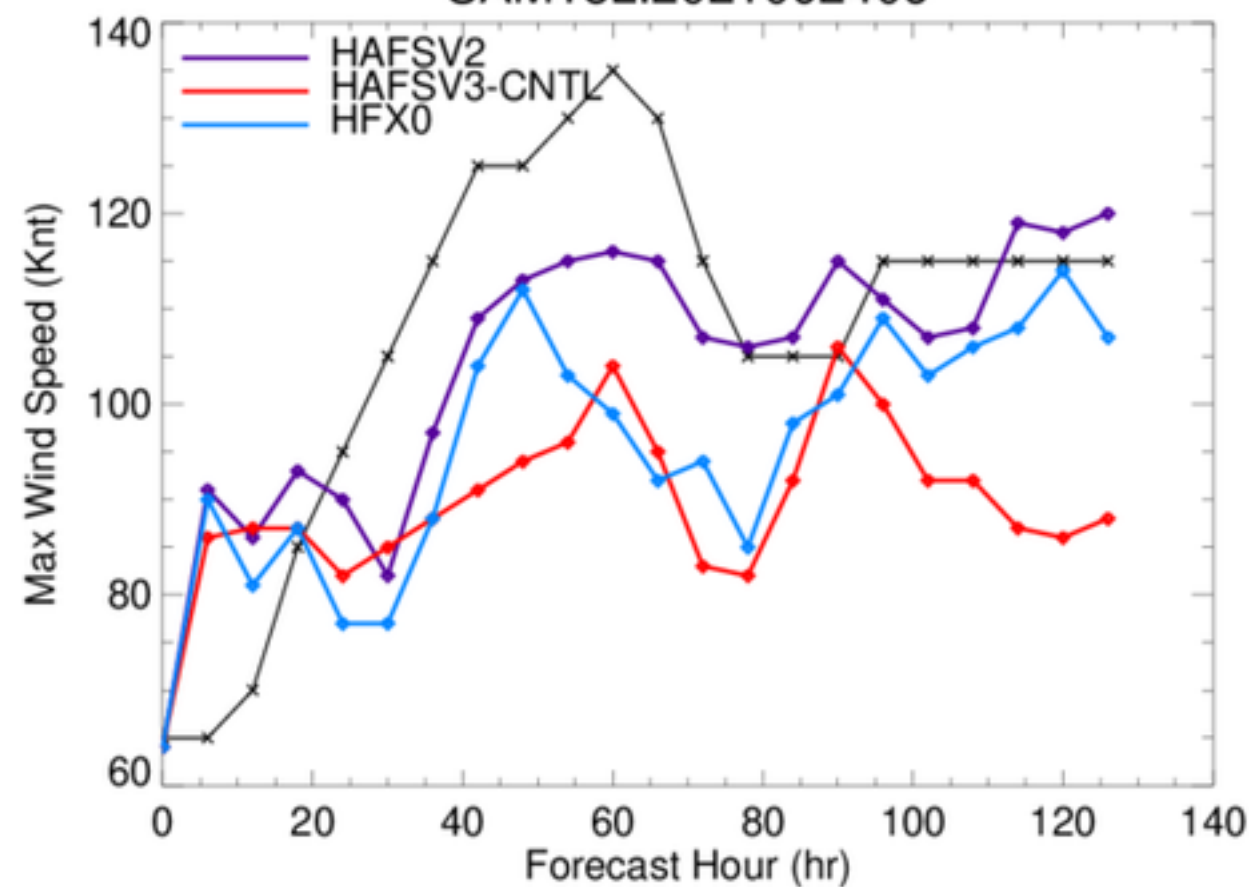
SAM18L.2021092406
