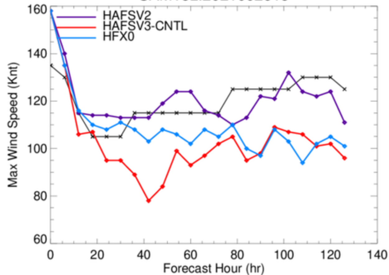
SAM18L.2021092618
