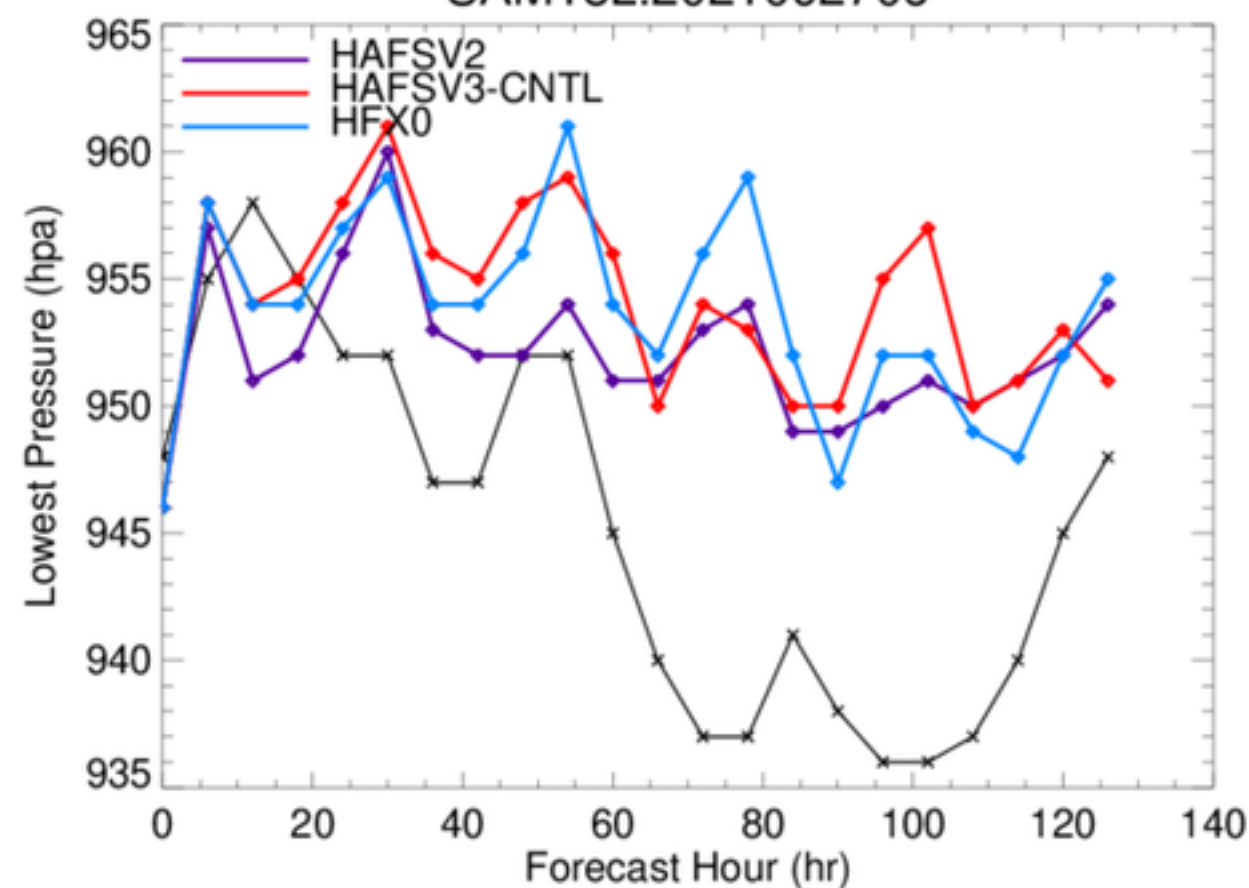
SAM18L.2021092706
