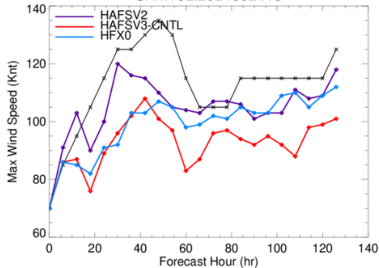
SAM18L.2021092418
