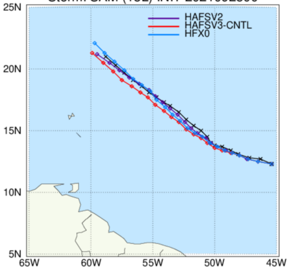
HWRF: TC Tracks Storm: SAM (18L) INIT 2021092500
