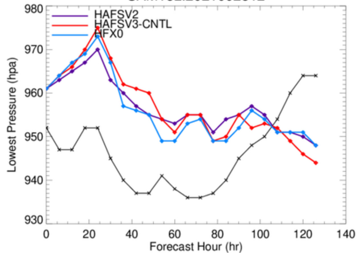
SAM18L.2021092812
