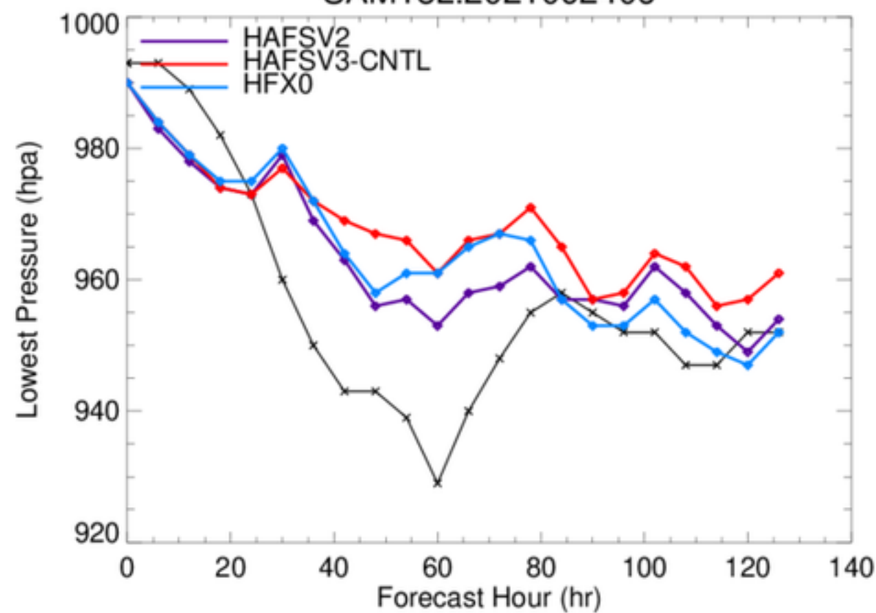
SAM18L.2021092406
