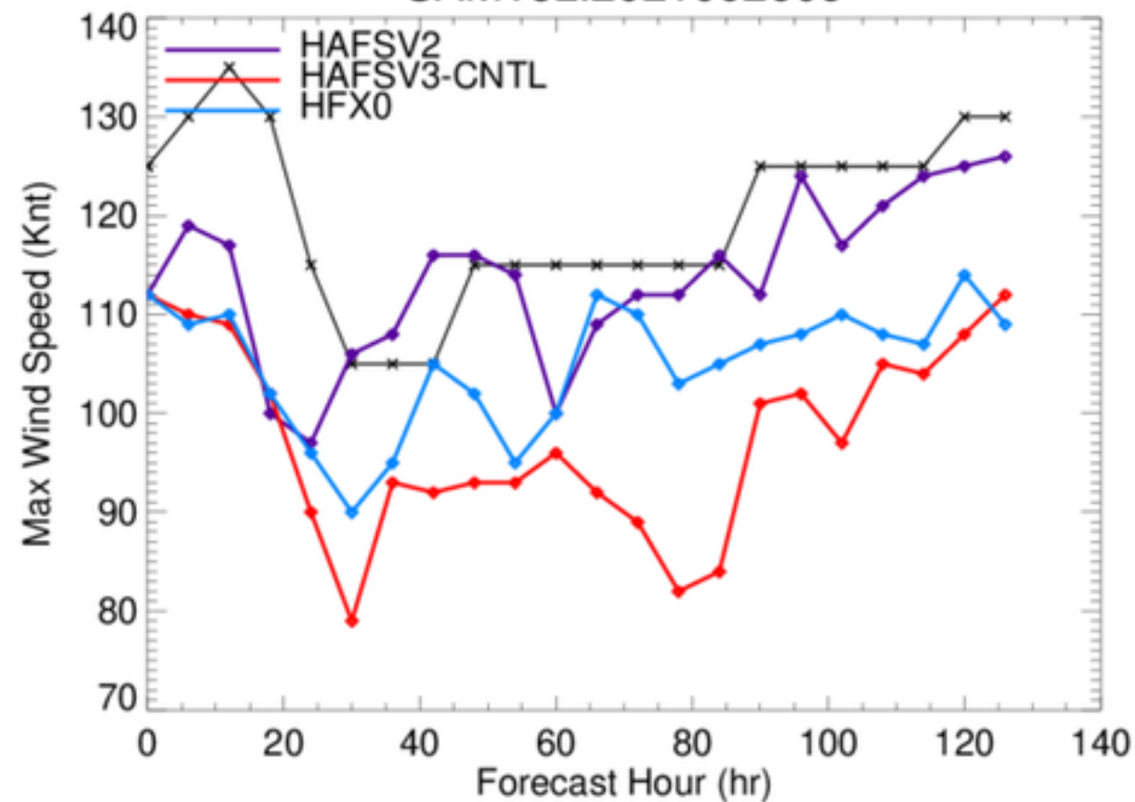
SAM18L.2021092606
