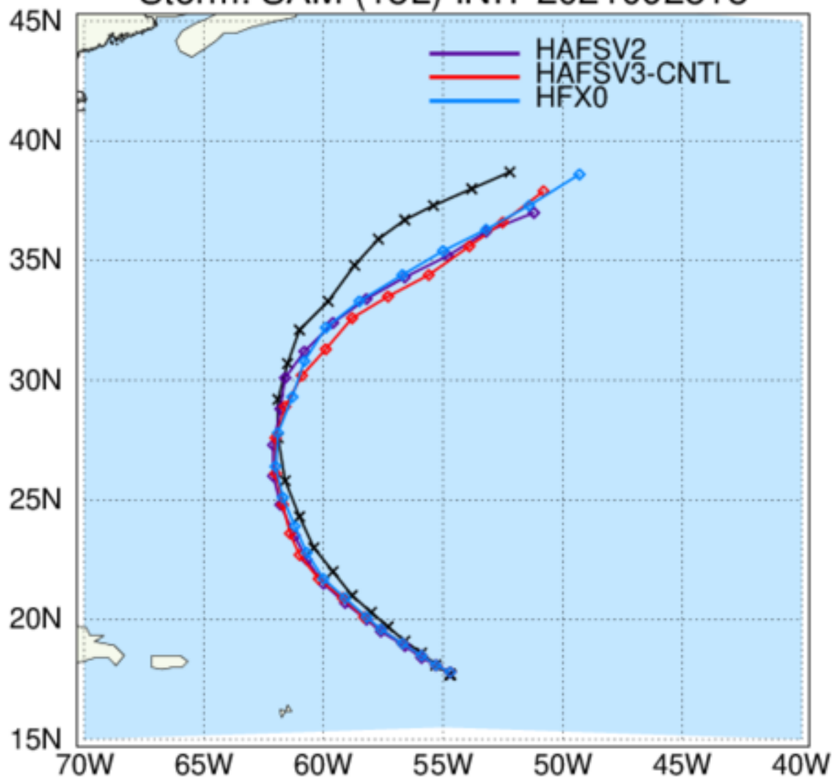
HWRF: TC Tracks Storm: SAM (18L) INIT 2021092818
