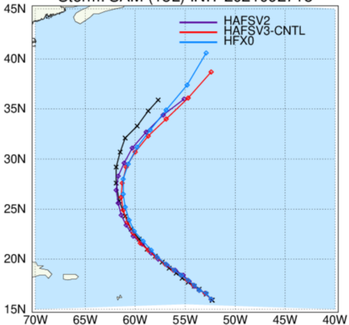
HWRF: TC Tracks Storm: SAM (18L) INIT 2021092718
