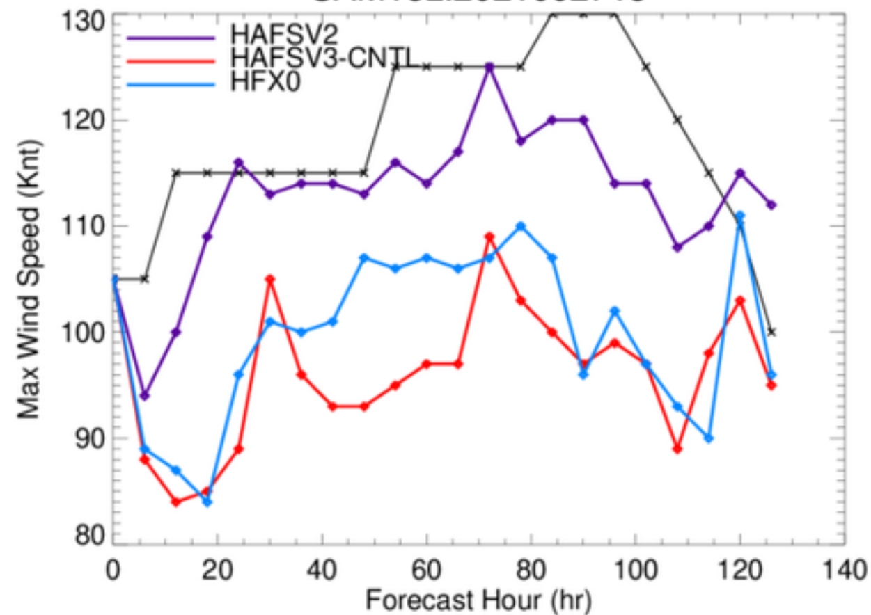
SAM18L.2021092718
