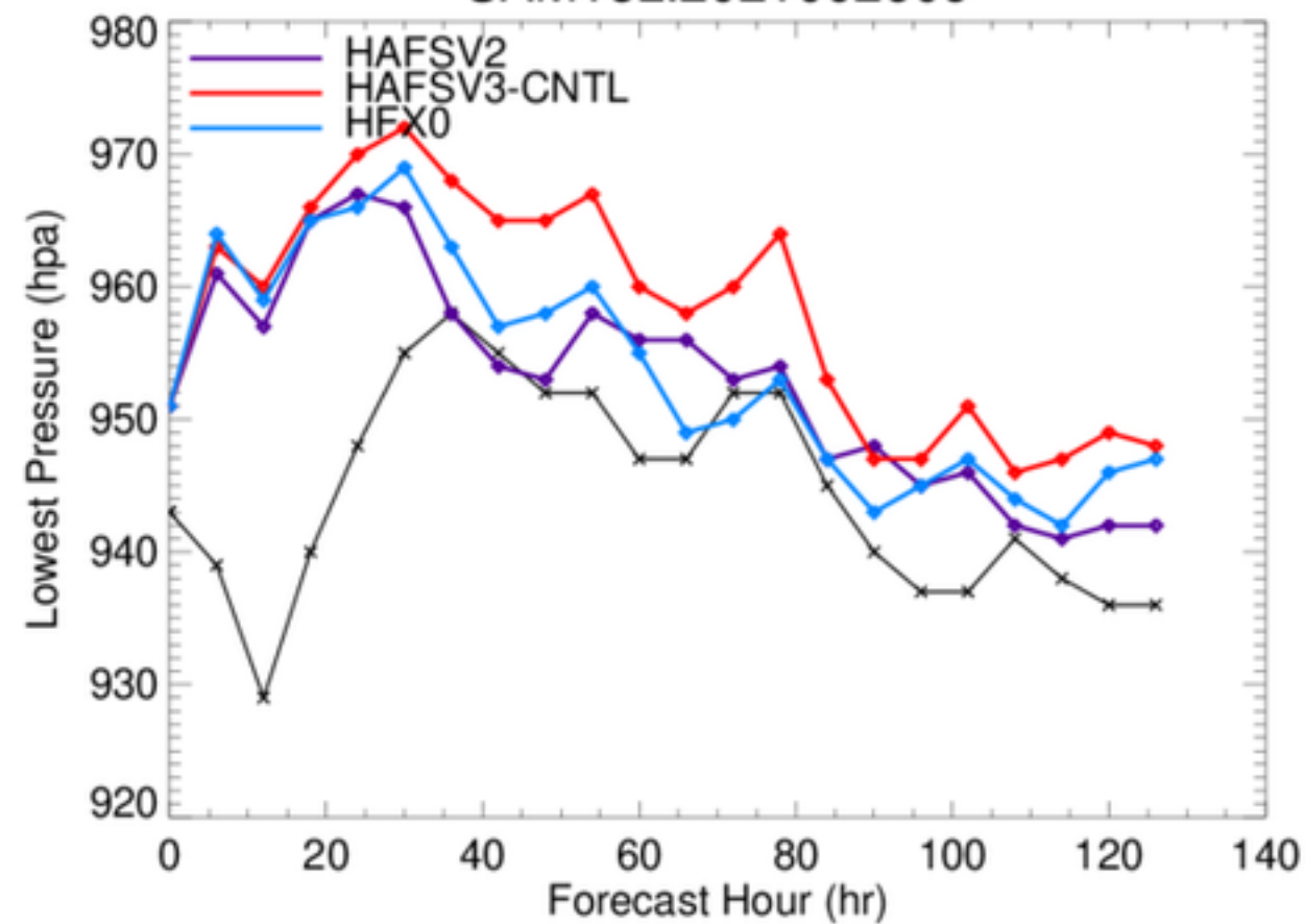
SAM18L.2021092606
