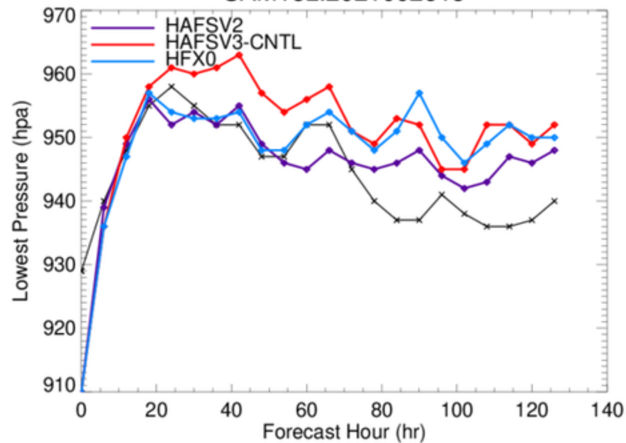
SAM18L.2021092618
