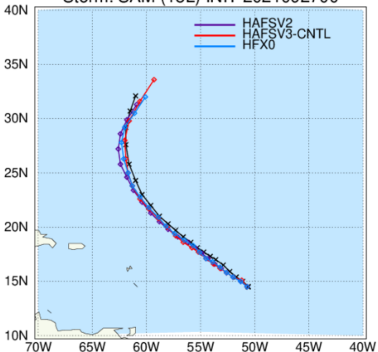
HWRF: TC Tracks Storm: SAM (18L) INIT 2021092700
