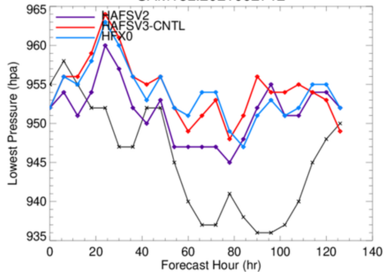
SAM18L.2021092712
