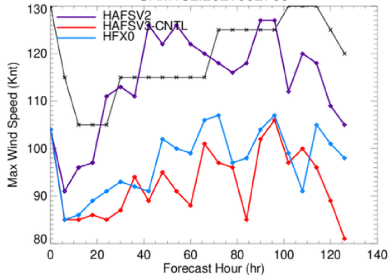
SAM18L.2021092700
