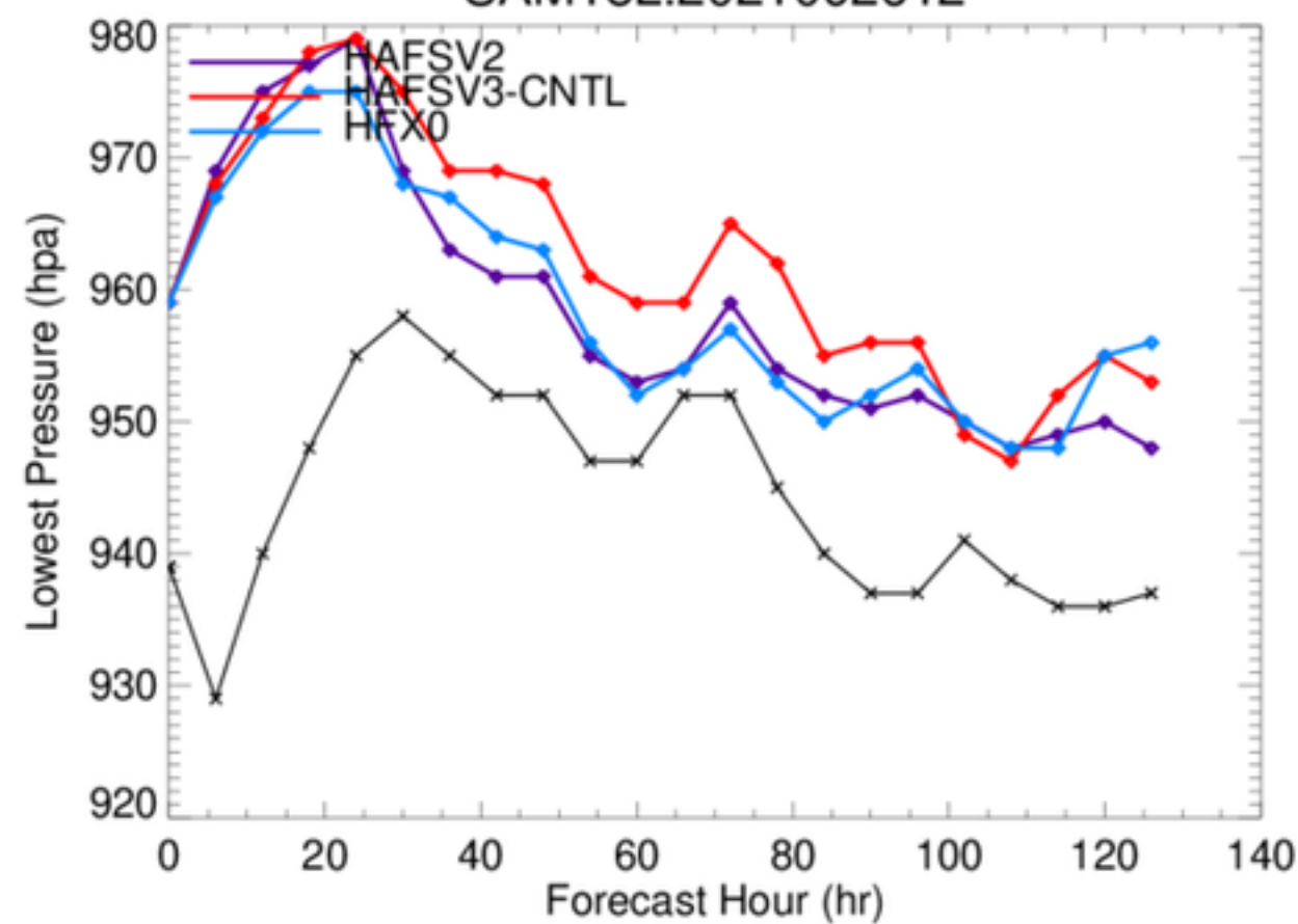
SAM18L.2021092612
