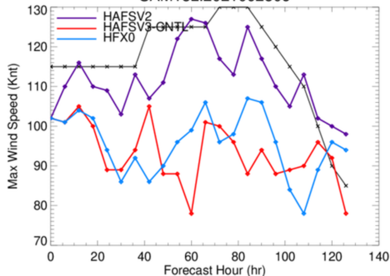
SAM18L.2021092806
