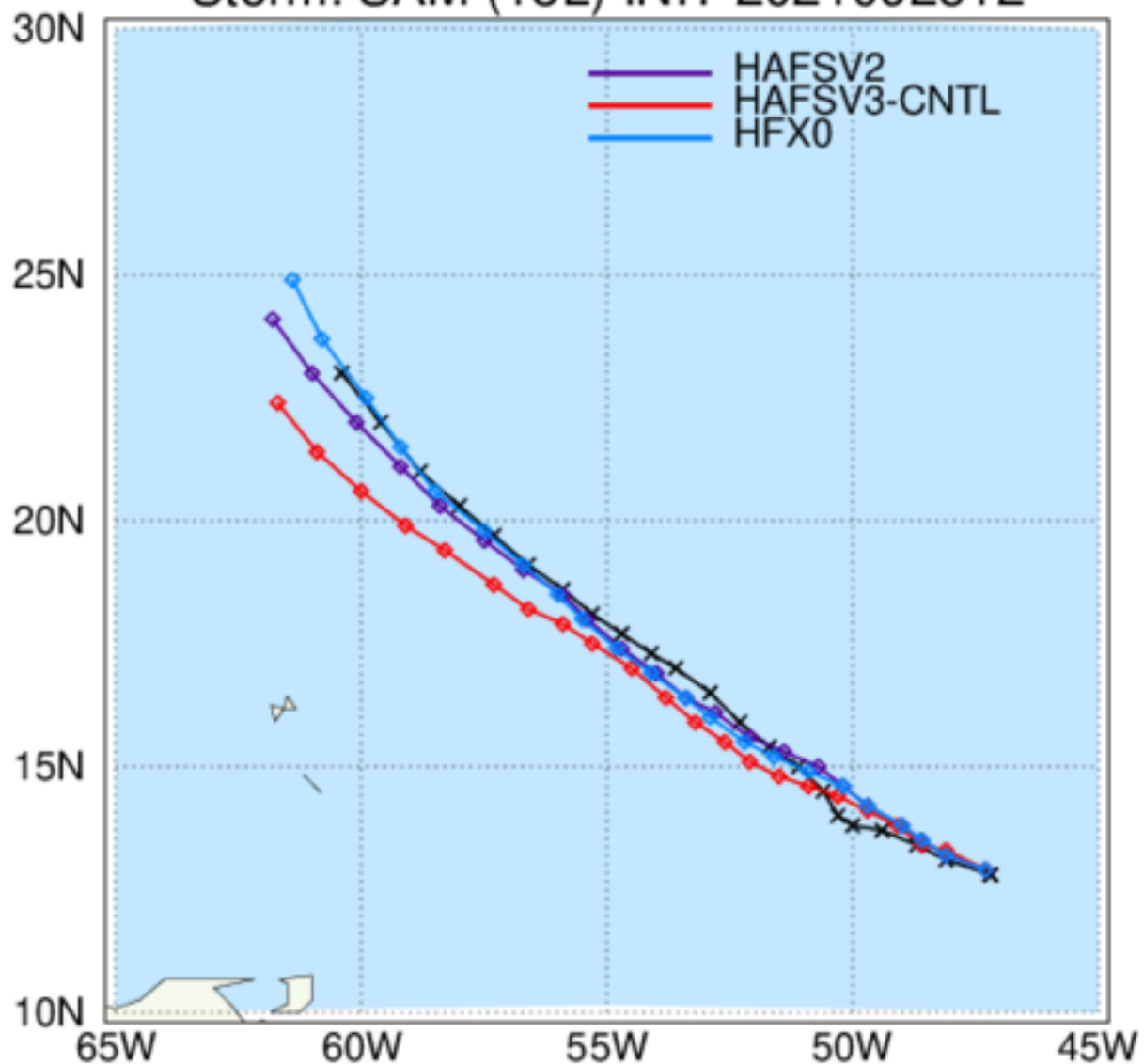
HWRF: TC Tracks Storm: SAM (18L) INIT 2021092512
