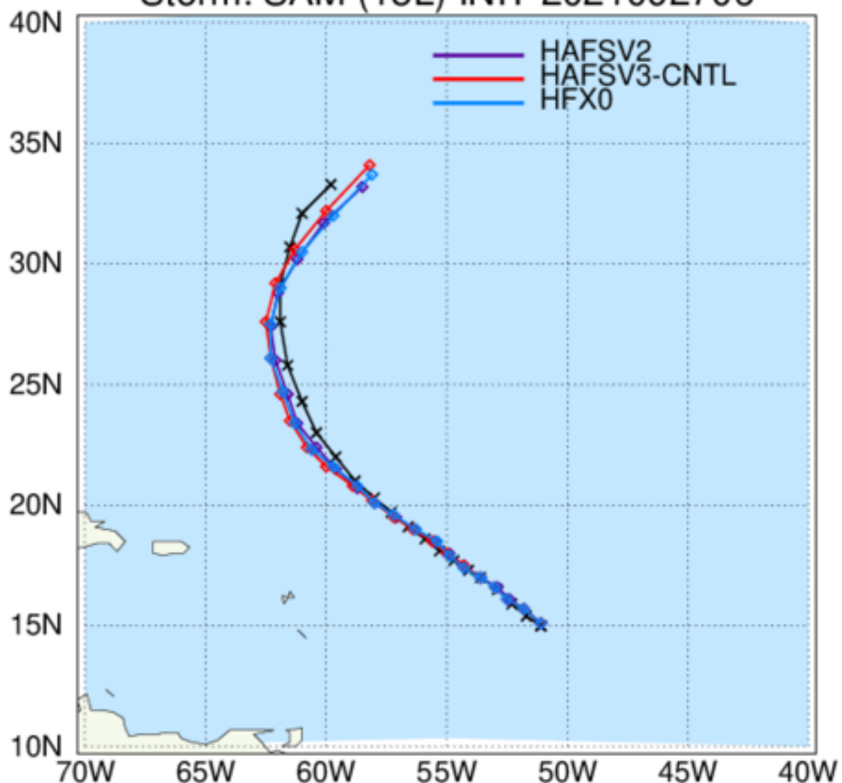
HWRF: TC Tracks Storm: SAM (18L) INIT 2021092706
