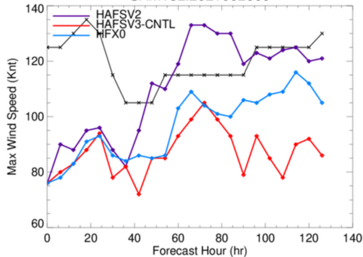
SAM18L.2021092600
