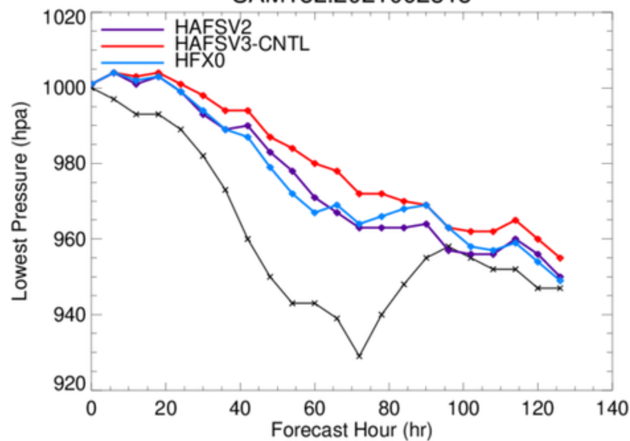
SAM18L.2021092318
