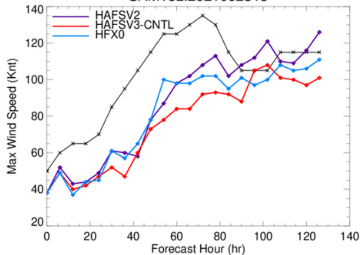
SAM18L.2021092318
