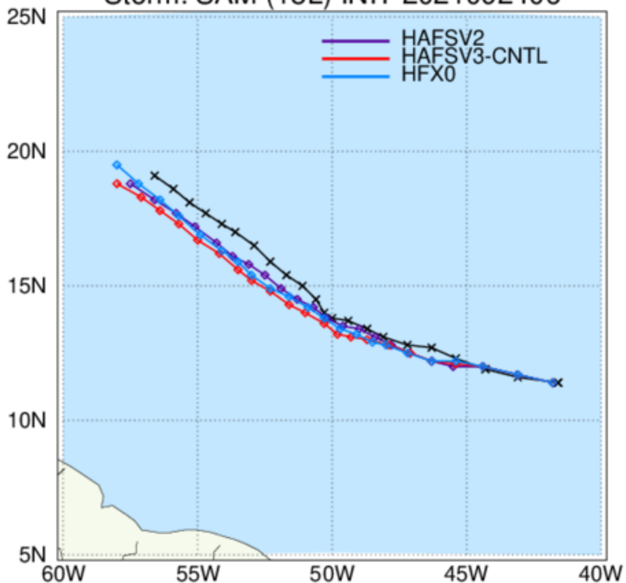
HWRF: TC Tracks Storm: SAM (18L) INIT 2021092406
