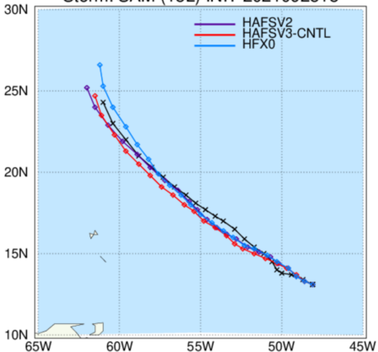
HWRF: TC Tracks Storm: SAM (18L) INIT 2021092518
