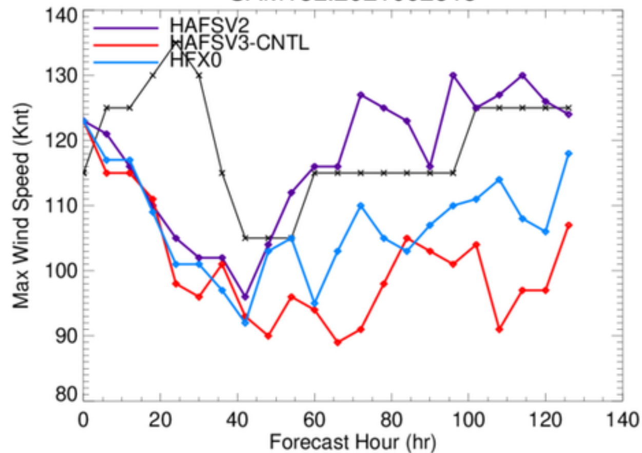
SAM18L.2021092518
