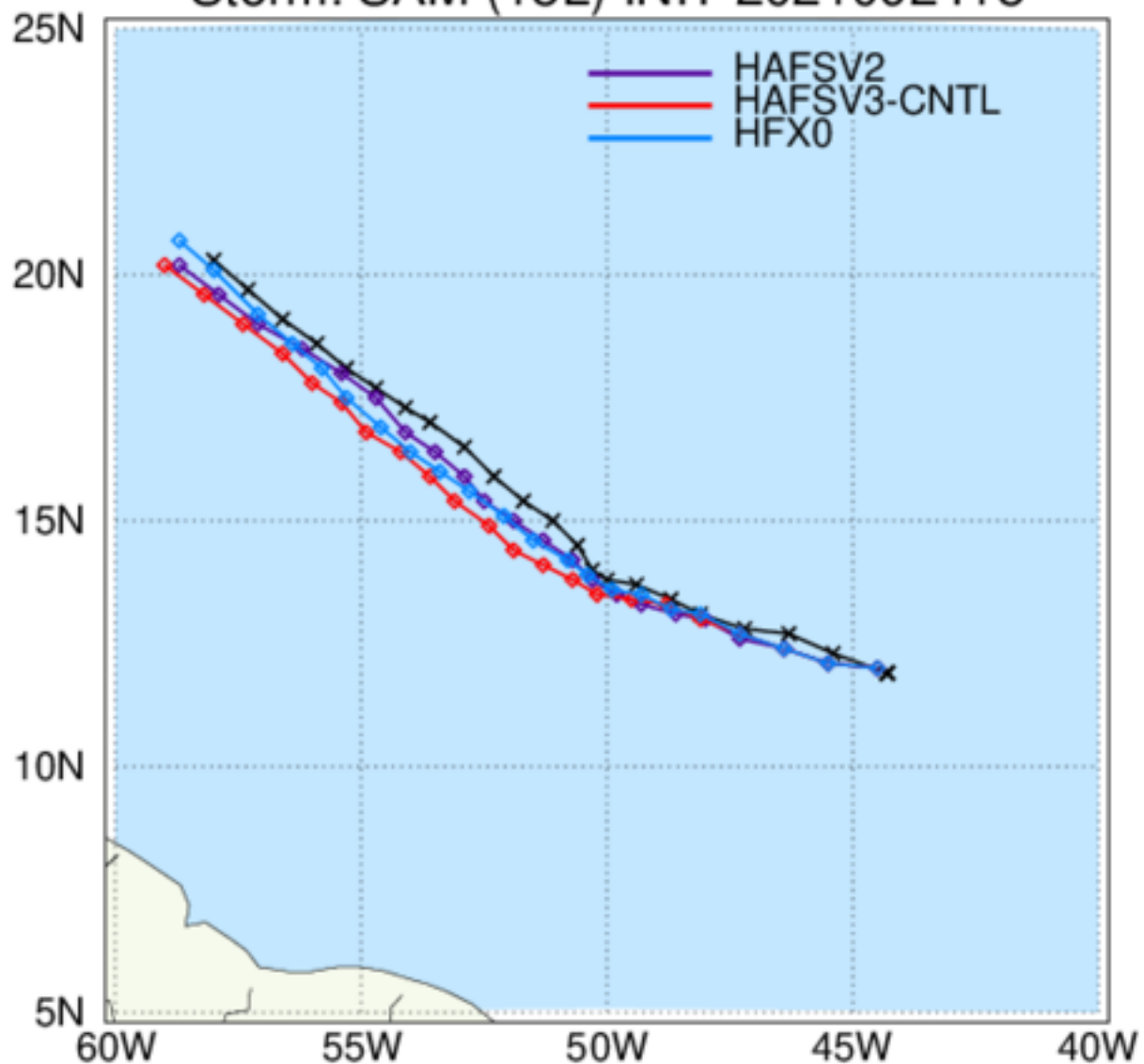
HWRF: TC Tracks Storm: SAM (18L) INIT 2021092418
