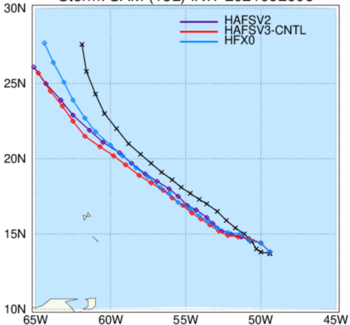
HWRF: TC Tracks Storm: SAM (18L) INIT 2021092606
