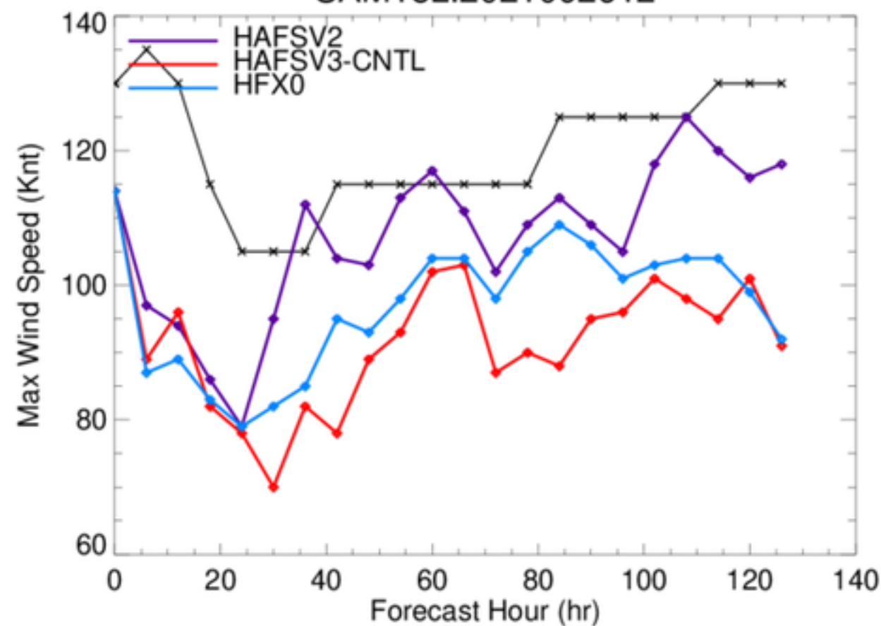
SAM18L.2021092612
