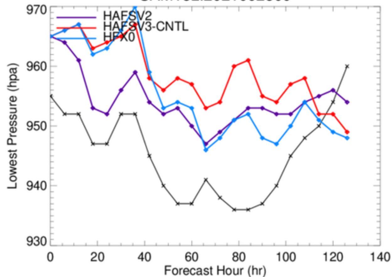
SAM18L.2021092800
