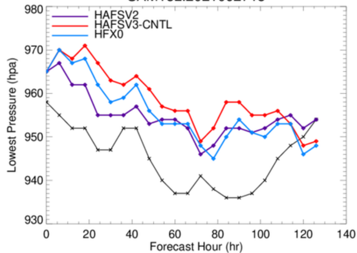
SAM18L.2021092718
