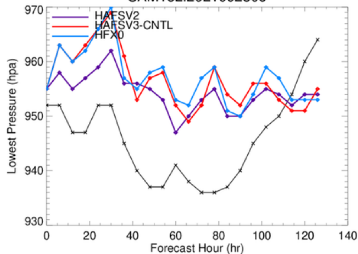
SAM18L.2021092806
