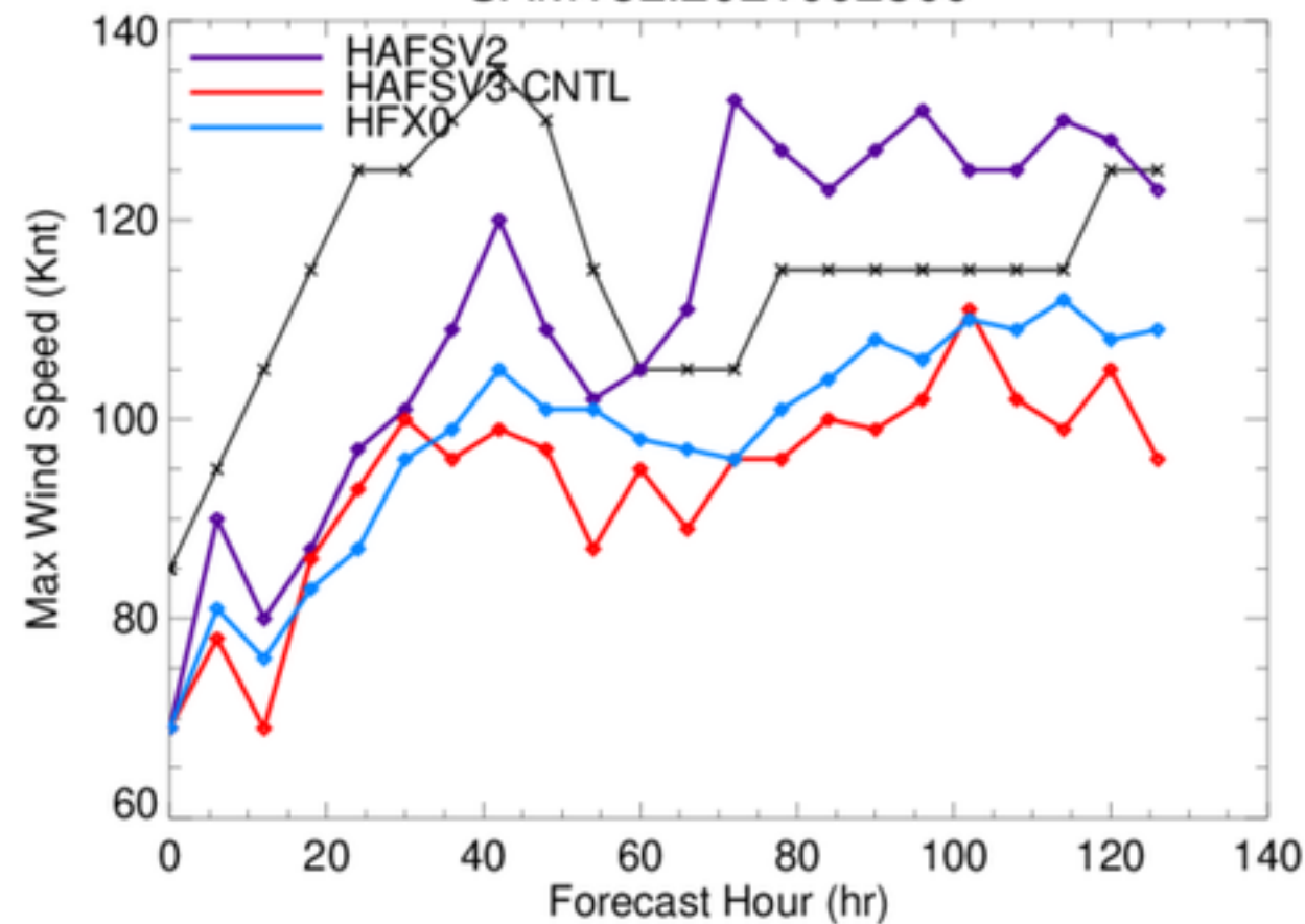
SAM18L.2021092500
