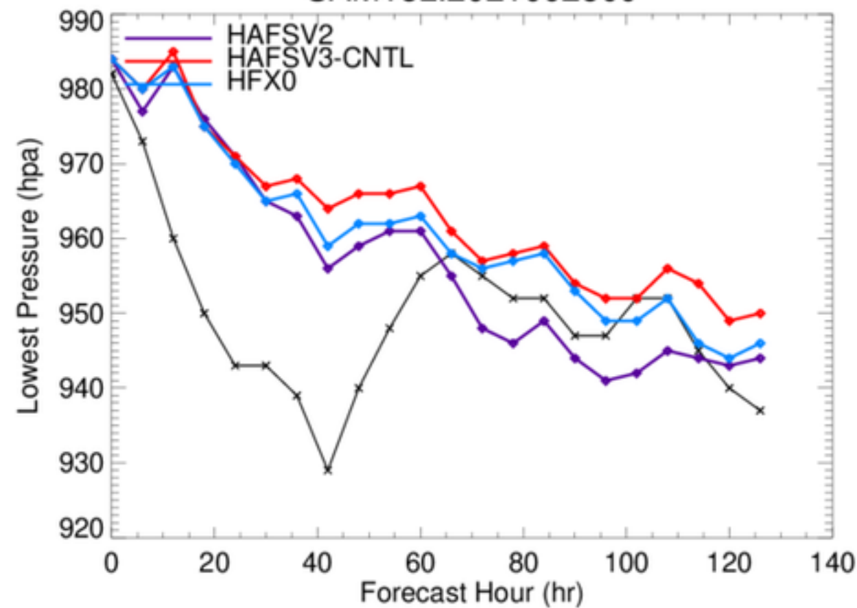
SAM18L.2021092500
