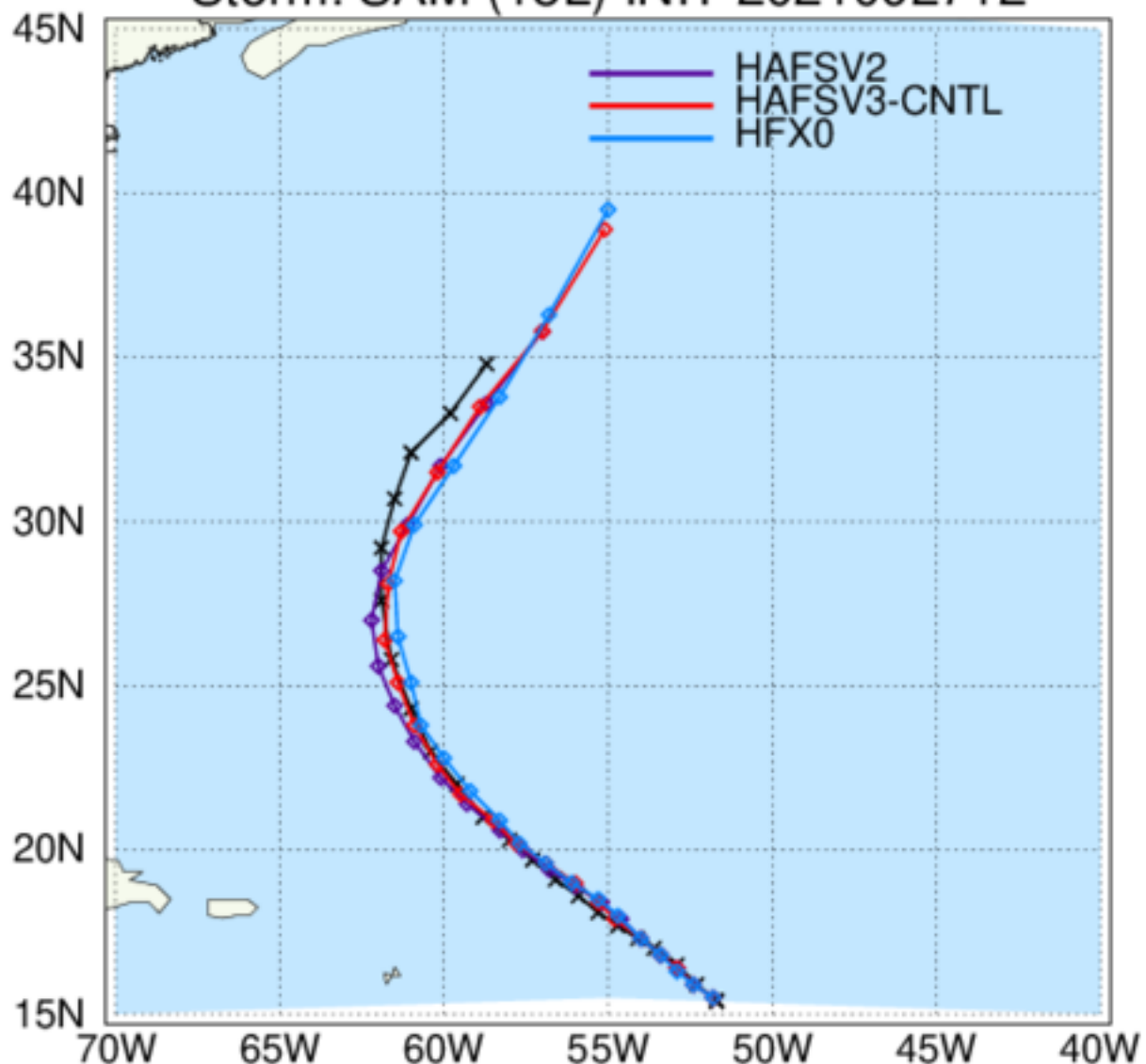
HWRF: TC Tracks Storm: SAM (18L) INIT 2021092712
