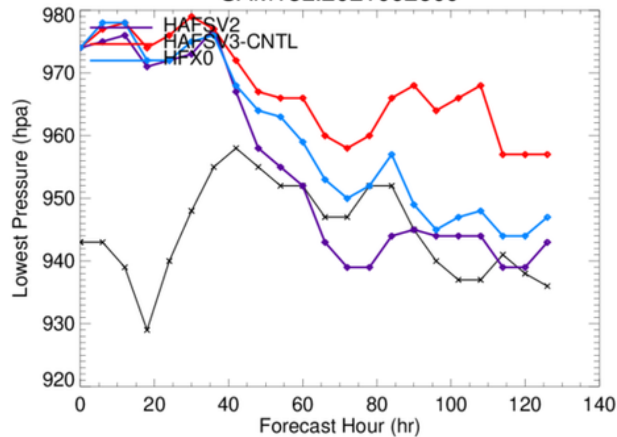
SAM18L.2021092600
