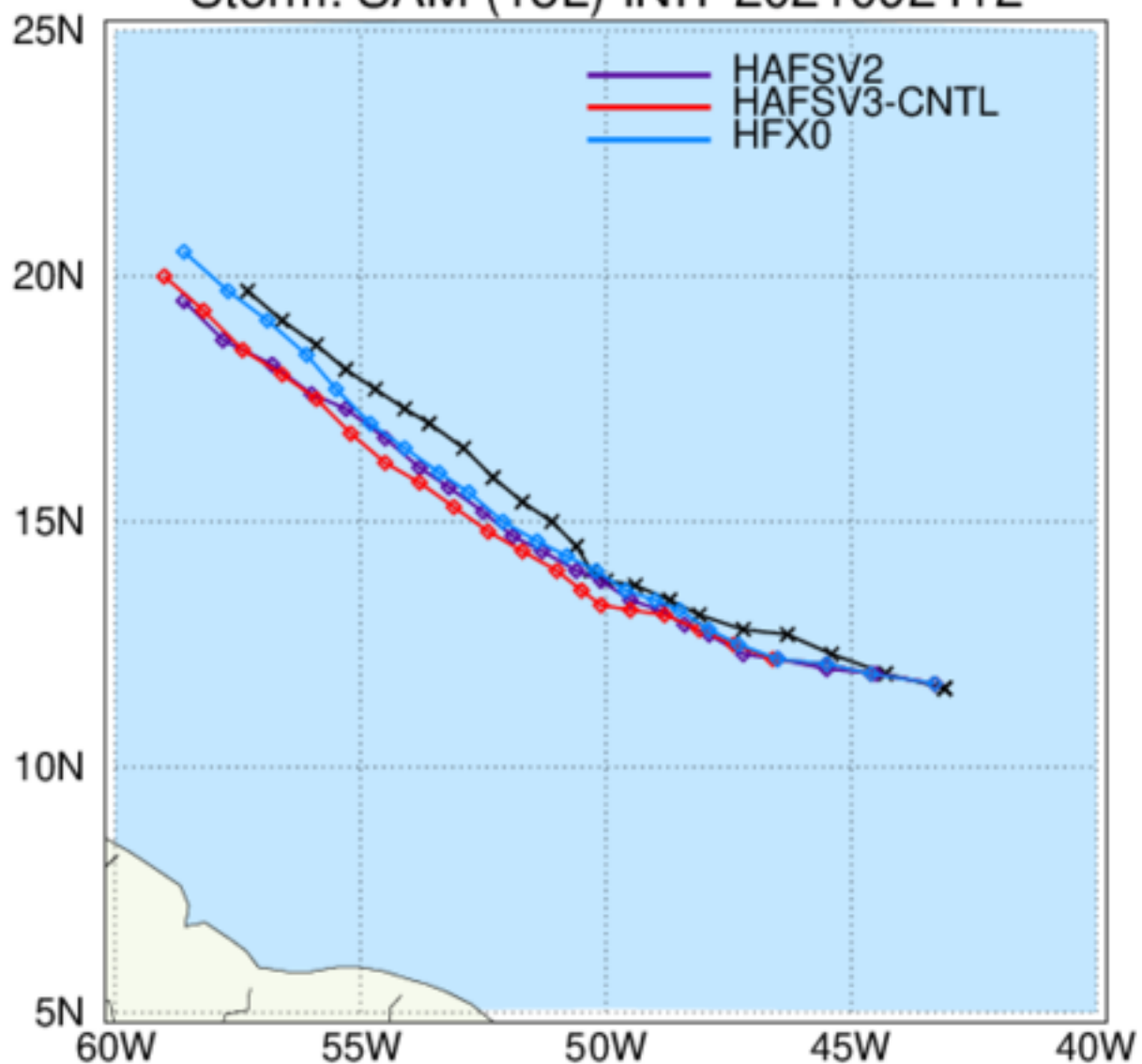
HWRF: TC Tracks Storm: SAM (18L) INIT 2021092412
