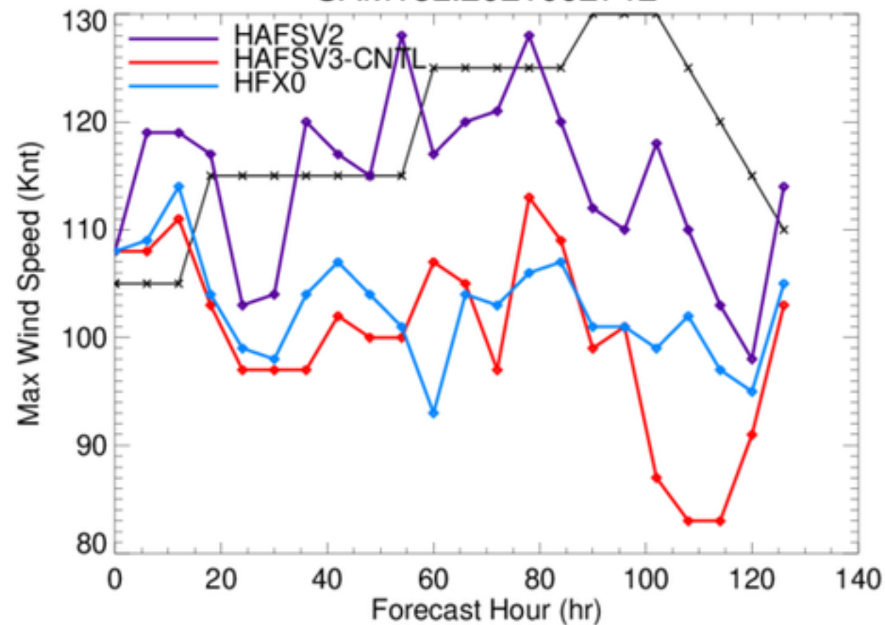
SAM18L.2021092712
