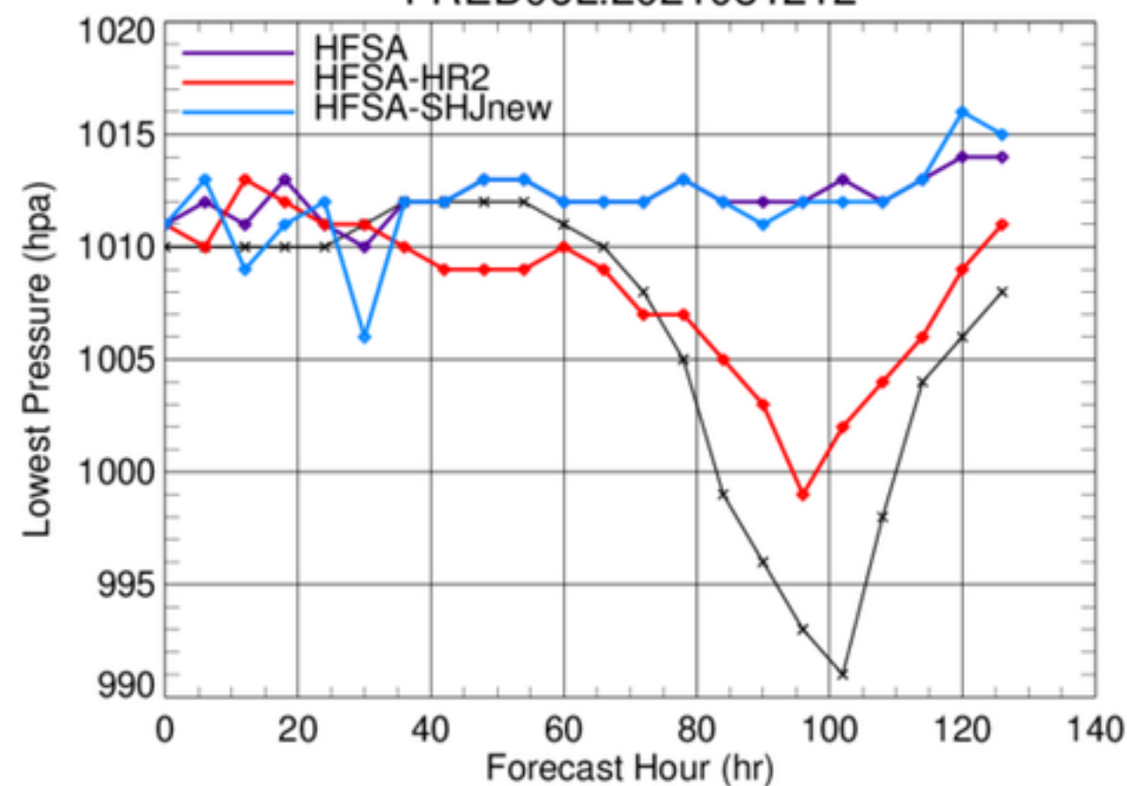
FRED06L.2021081212
