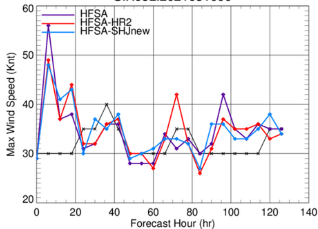
SIX06L.2021081000
