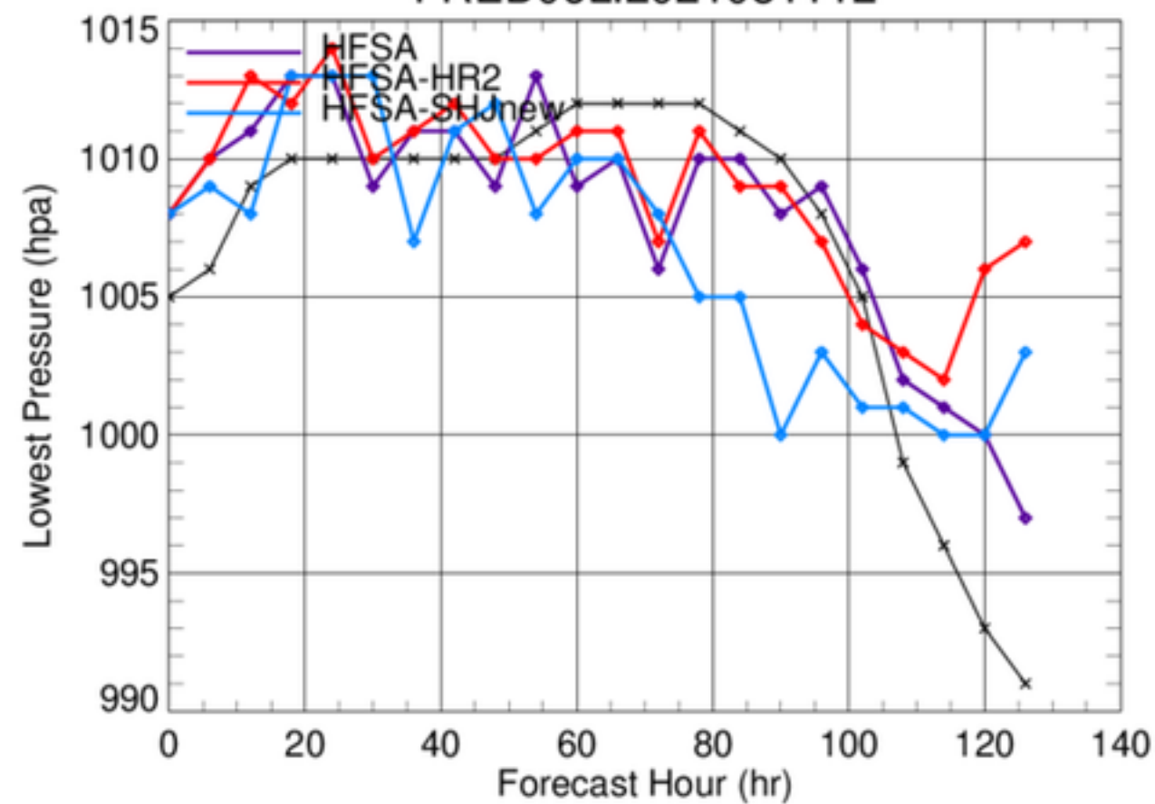
FRED06L.2021081112
