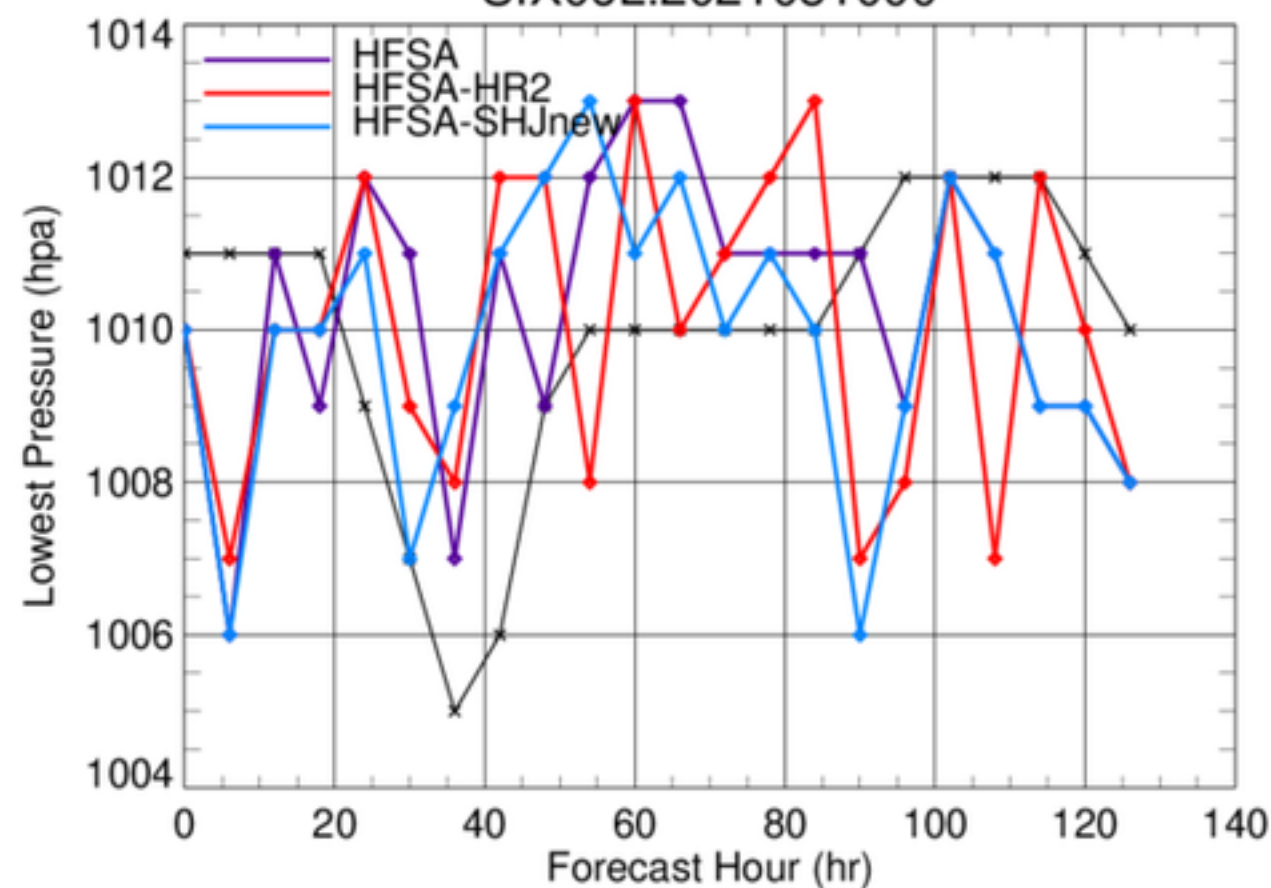
SIX06L.2021081000
