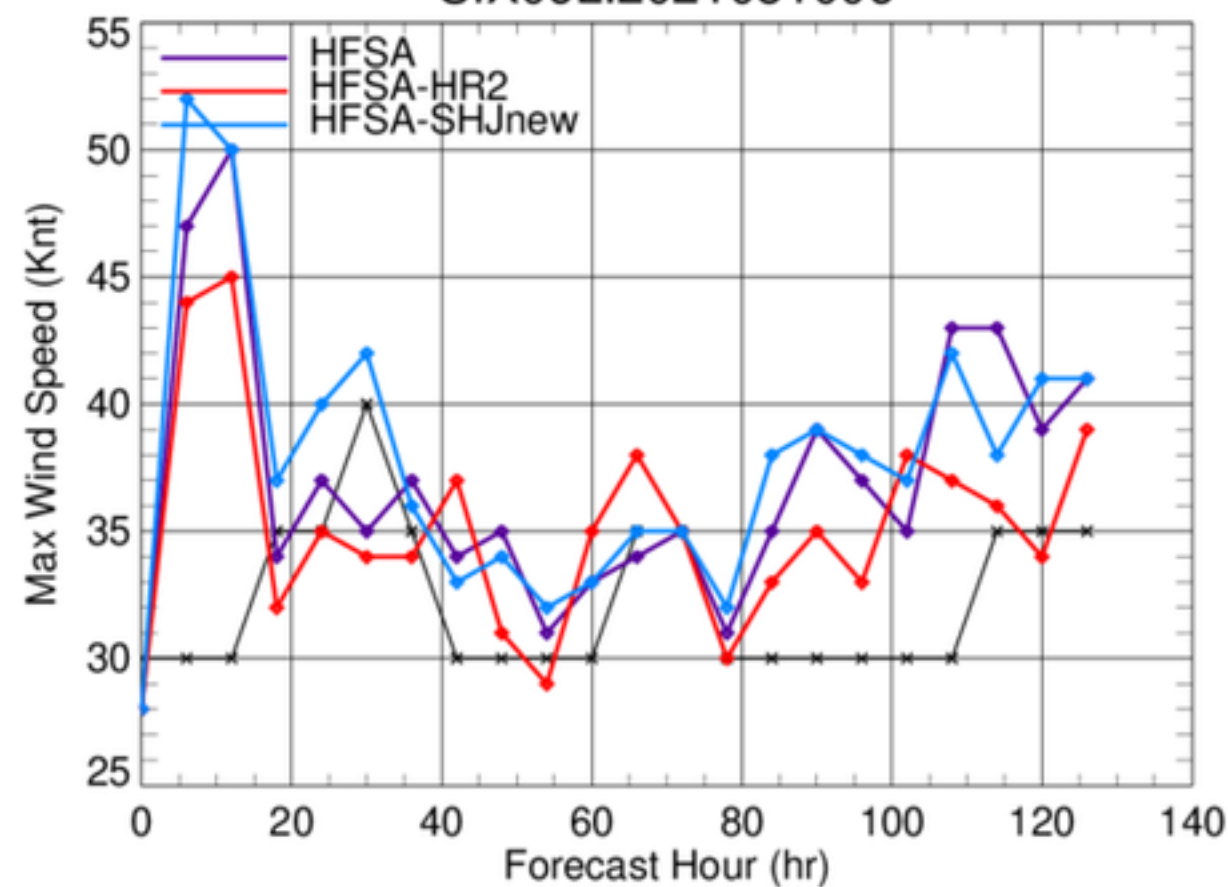
SIX06L.2021081006
