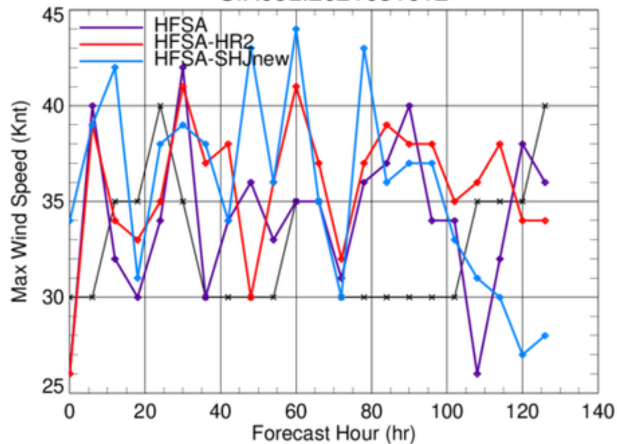
SIX06L.2021081012
