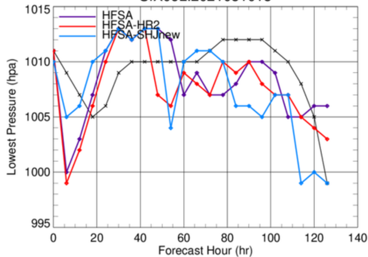
SIX06L.2021081018
