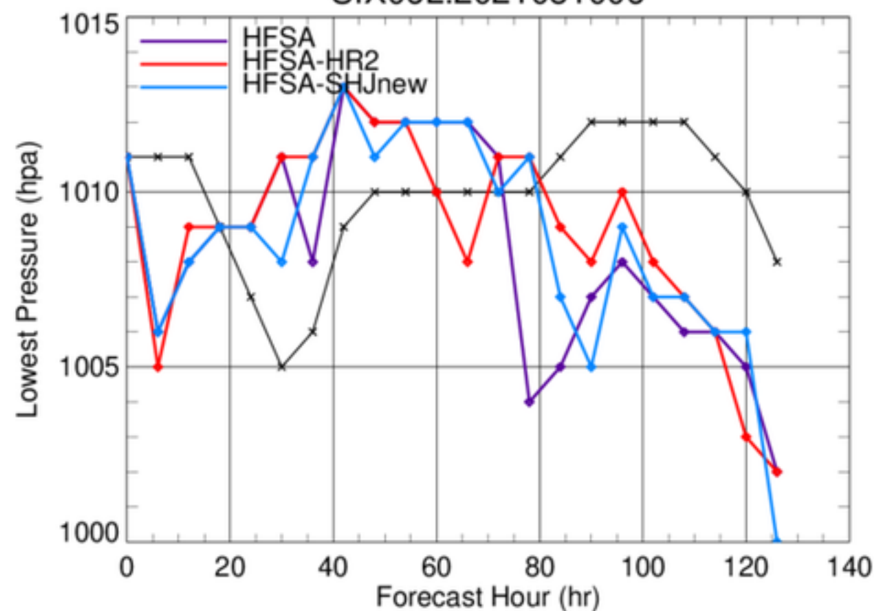
SIX06L.2021081006
