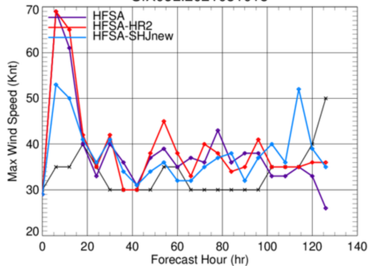
SIX06L.2021081018
