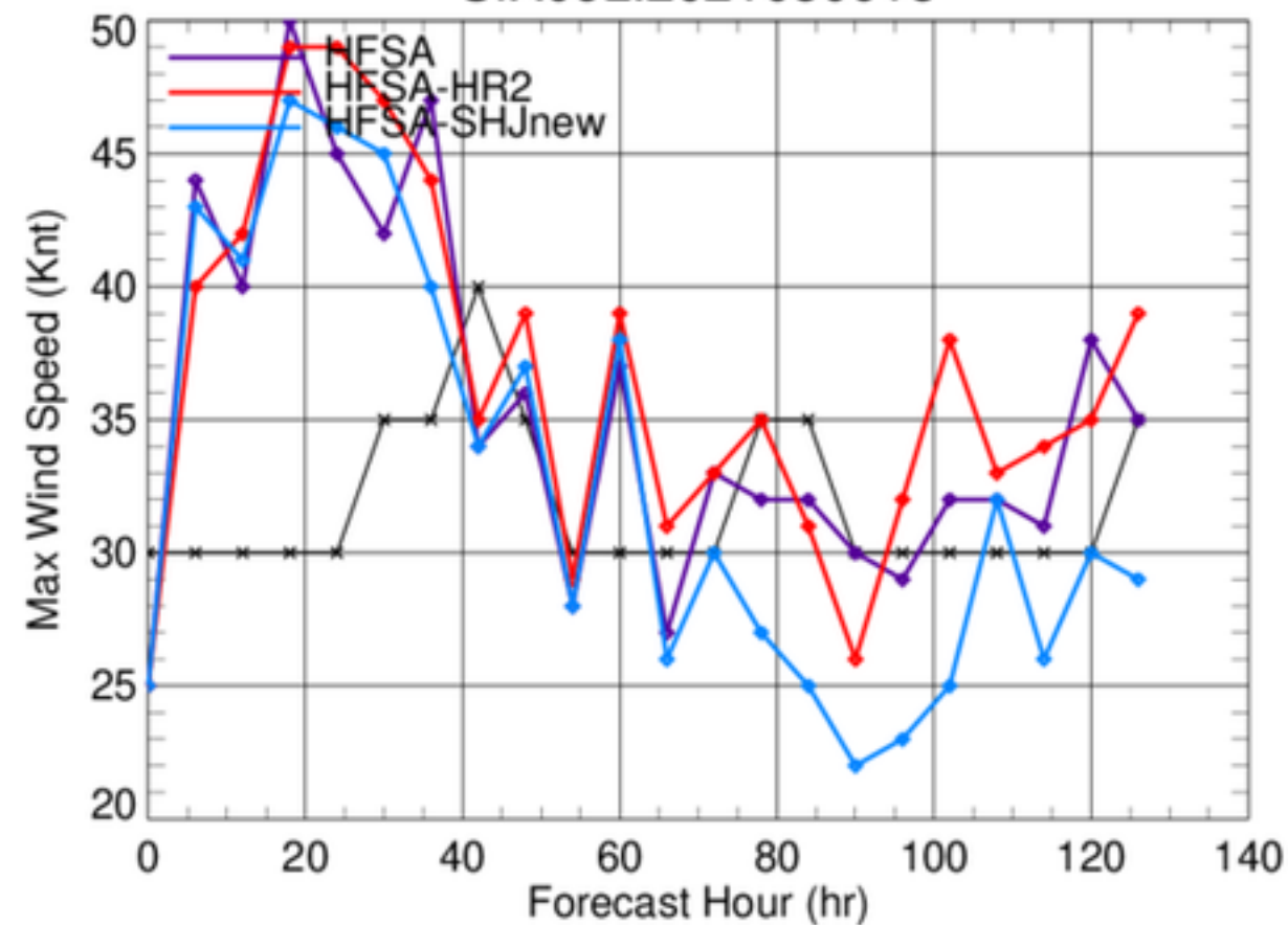
SIX06L.2021080918
