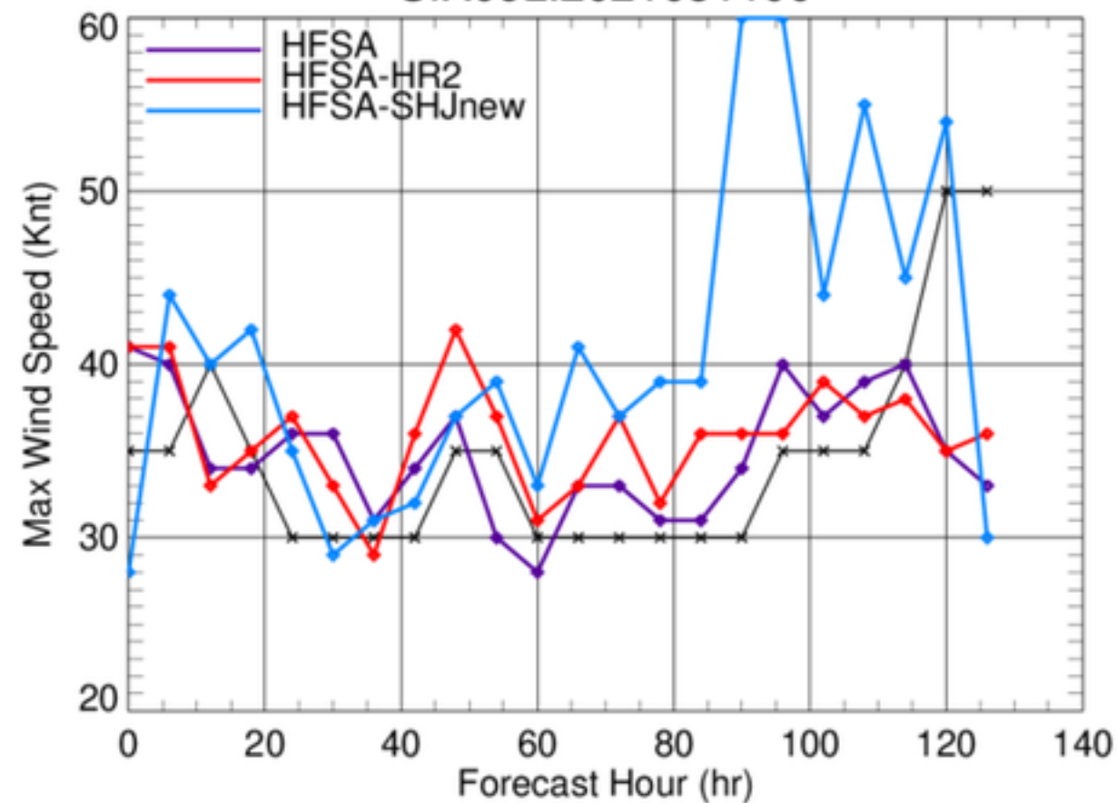
SIX06L.2021081100
