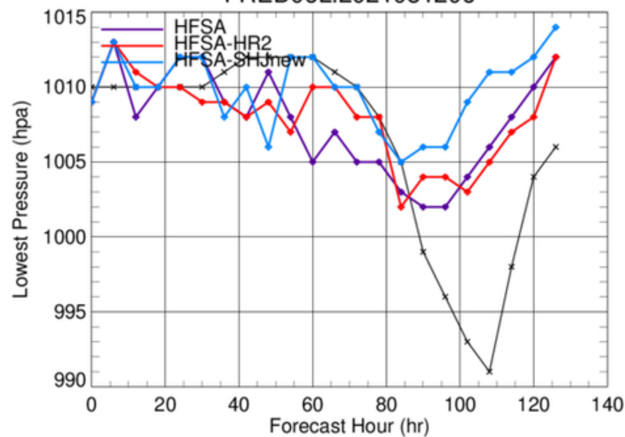
FRED06L.2021081206
