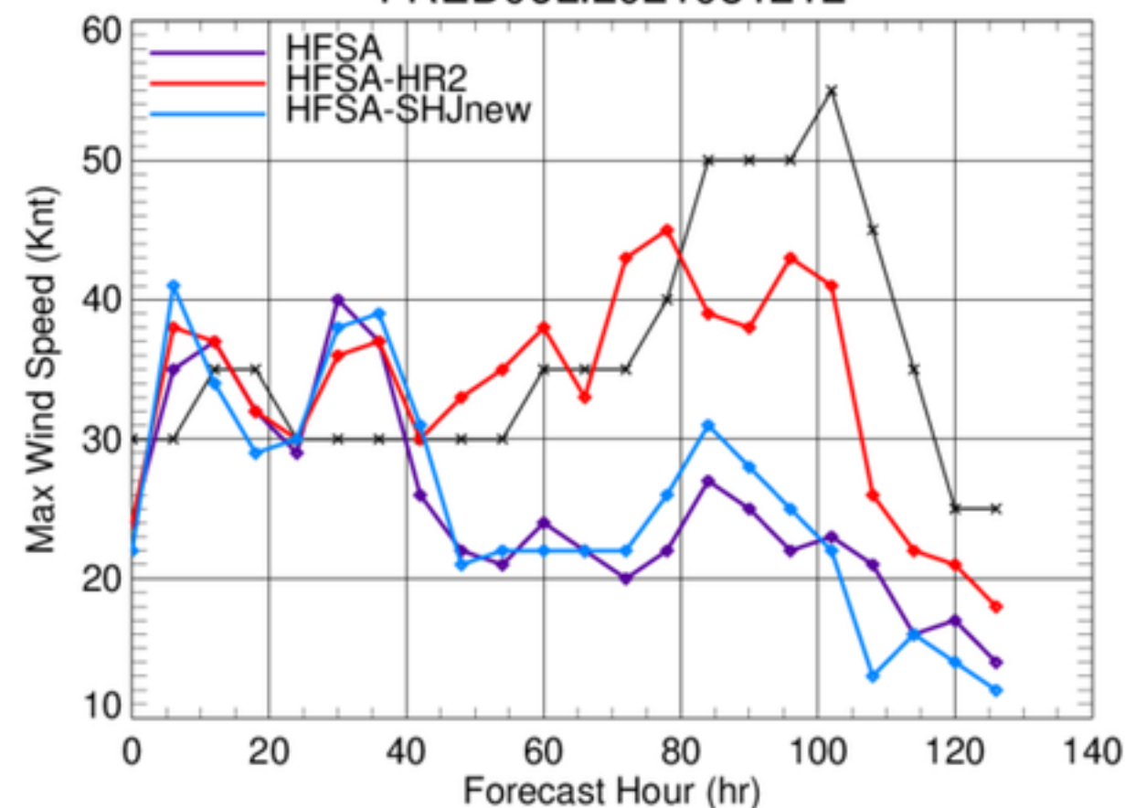
FRED06L.2021081212
