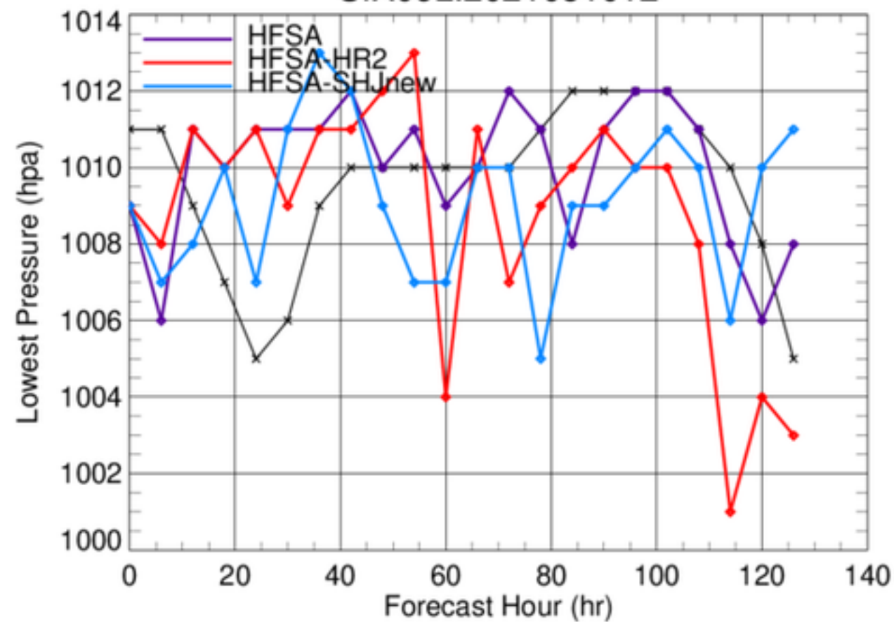
SIX06L.2021081012
