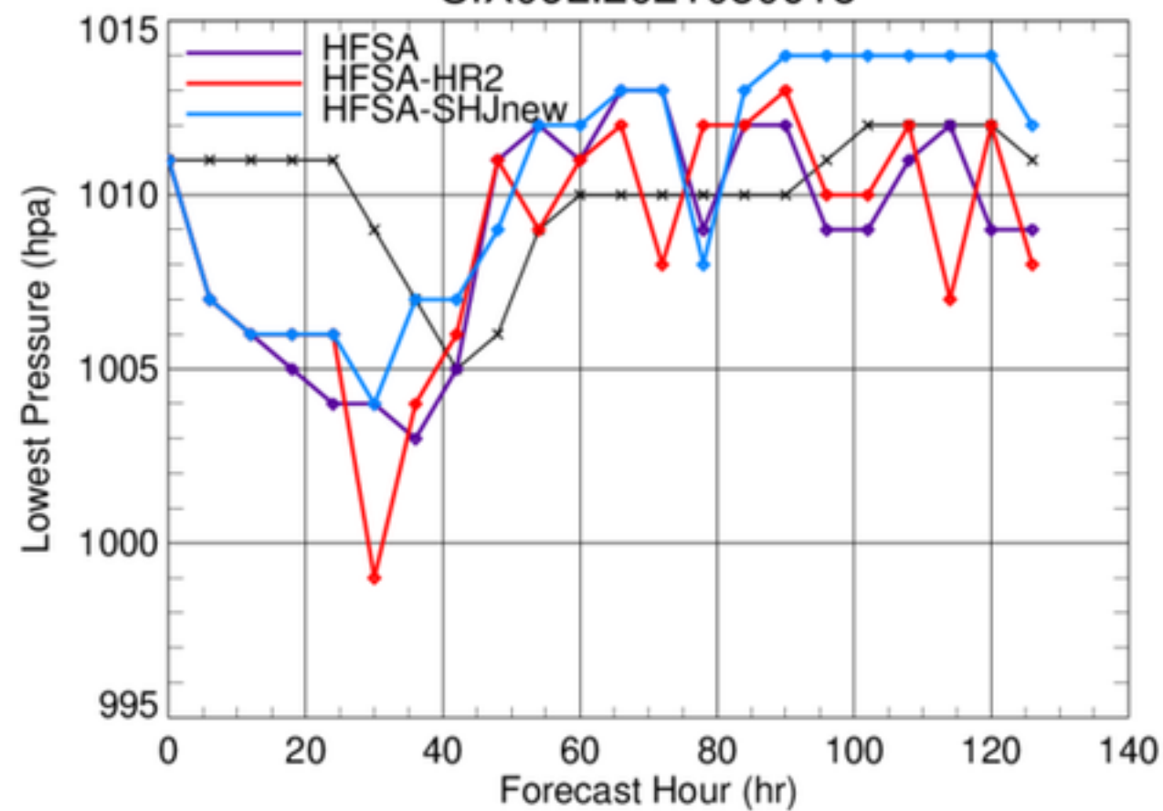
SIX06L.2021080918
