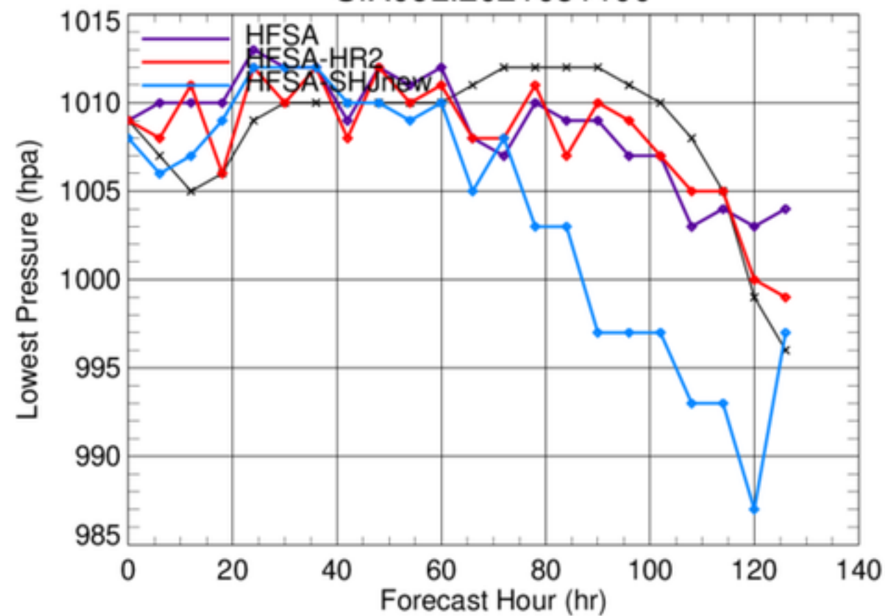
SIX06L.2021081100
