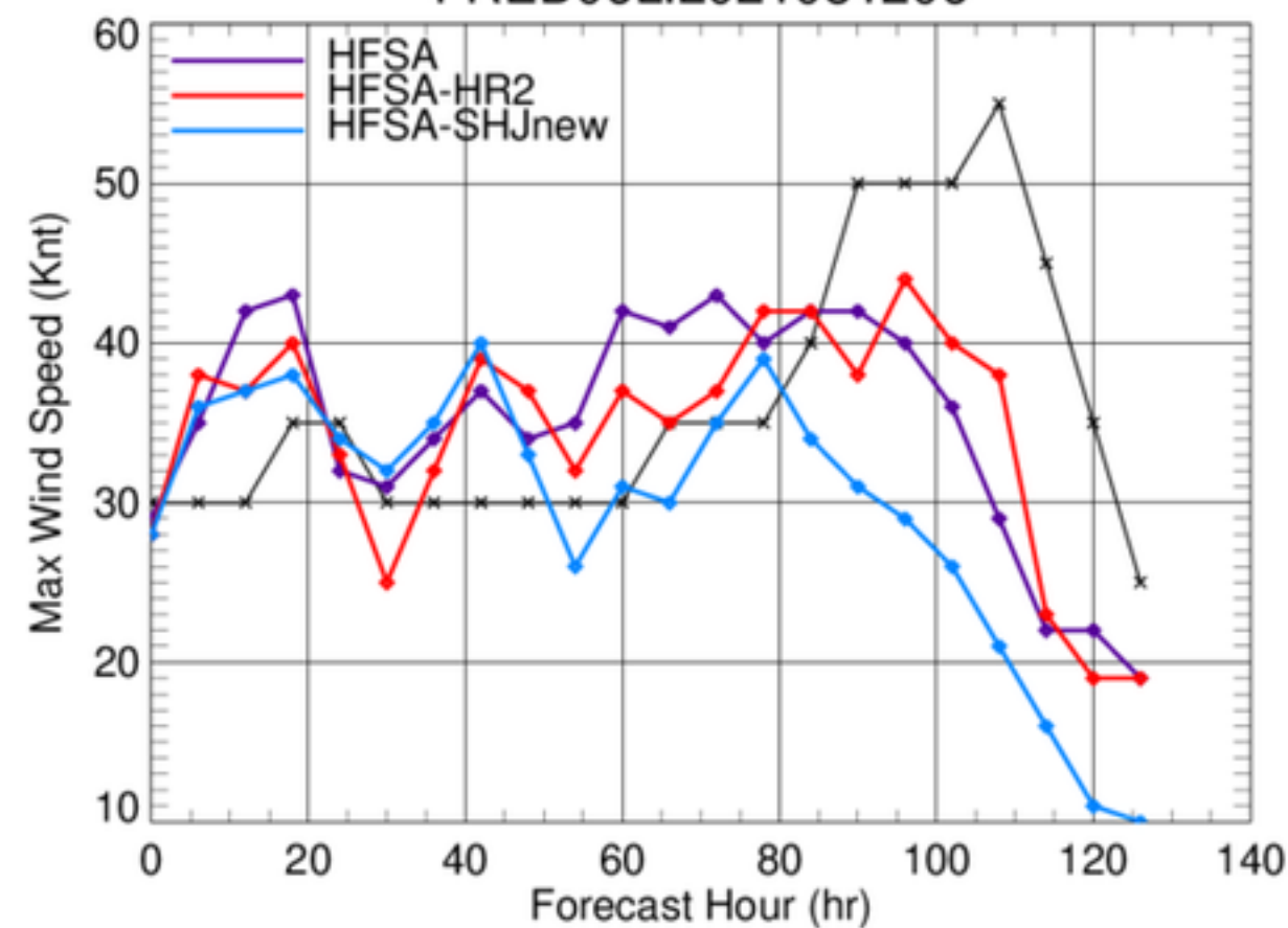
FRED06L.2021081206
