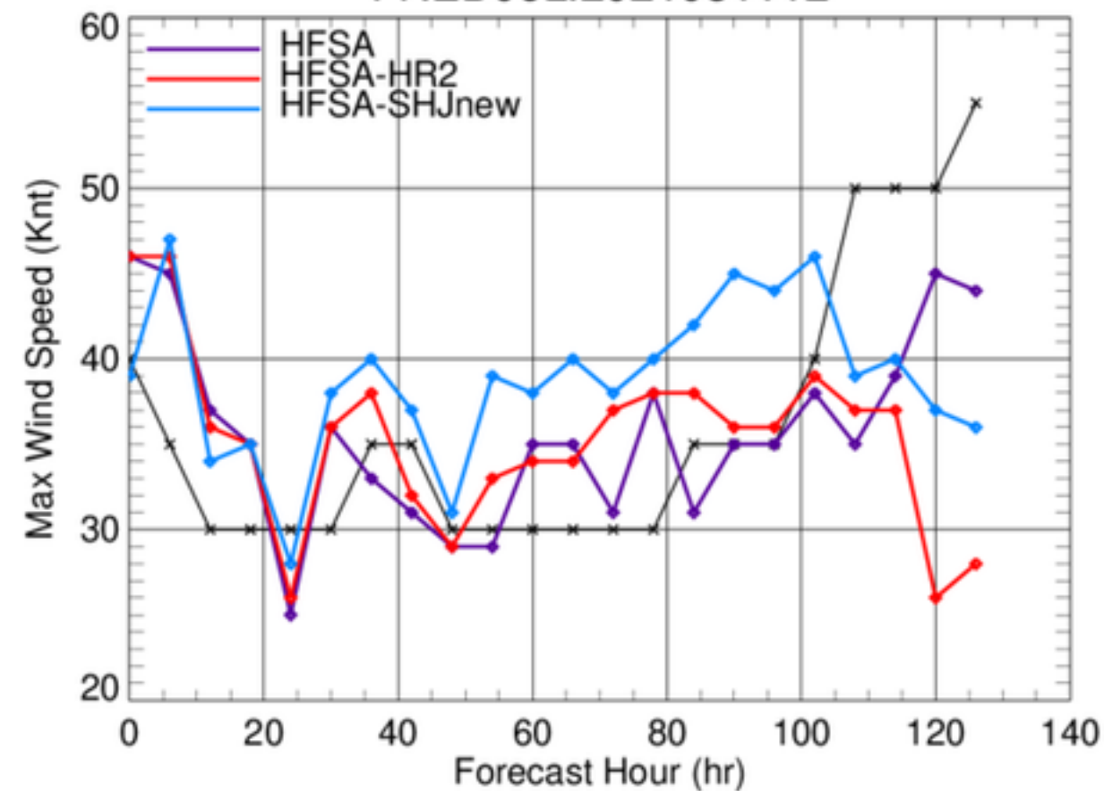
FRED06L.2021081112
