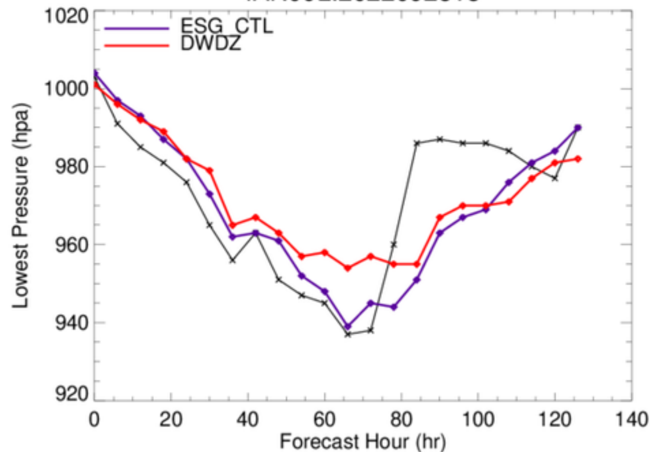
IAN09L.2022092518
