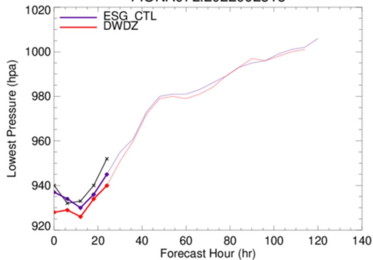
FIONA07L.2022092318
