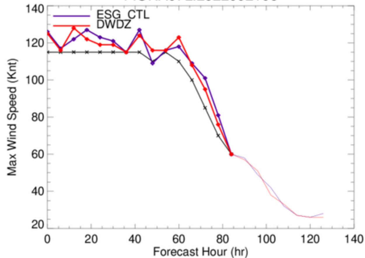
FIONA07L.2022092106
