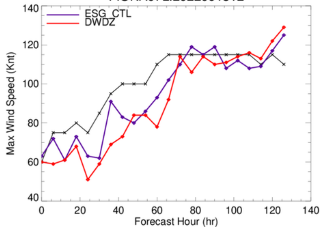
FIONA07L.2022091812
