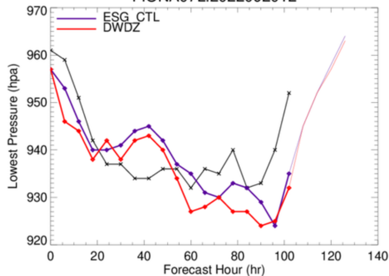
FIONA07L.2022092012
