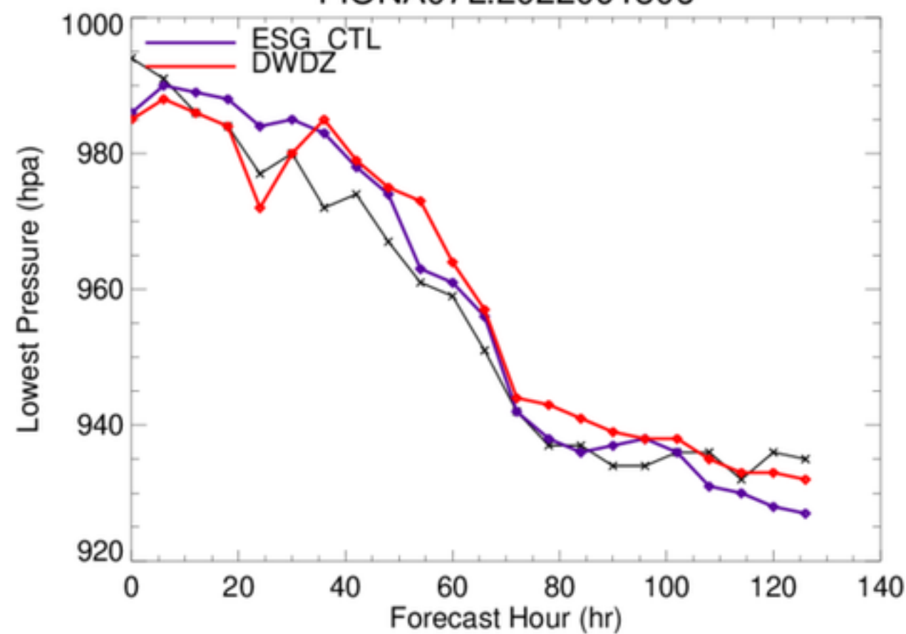
FIONA07L.2022091806
