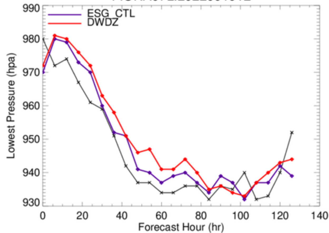
FIONA07L.2022091912
