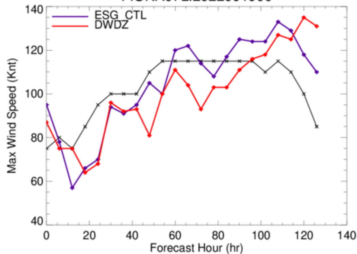
FIONA07L.2022091900
