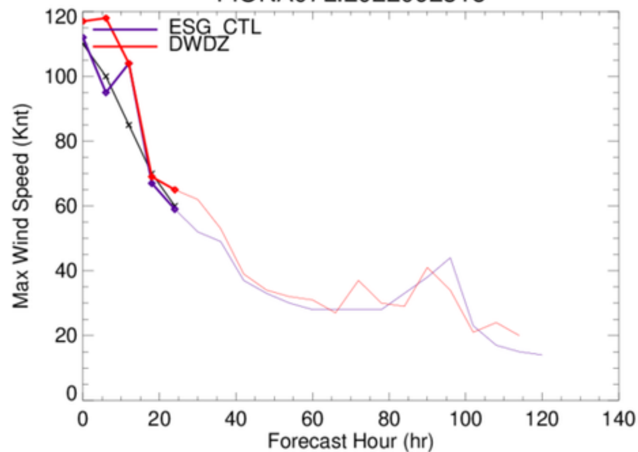
FIONA07L.2022092318
