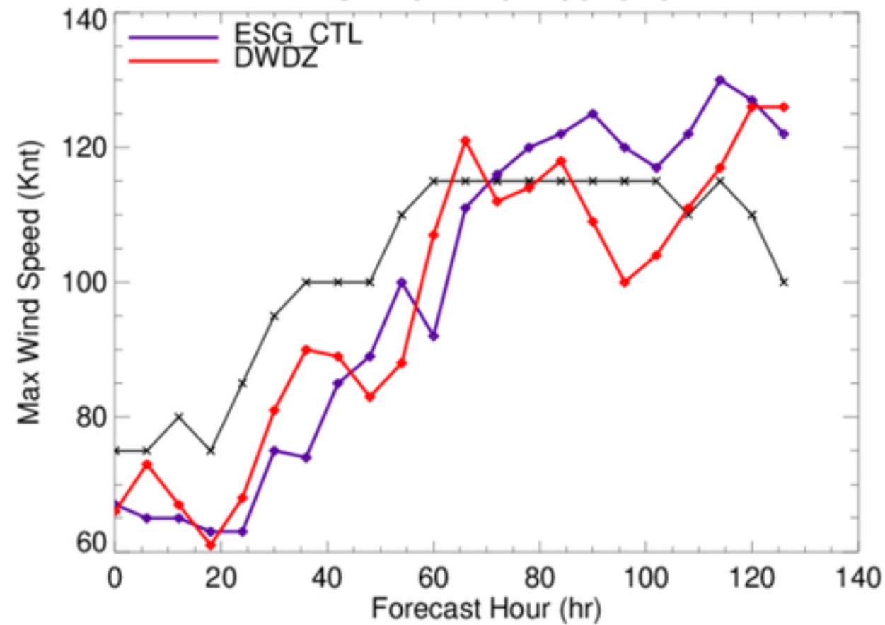
FIONA07L.2022091818
