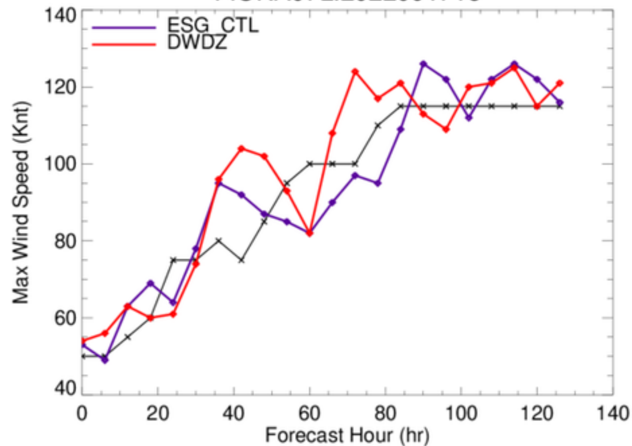
FIONA07L.2022091718
