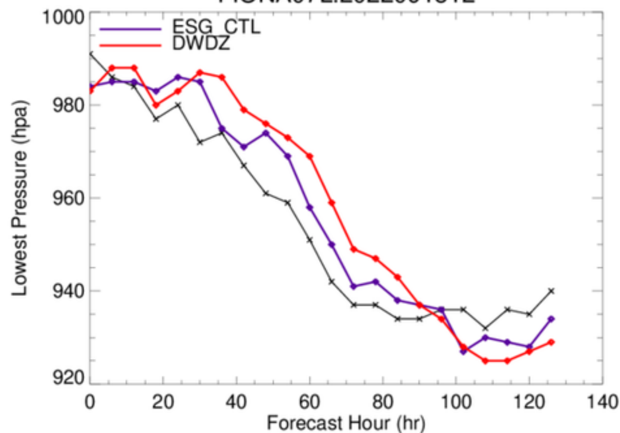
FIONA07L.2022091812
