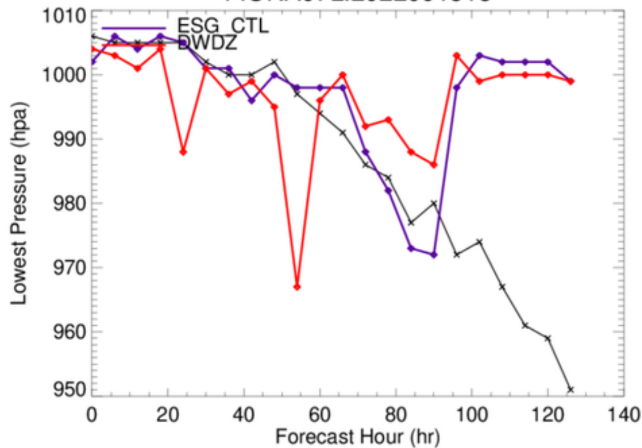
FIONA07L.2022091518
