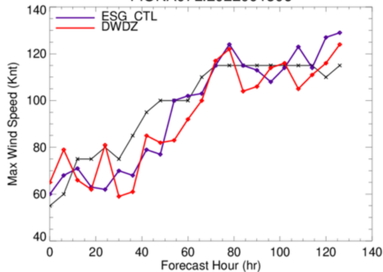
FIONA07L.2022091806
