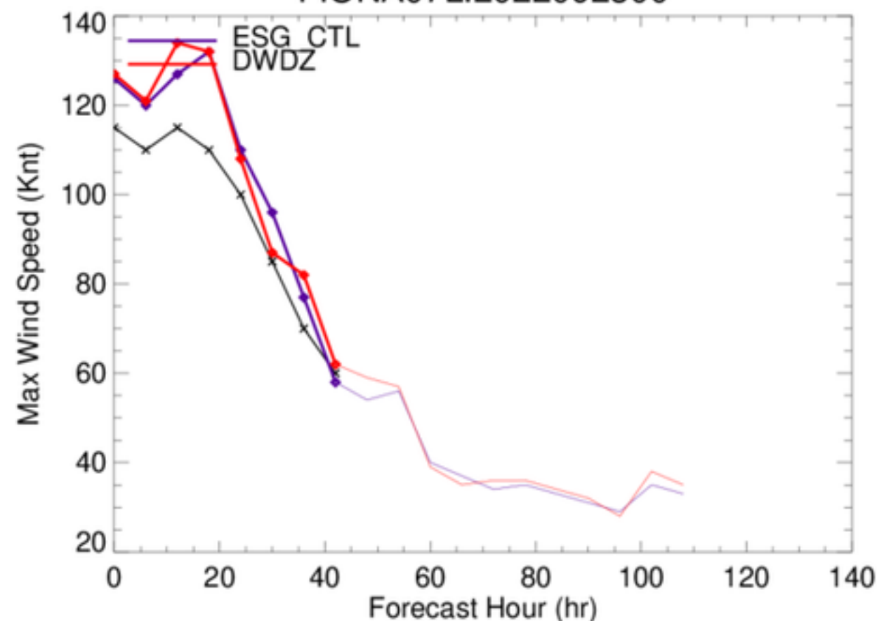
FIONA07L.2022092300
