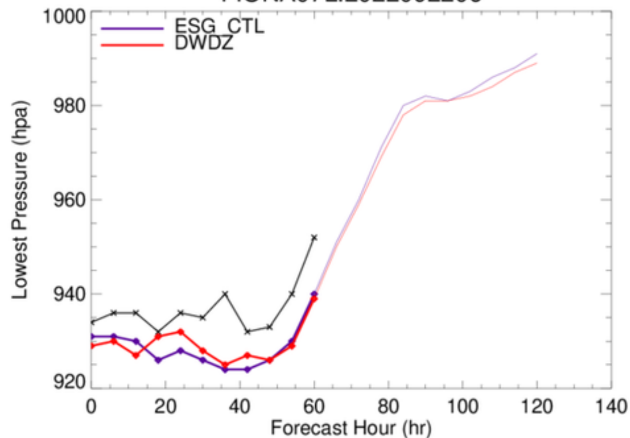
FIONA07L.2022092206
