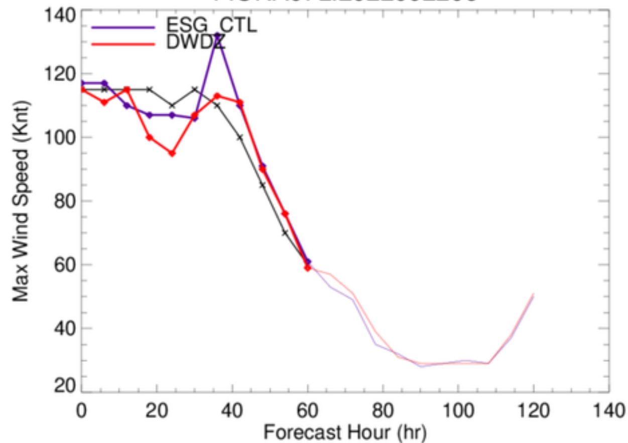
FIONA07L.2022092206
