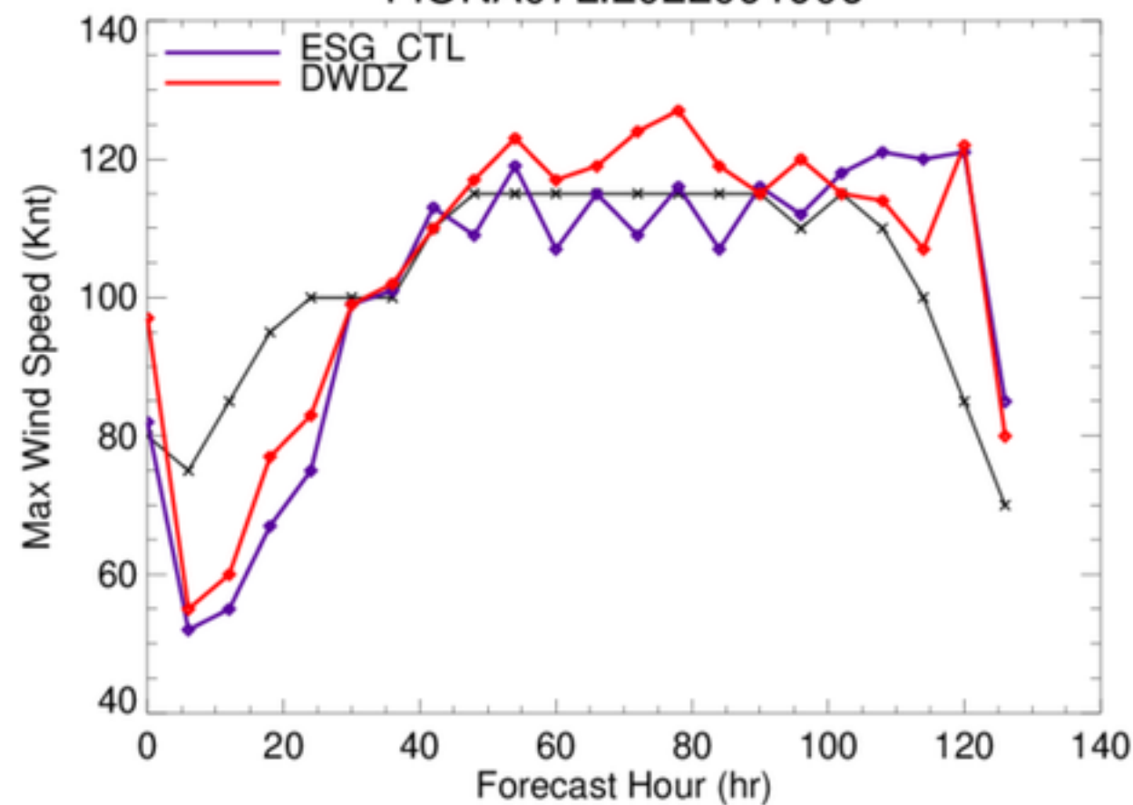
FIONA07L.2022091906
