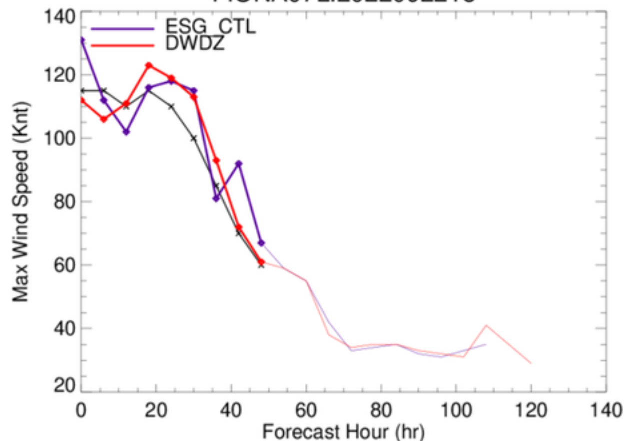
FIONA07L.2022092218
