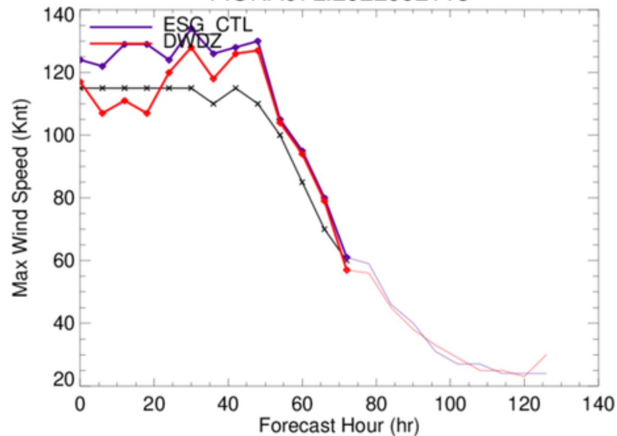
FIONA07L.2022092118
