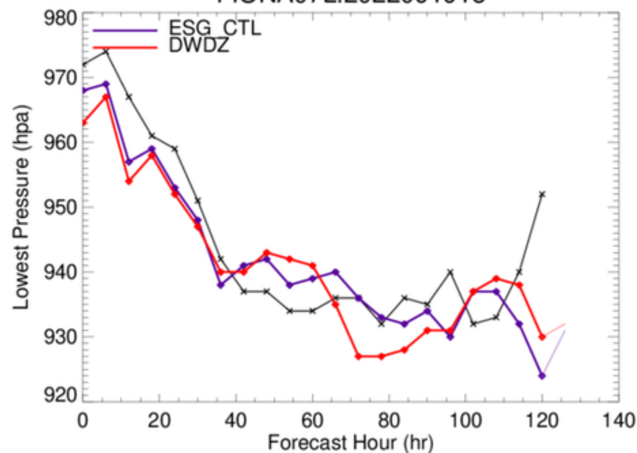
FIONA07L.2022091918
