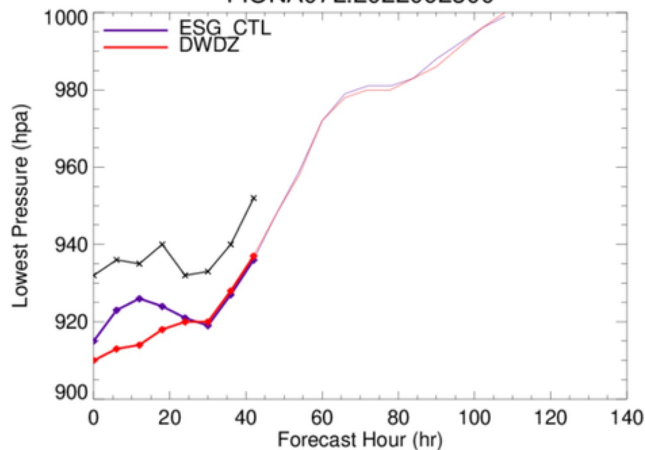
FIONA07L.2022092300
