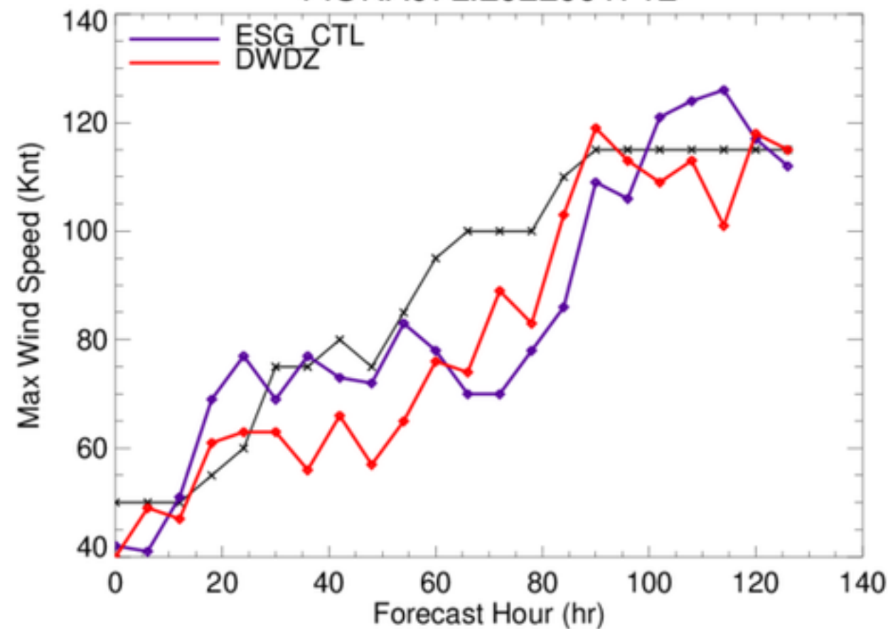
FIONA07L.2022091712
