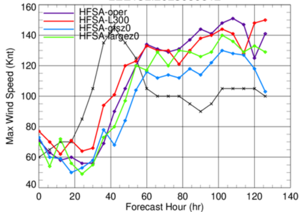
LEE13L.2023090612
