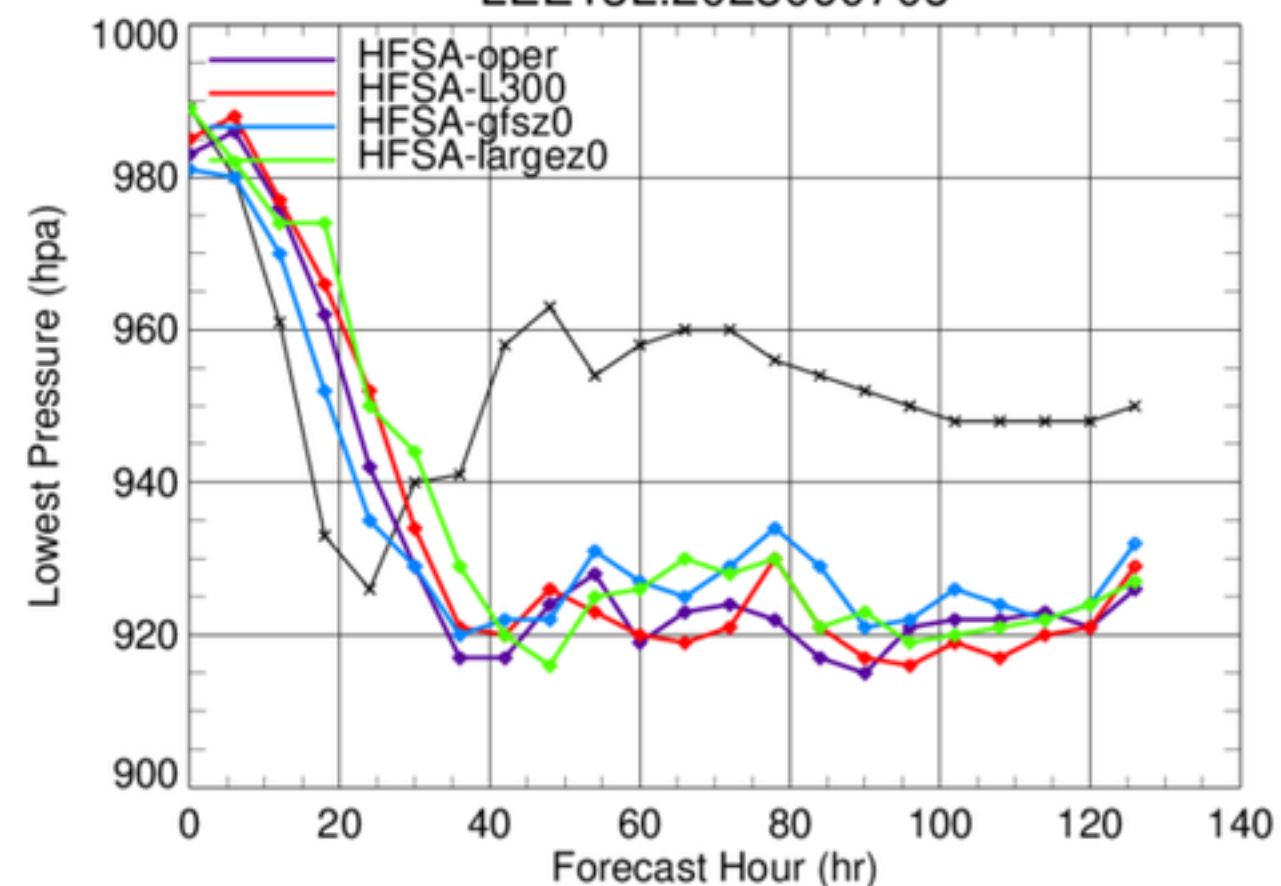
LEE13L.2023090706
