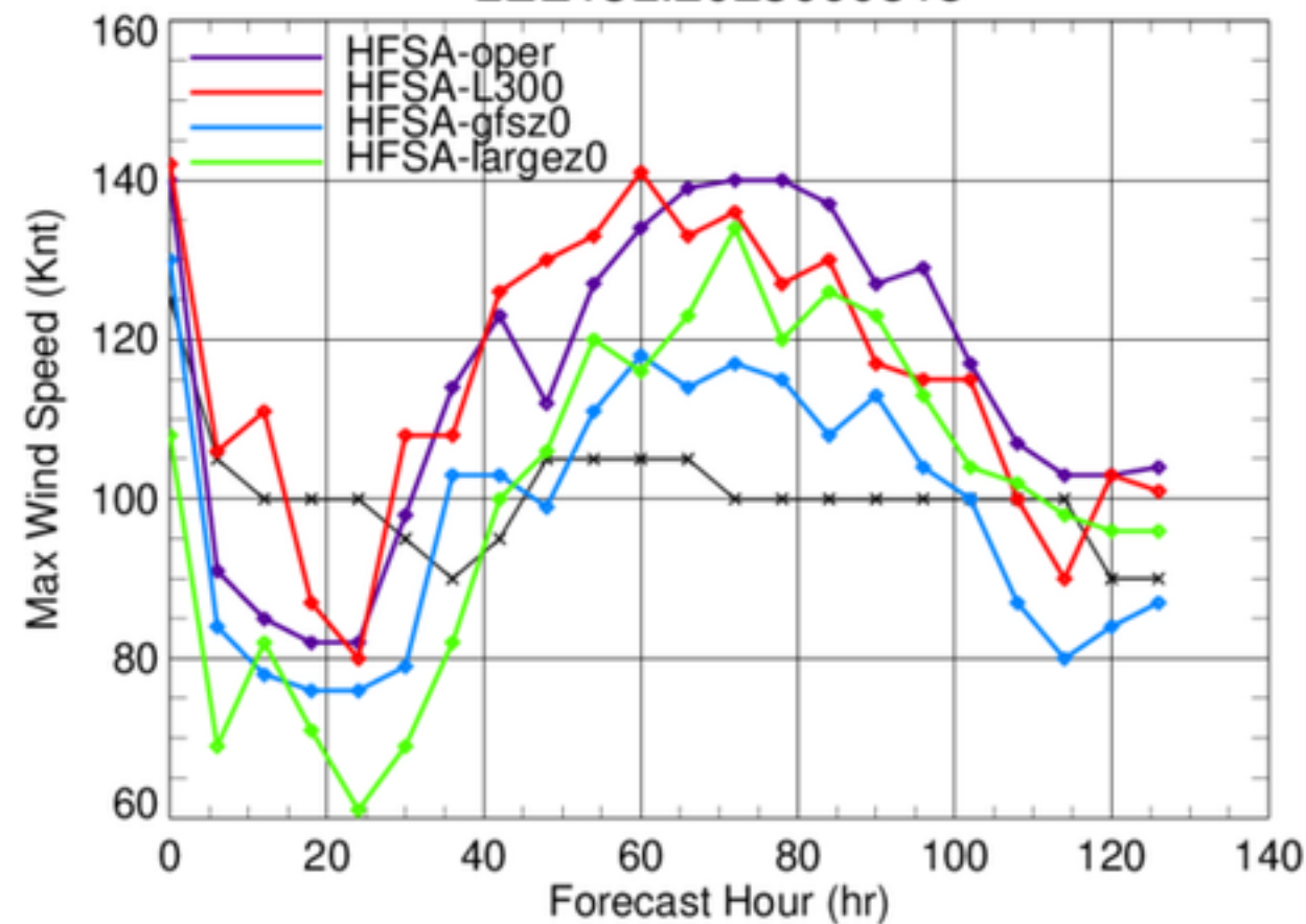
LEE13L.2023090818
