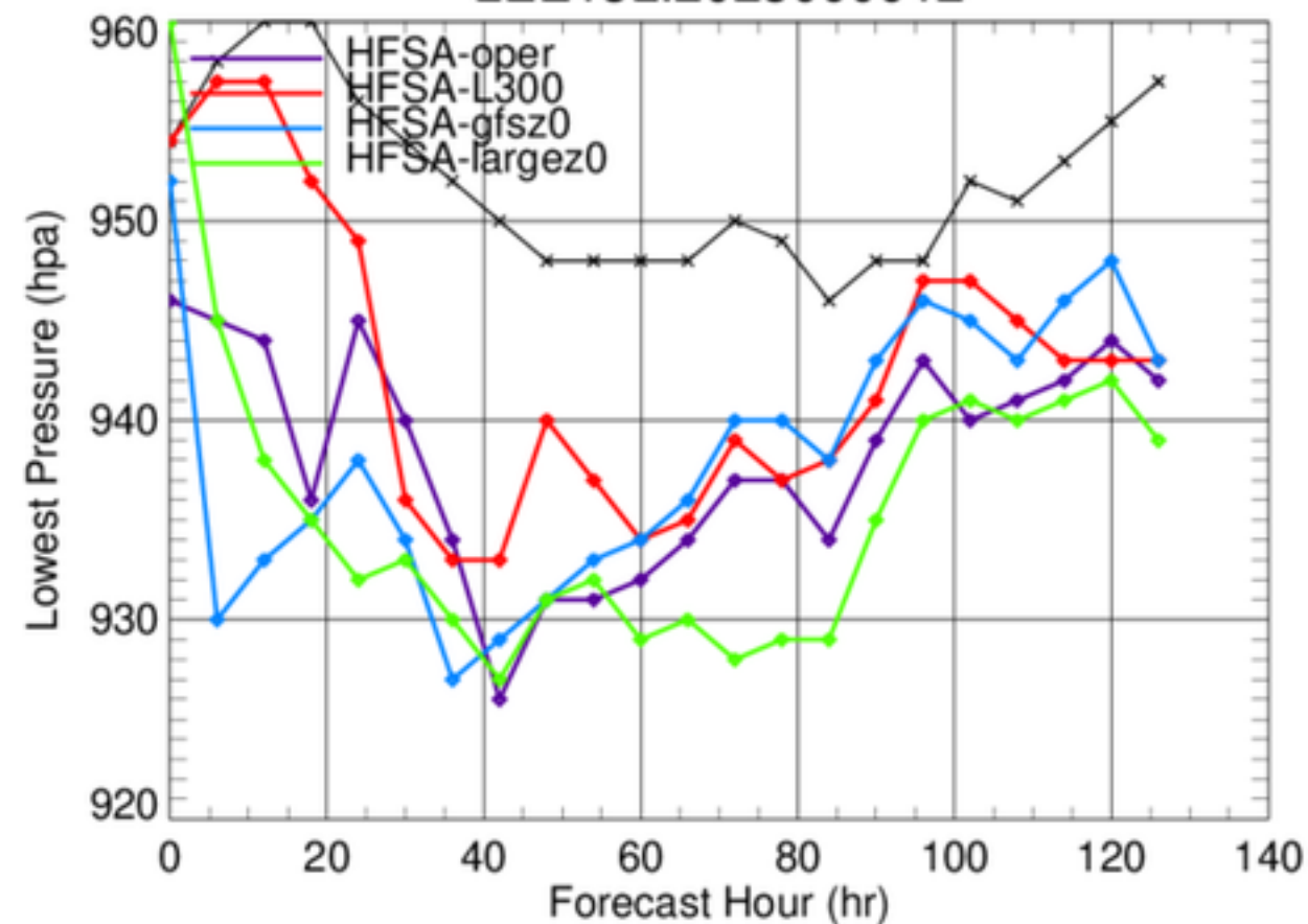
LEE13L.2023090912
