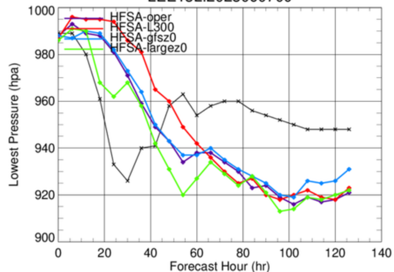
LEE13L.2023090700
