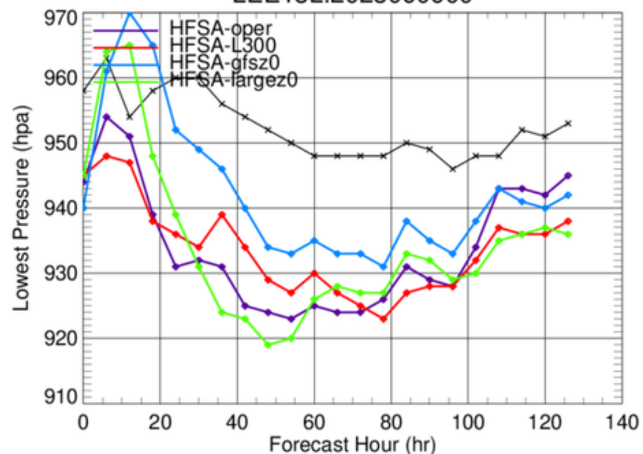
LEE13L.2023090900
