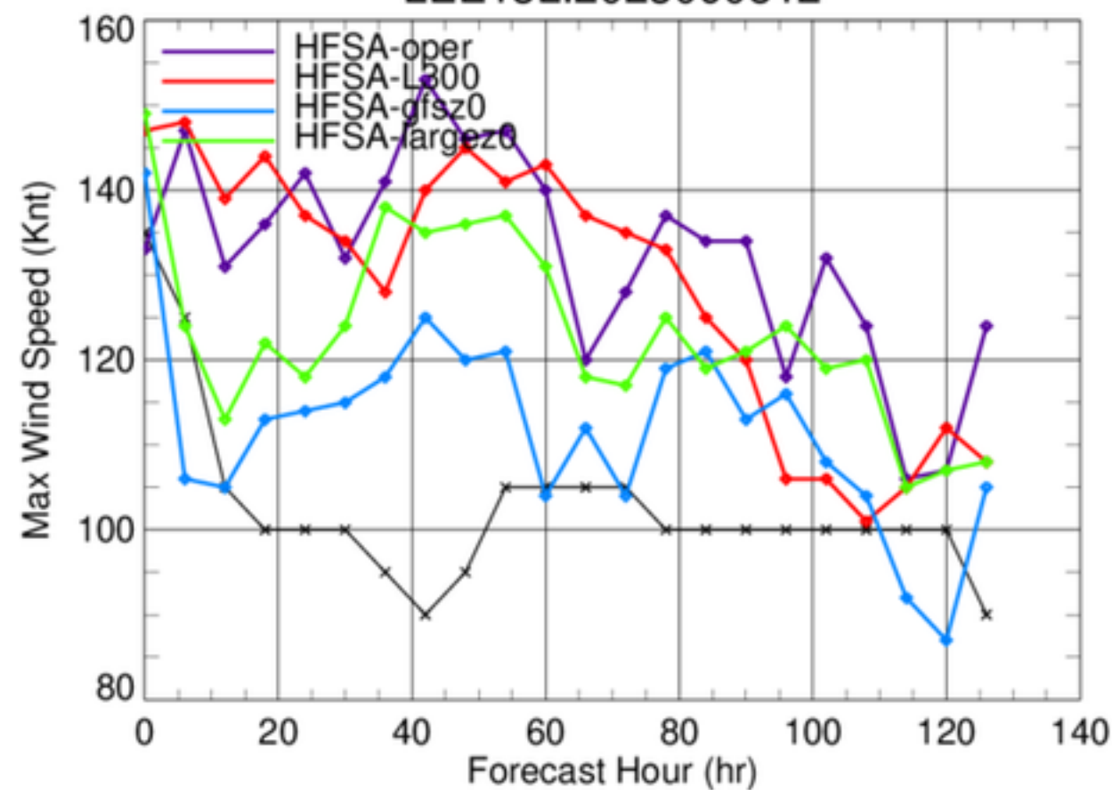
LEE13L.2023090812
