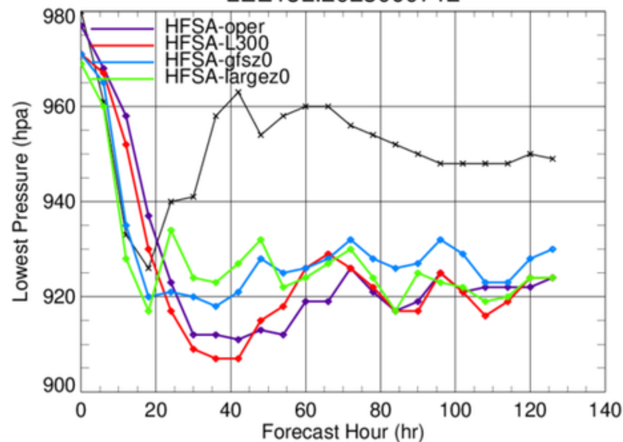
LEE13L.2023090712
