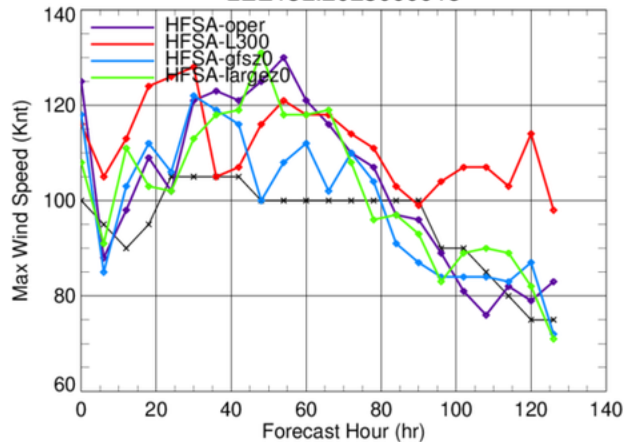
LEE13L.2023090918
