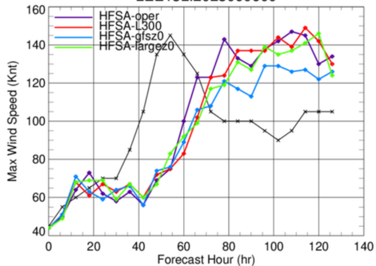
LEE13L.2023090600
