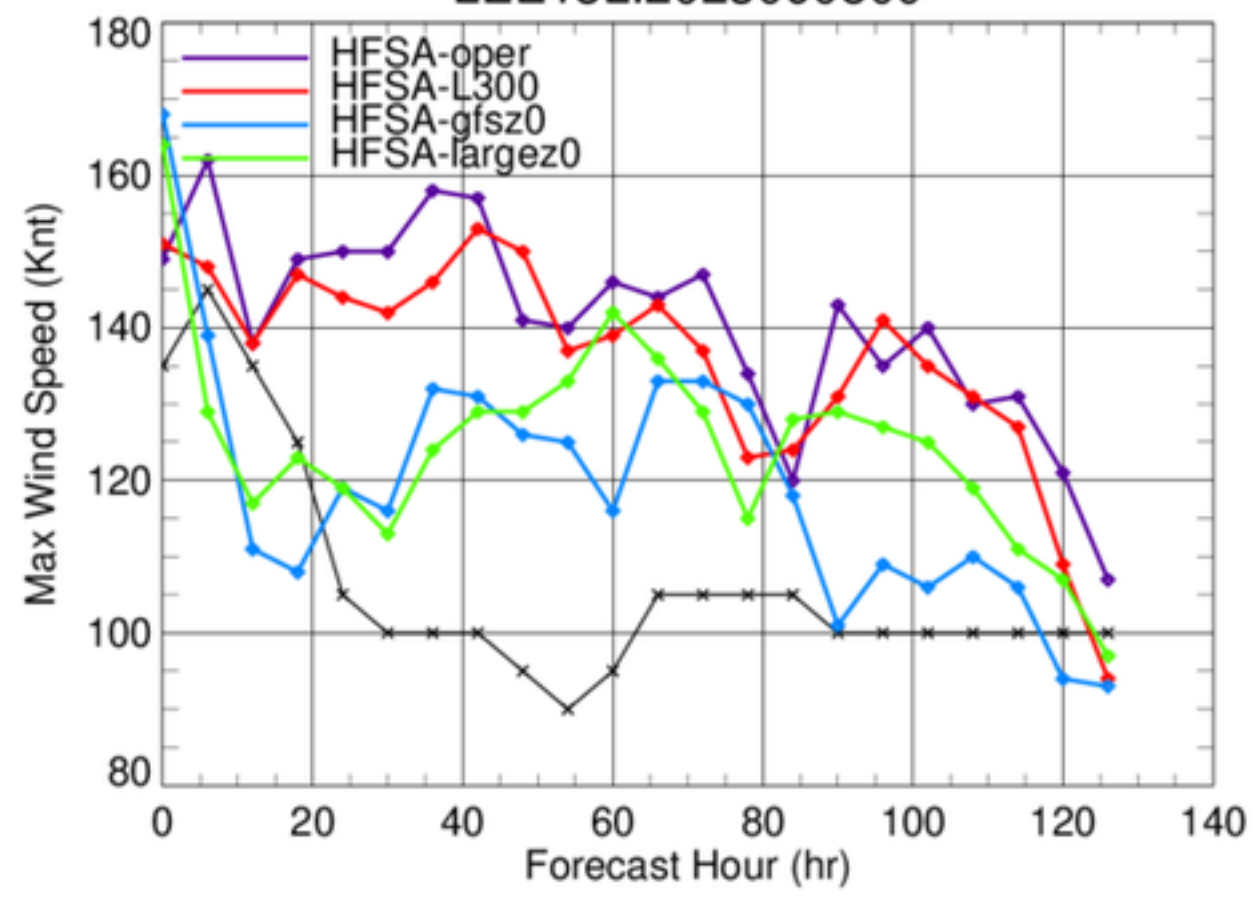
LEE13L.2023090800
