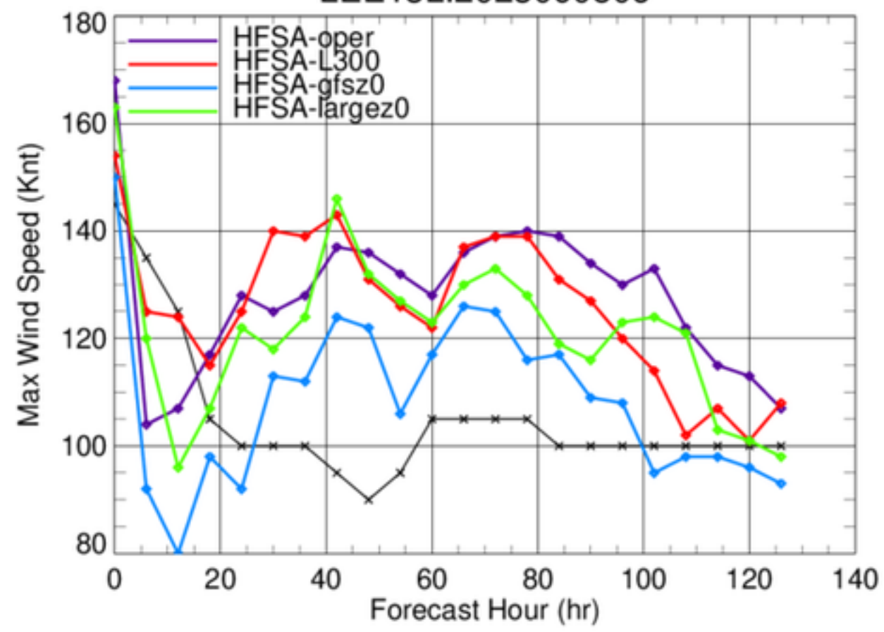
LEE13L.2023090806
