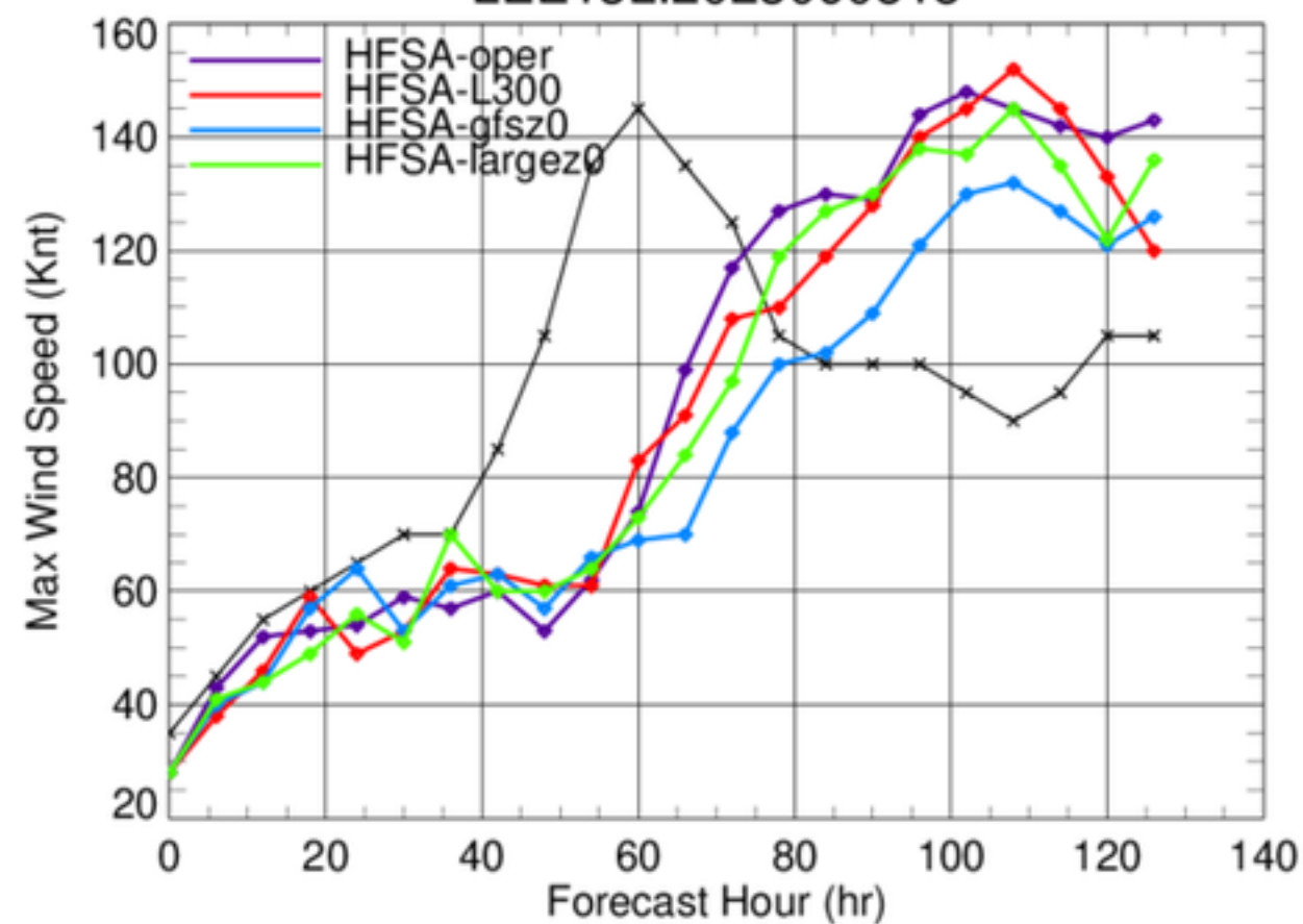
LEE13L.2023090518
