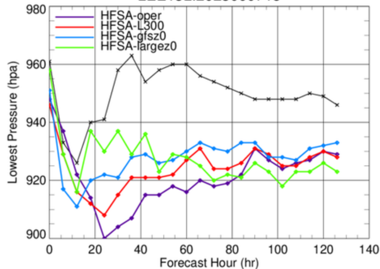
LEE13L.2023090718
