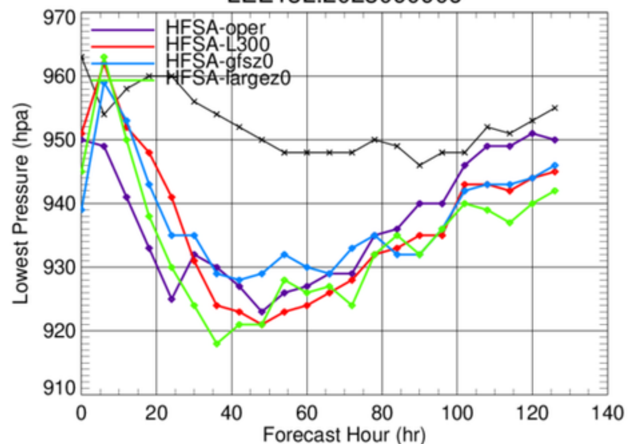
LEE13L.2023090906
