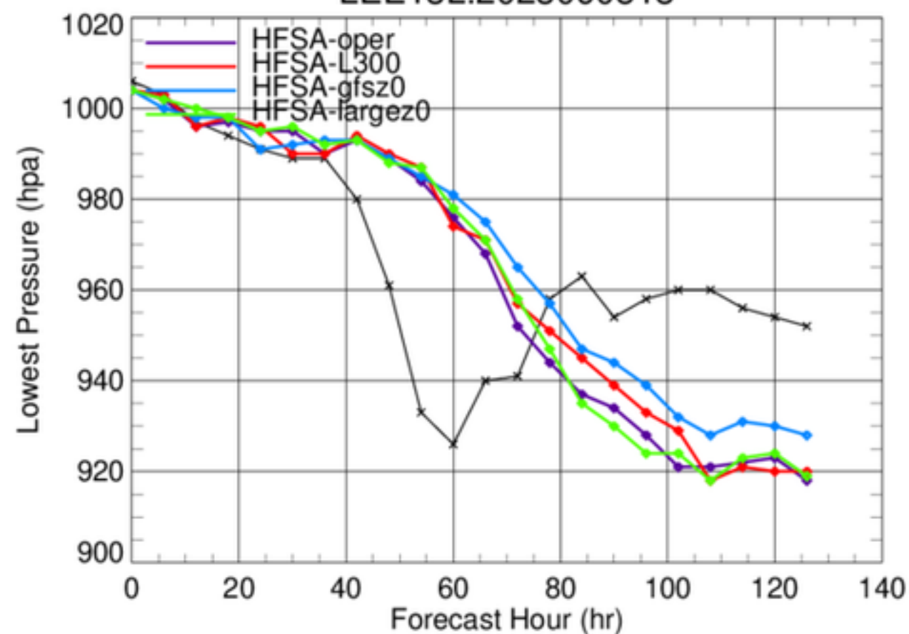
LEE13L.2023090518
