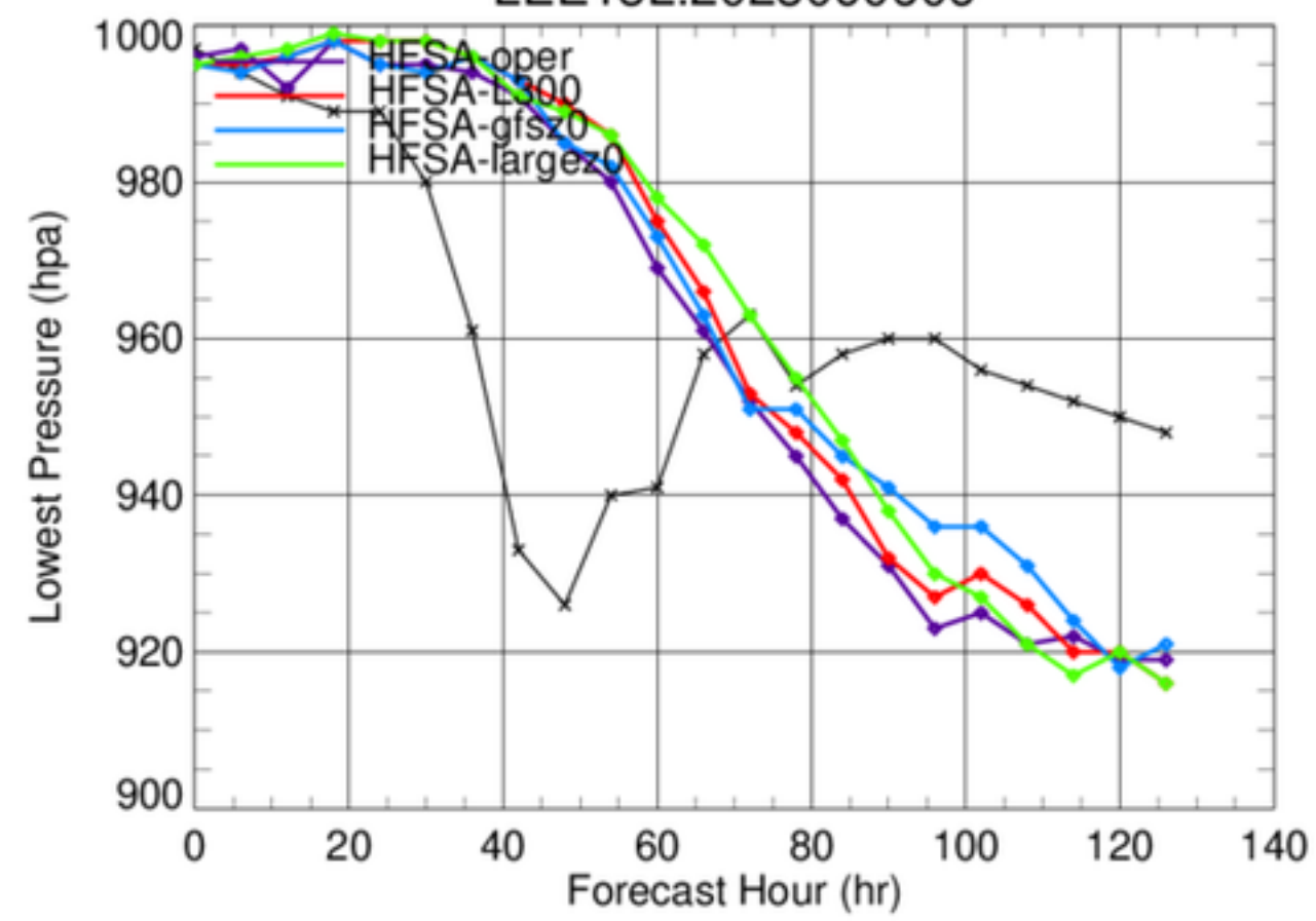
LEE13L.2023090606
