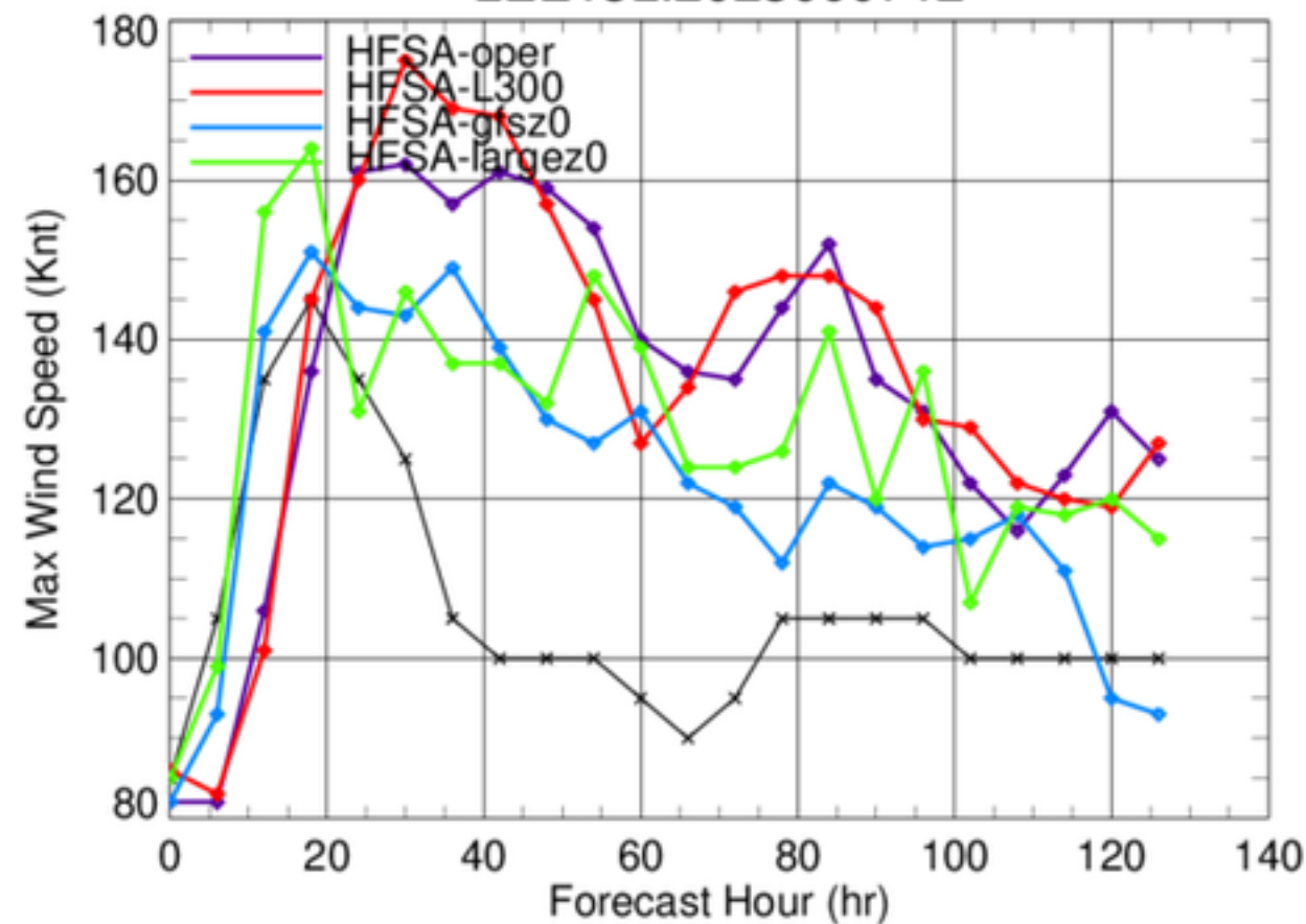
LEE13L.2023090712
