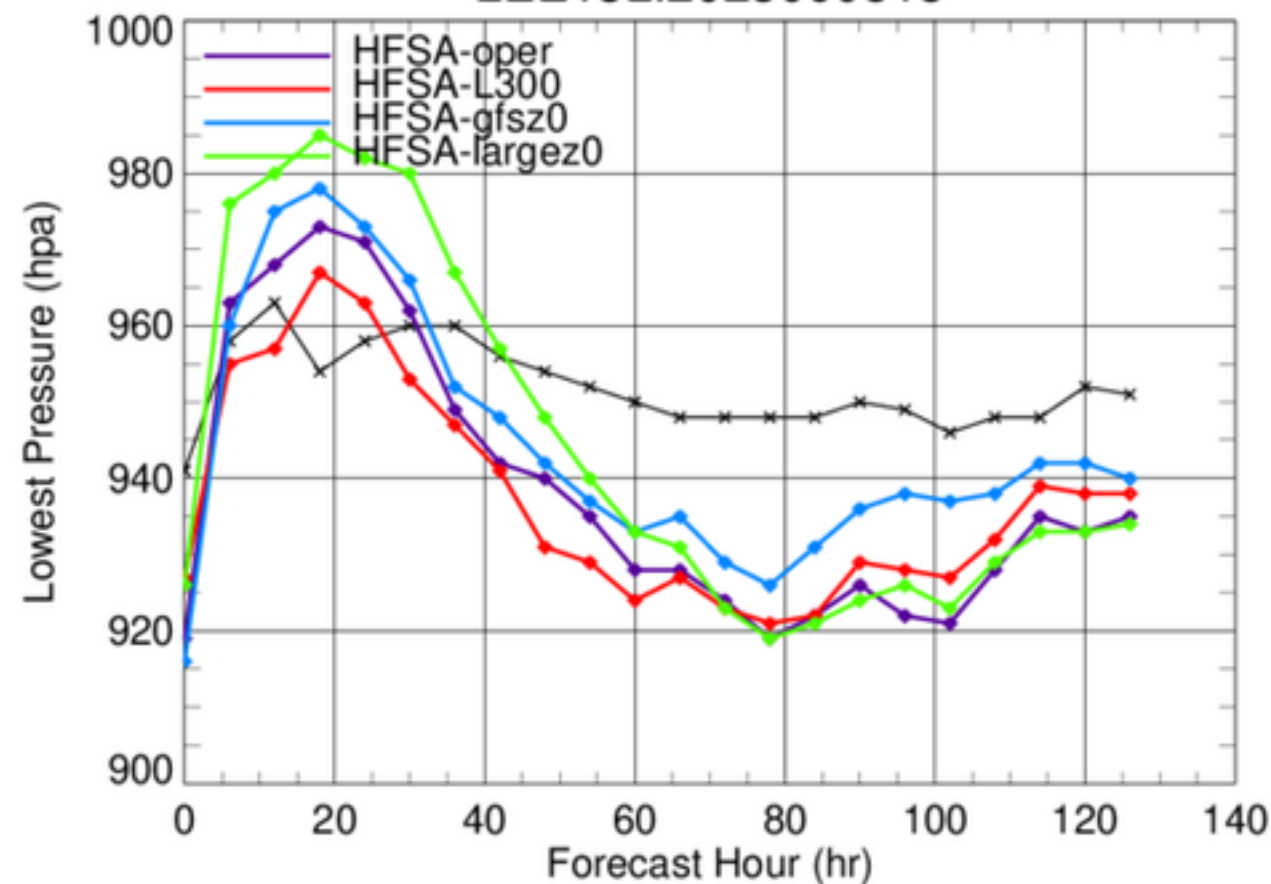
LEE13L.2023090818
