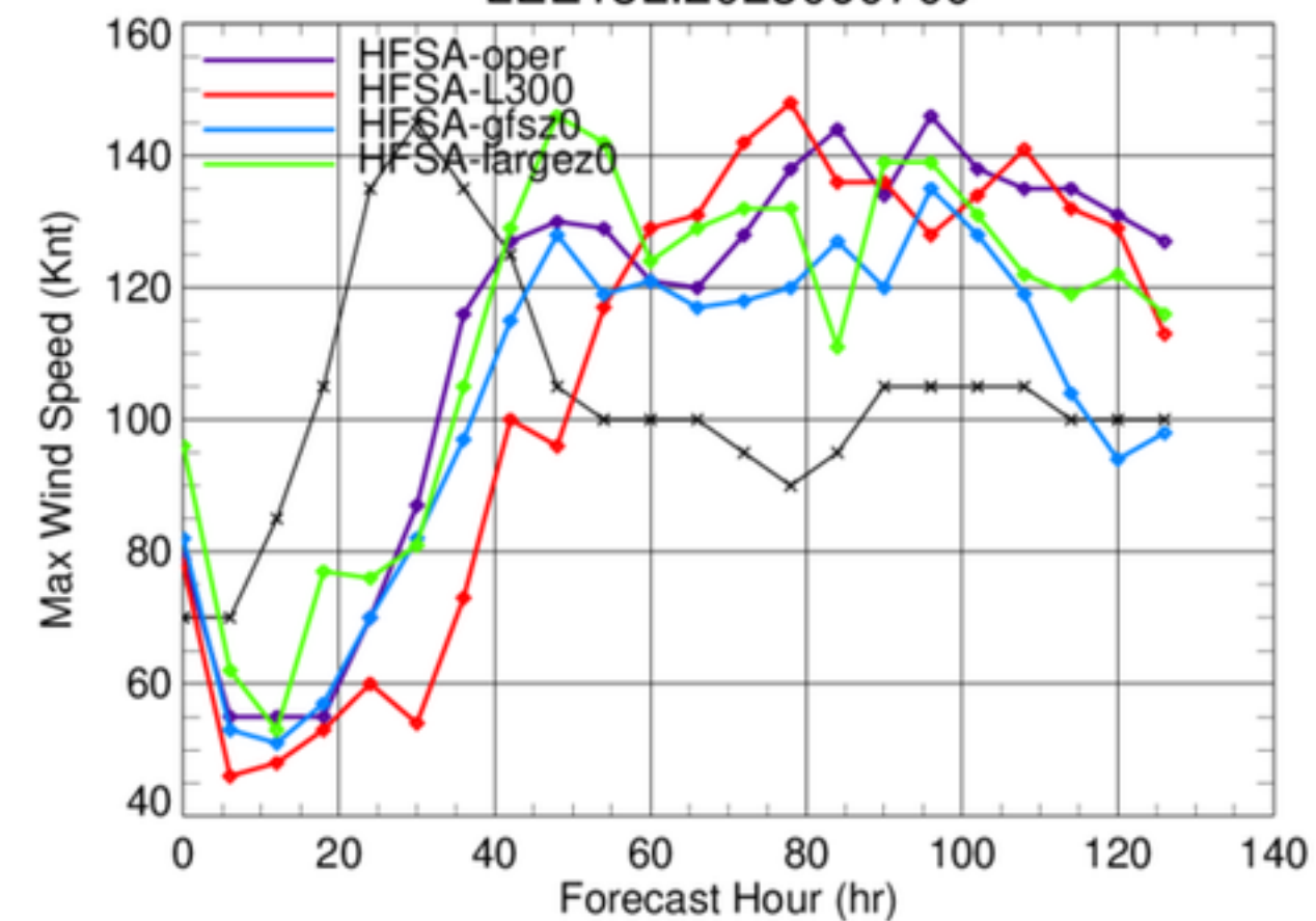
LEE13L.2023090700
