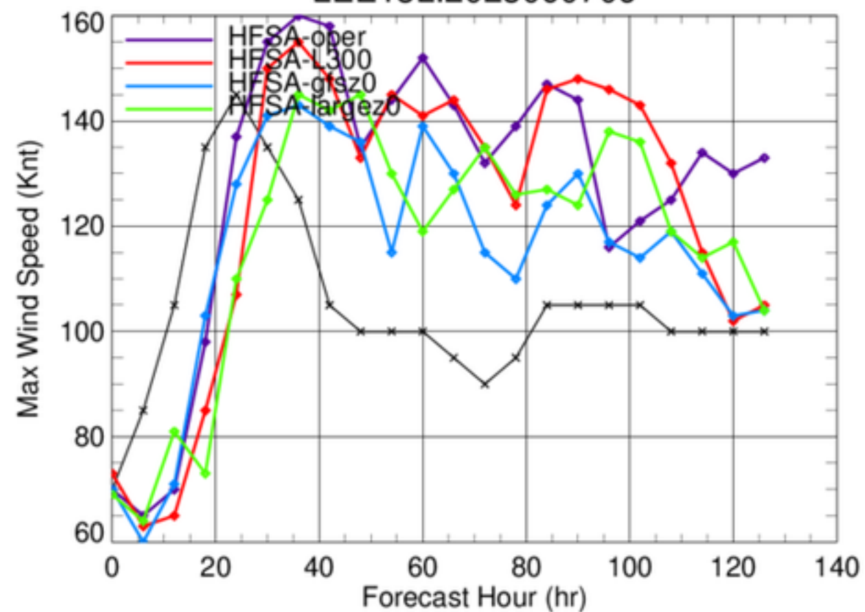
LEE13L.2023090706
