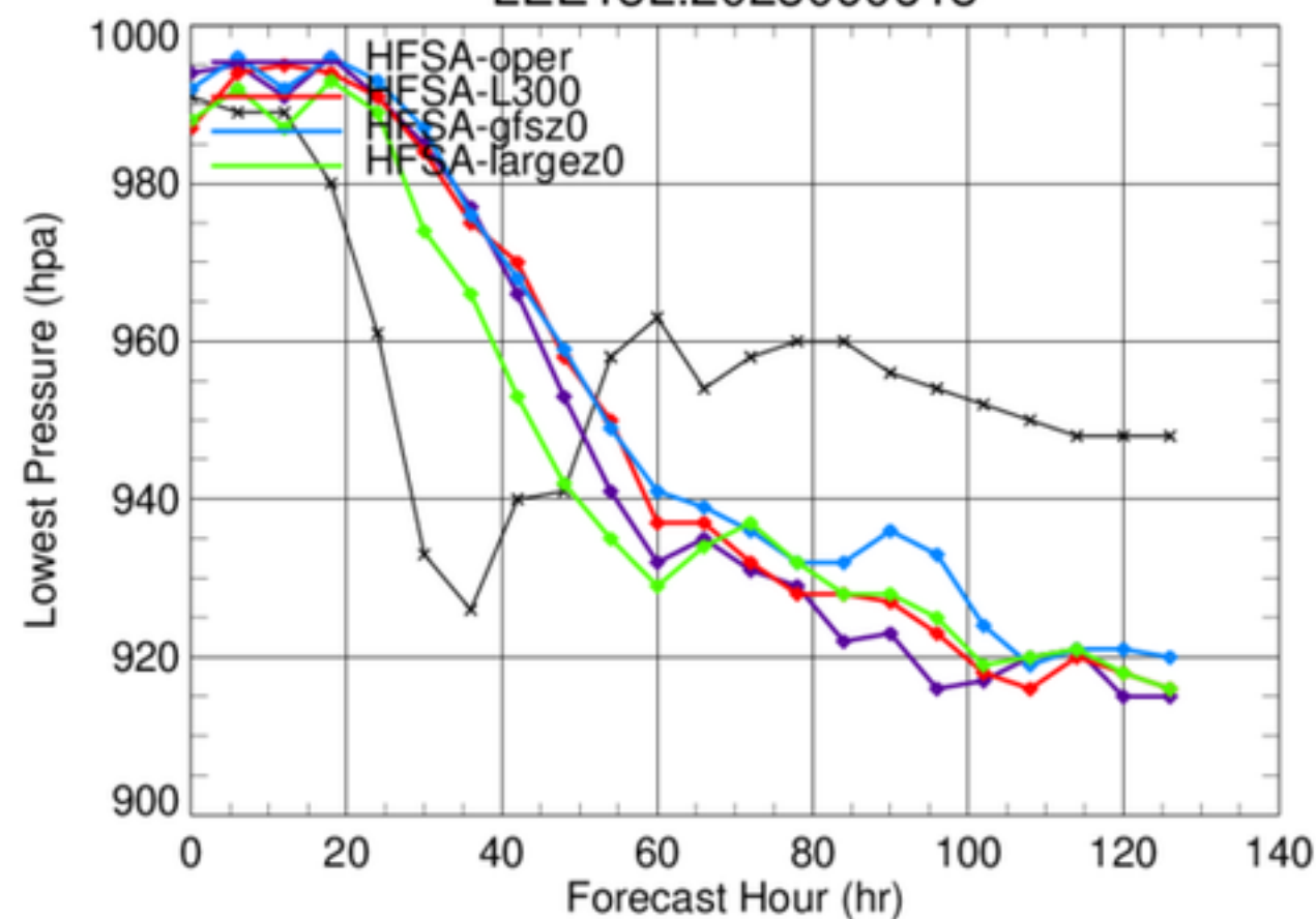
LEE13L.2023090618
