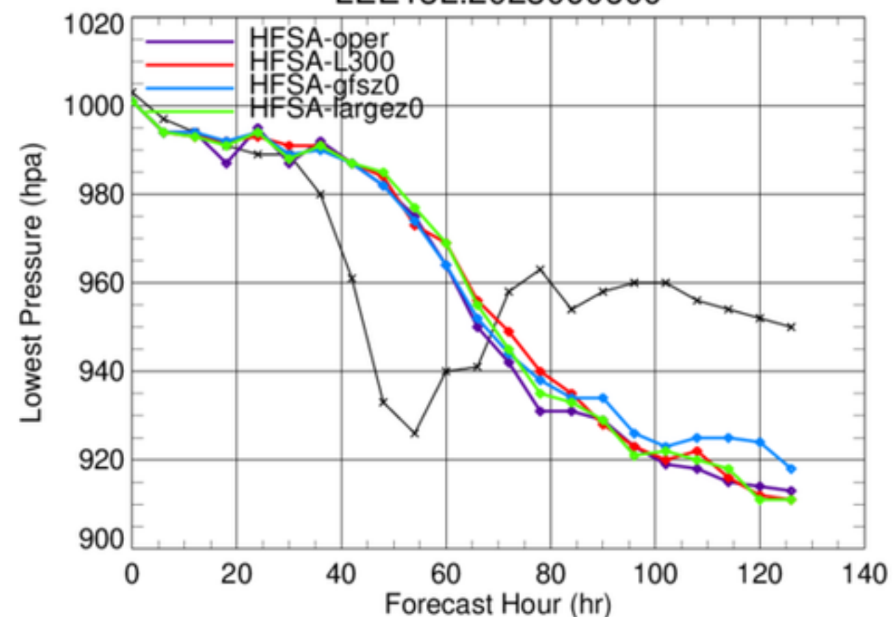
LEE13L.2023090600
