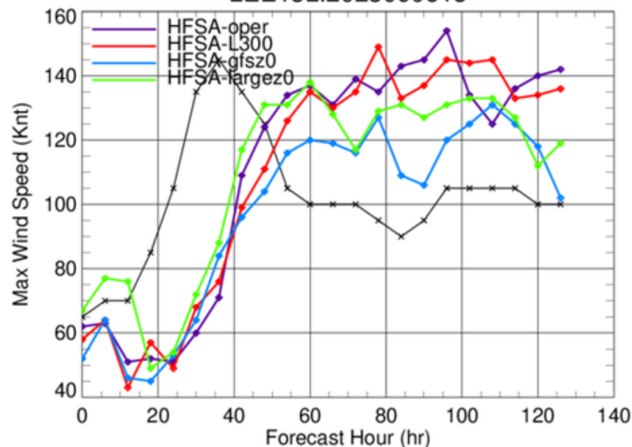
LEE13L.2023090618
