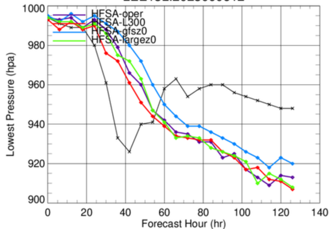
LEE13L.2023090612
