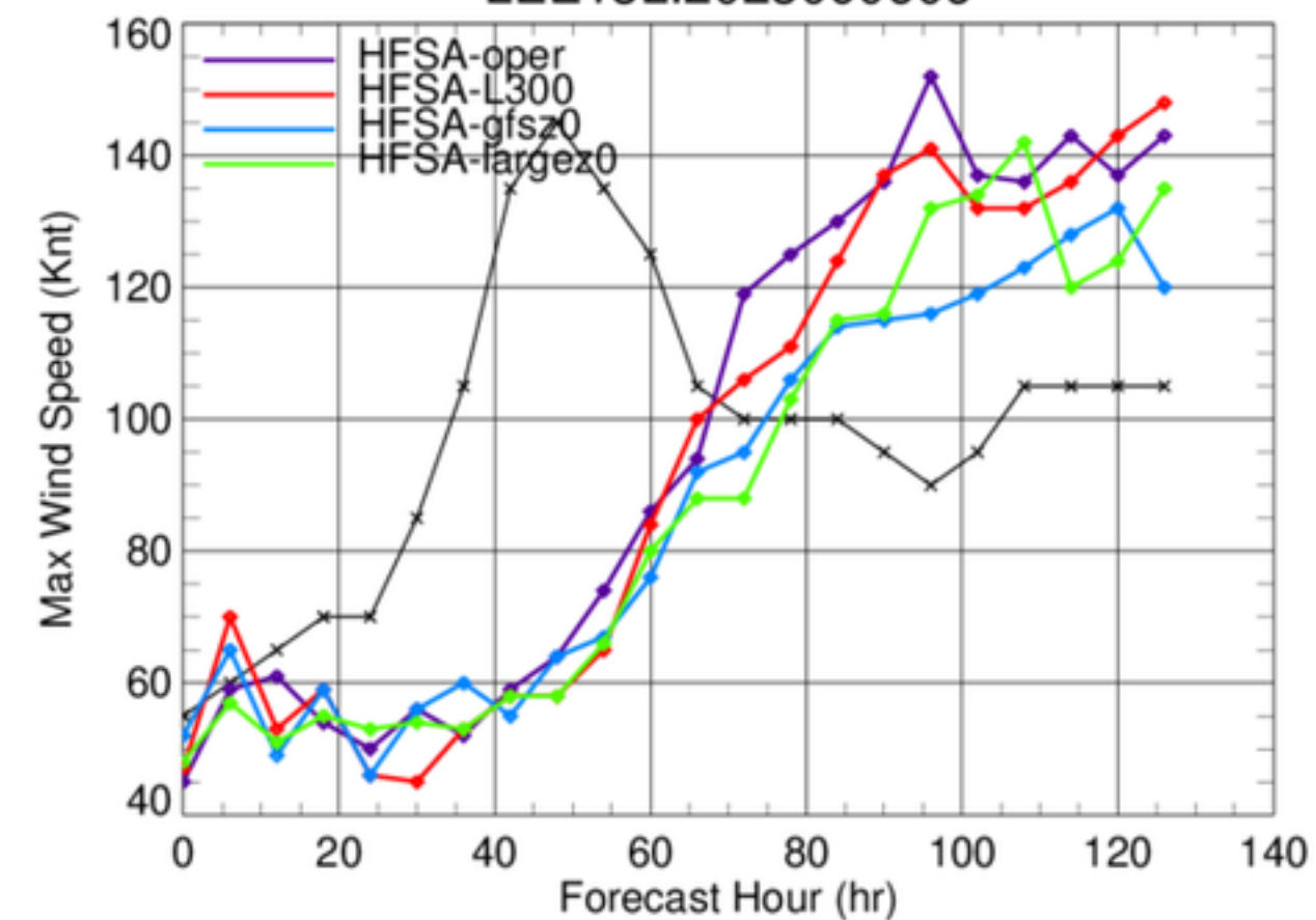
LEE13L.2023090606
